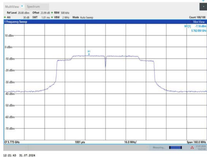
11AC80MIMO_Ant1_5775
