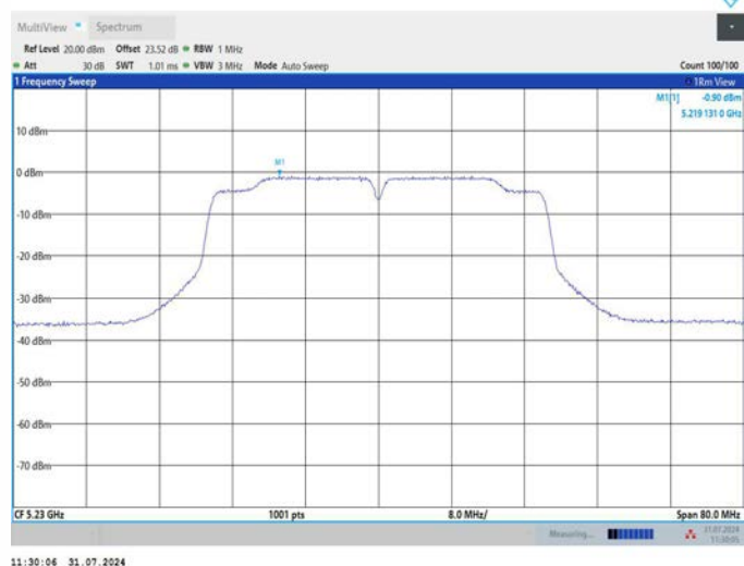
11AC40MIMO_Ant1_5230
