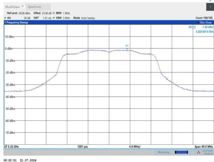
11N20MIMO_Ant2_5320
