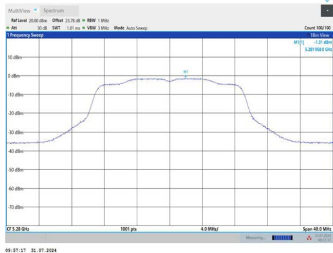
11AC20MIMO_Ant1_5280
