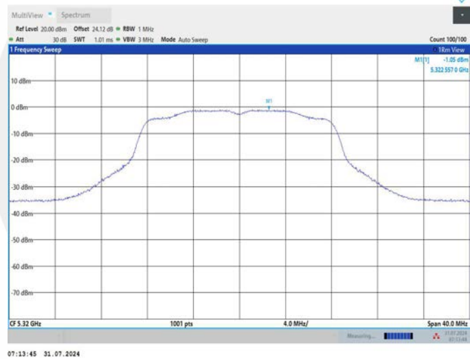
11A_Ant2_5320
