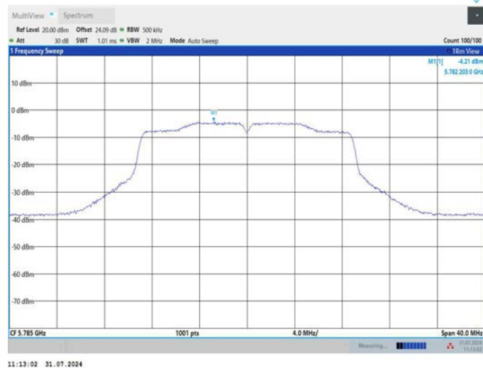
11AC20MIMO_Ant1_5785
