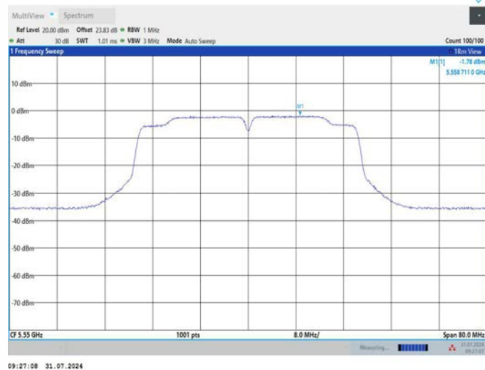
11N40MIMO_Ant2_5550
