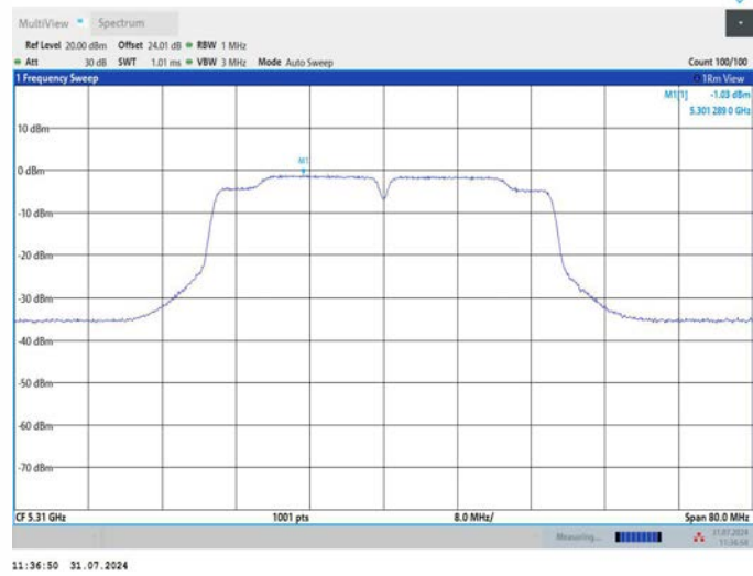
11AC40MIMO_Ant2_5310
