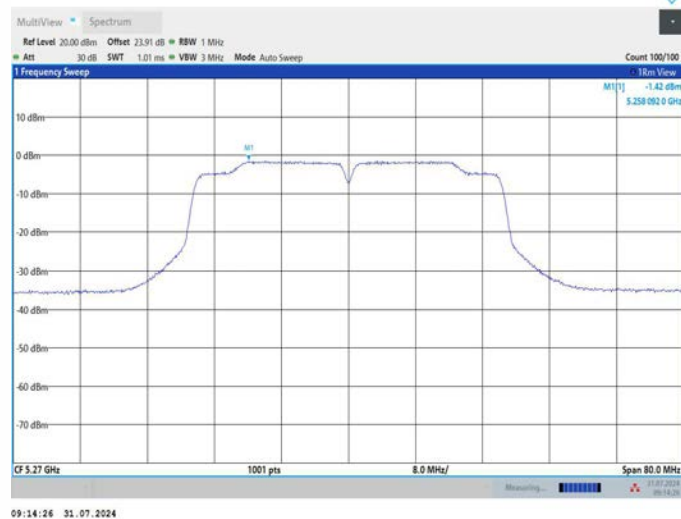
11N40MIMO_Ant2_5270
