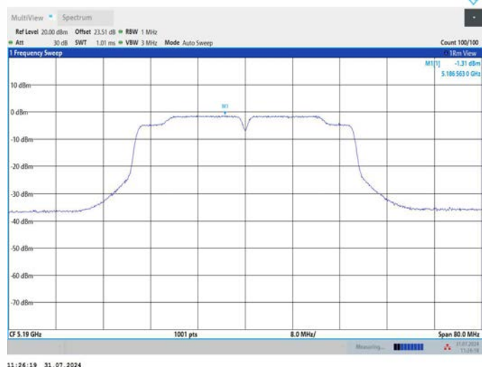
11AC40MIMO_Ant2_5190
