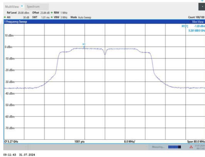
11N40MIMO_Ant2_5270
