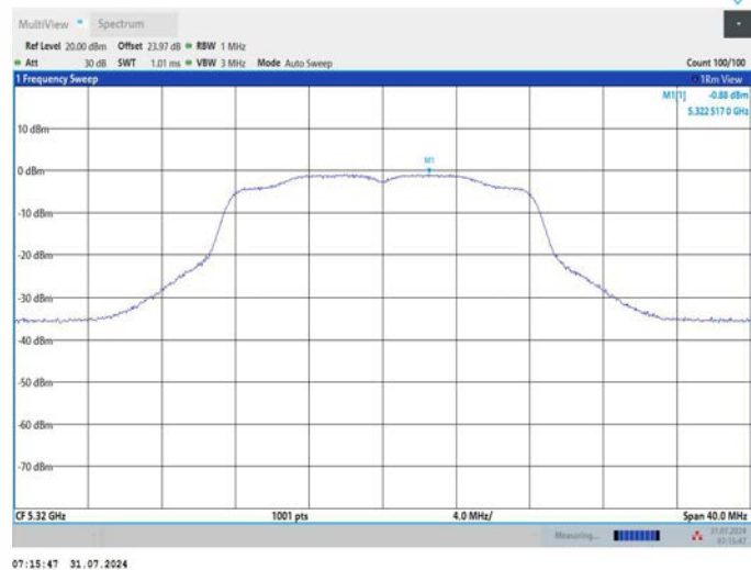
11A_Ant2_5320
