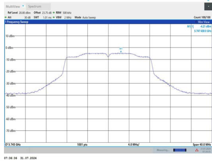
11A_Ant2_5745
