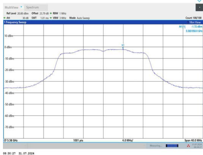
11N20MIMO_Ant1_5580
