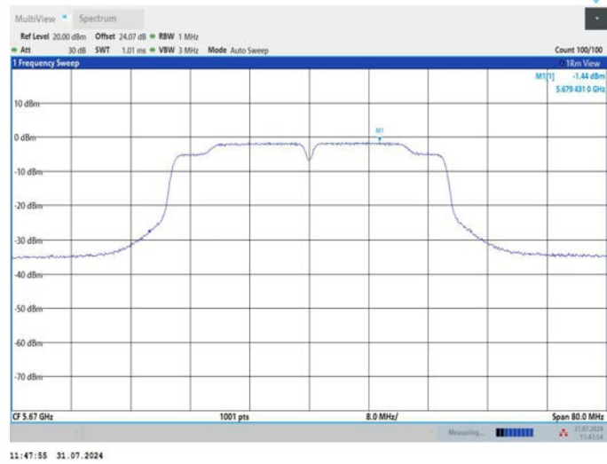
11AC40MIMO_Ant2_5670
