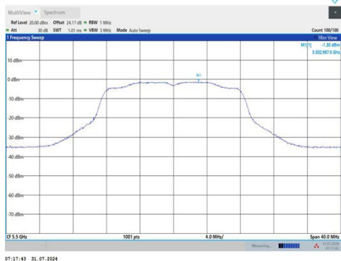
11A_Ant2_5500
