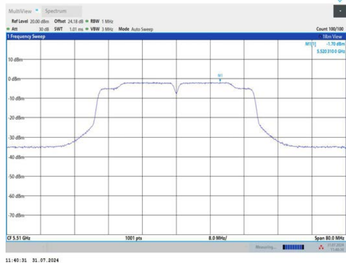
11AC40MIMO_Ant1_5510
