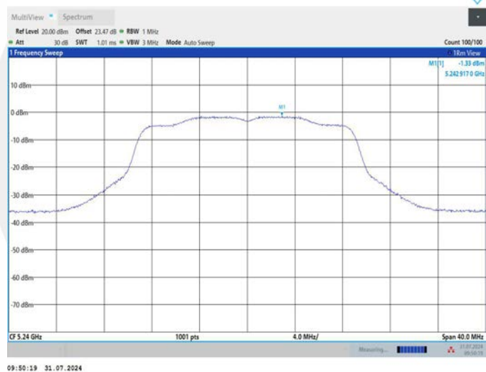
11AC20MIMO_Ant2_5240
