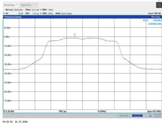
11AC20MIMO_Ant2_5260
