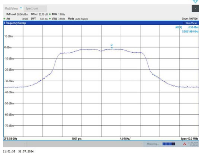
11AC20MIMO_Ant1_5580
