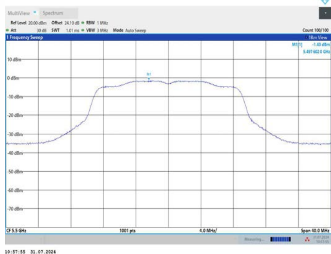
11AC20MIMO_Ant2_5500
