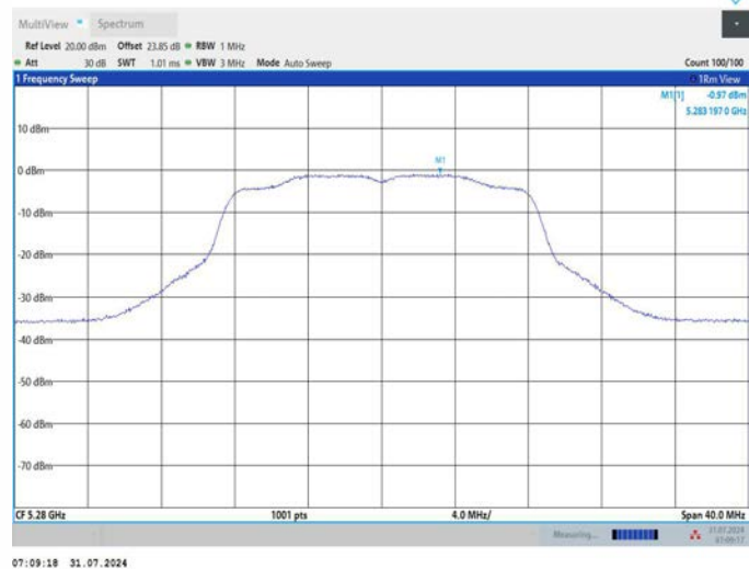
11A_Ant1_5280
