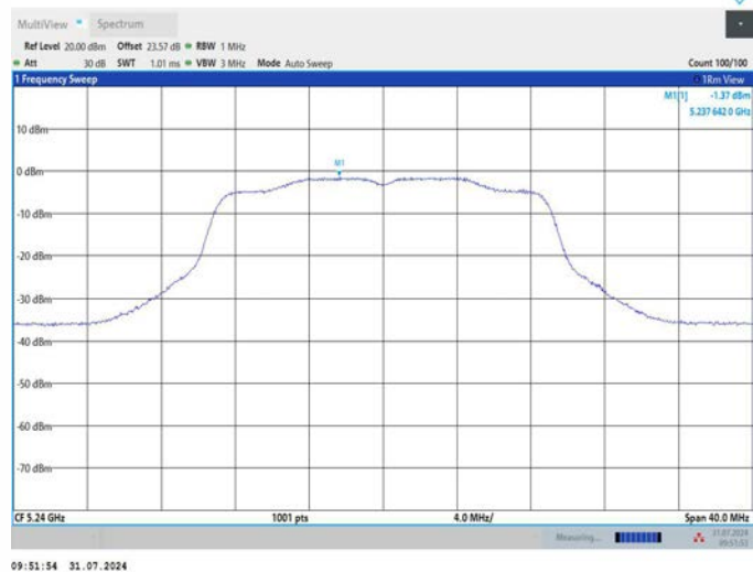
11AC20MIMO_Ant2_5240
