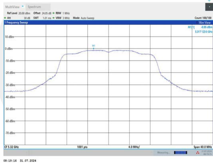
11N20MIMO_Ant2_5320
