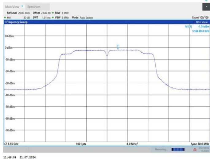
11AC40MIMO_Ant2_5550
