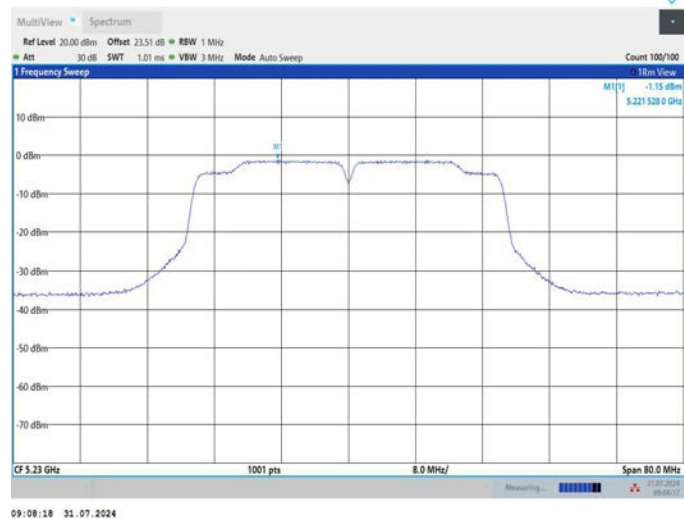
11N40MIMO_Ant1_5230
