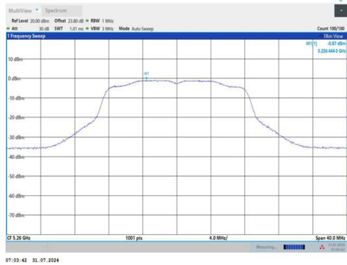
11A_Ant2_5260
