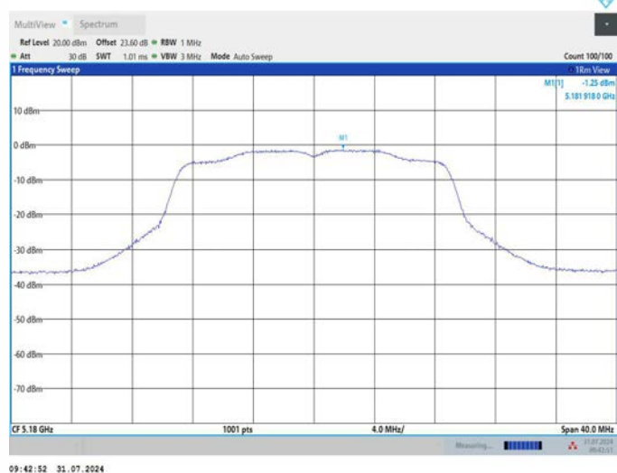
11AC20MIMO_Ant2_5180
