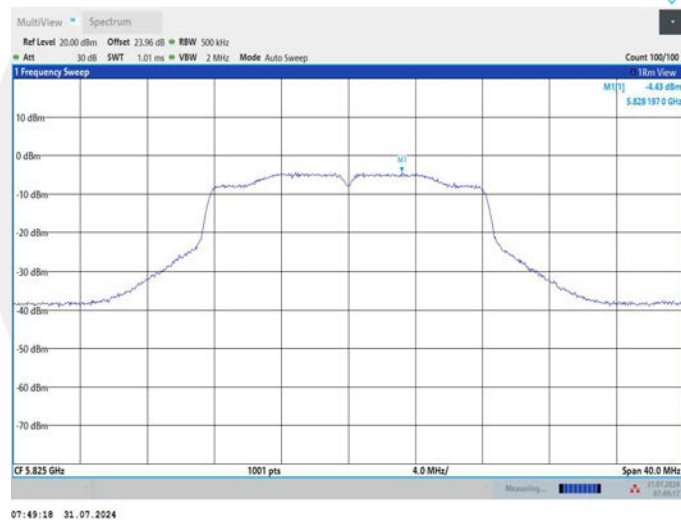
11A_Ant2_5825
