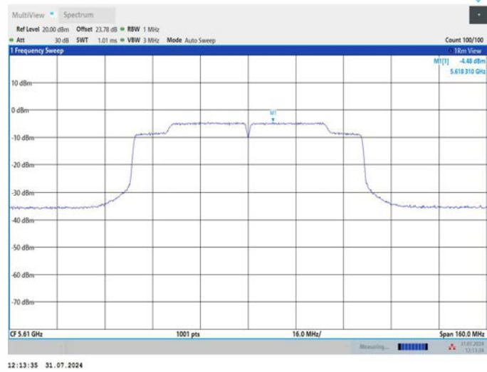
11AC80MIMO_Ant2_5610
