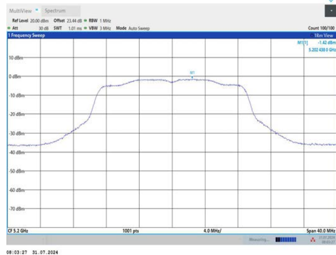
11N20MIMO_Ant1_5200
