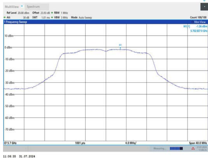
11AC20MIMO_Ant2_5700
