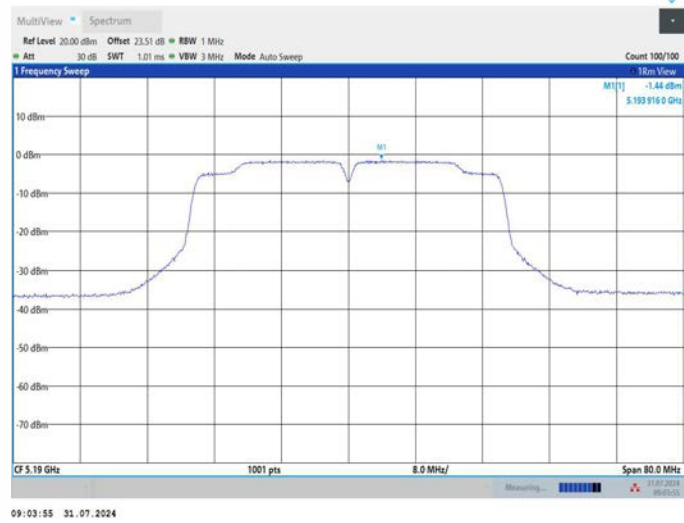
11N40MIMO_Ant2_5190
