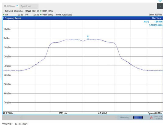
11A_Ant2_5700
