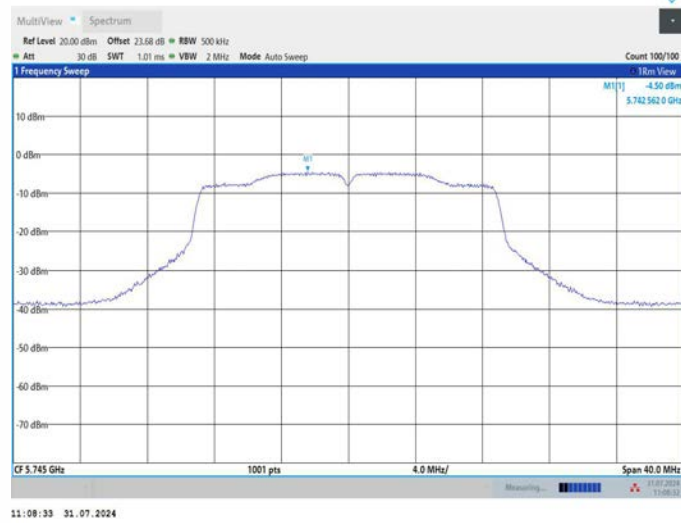
11AC20MIMO_Ant2_5745
