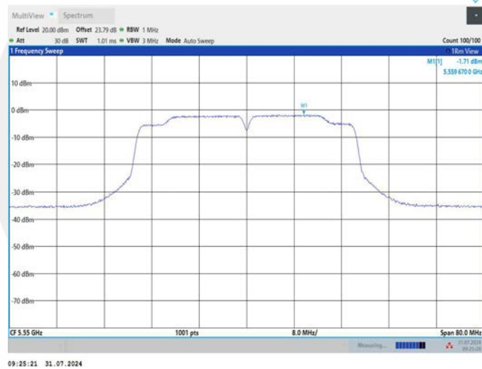
11N40MIMO_Ant2_5550
