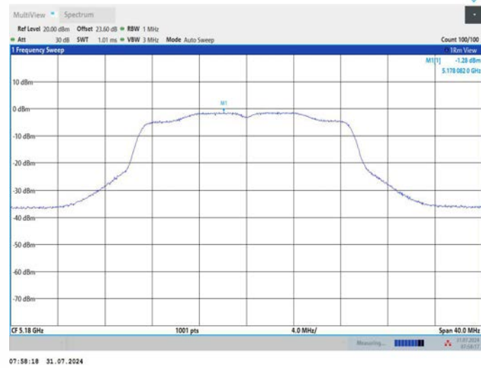
11N20MIMO_Ant2_5180
