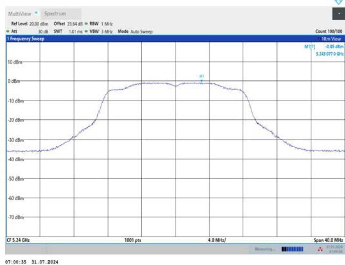
11A_Ant2_5240
