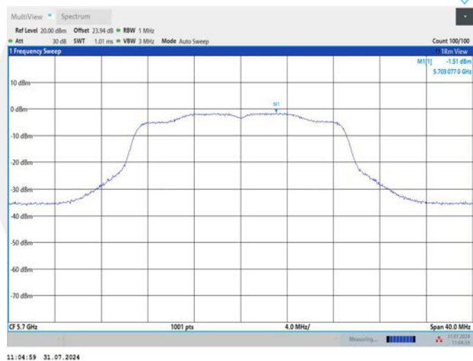
11AC20MIMO_Ant2_5700
