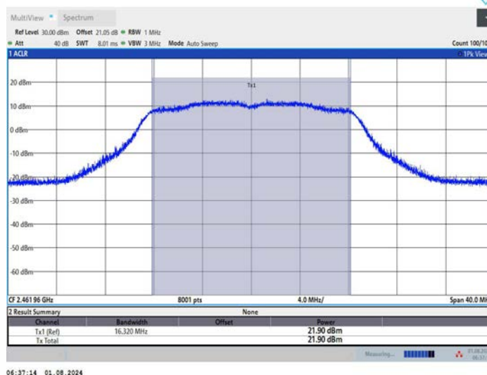
11N20MIMO_Ant2_2462
