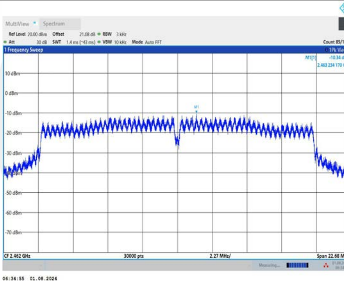
11N20MIMO_Ant2_2462
