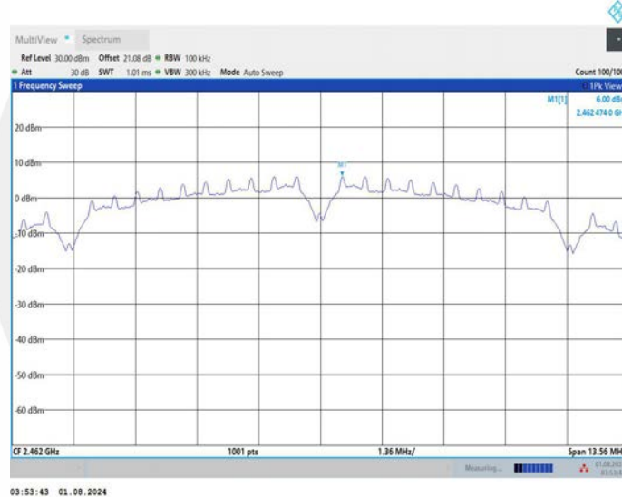
11B_Ant2_2462
