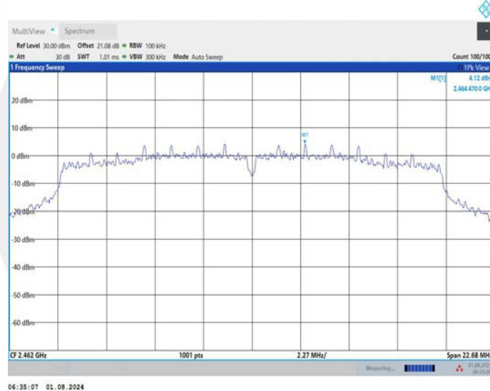
11N20MIMO_Ant2_2462
