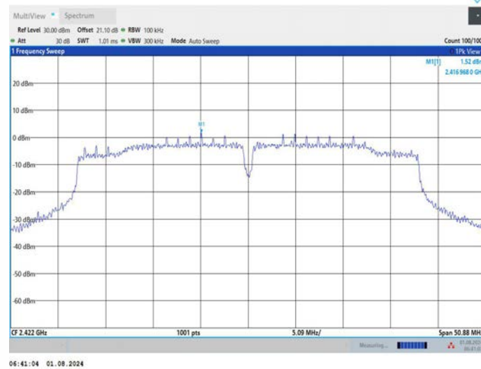
11N40MIMO_Ant2_2422
