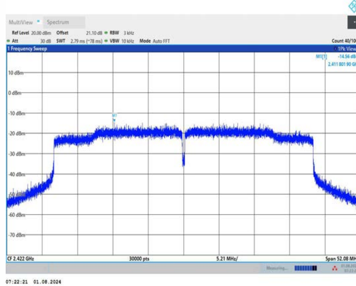
11AX40MIMO_Ant2_2422
