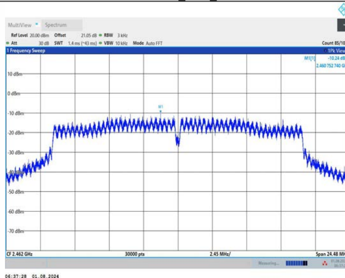
11N20MIMO_Ant2_2462
