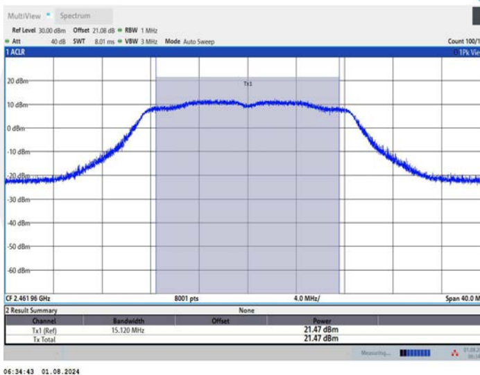
11N20MIMO_Ant2_2462
