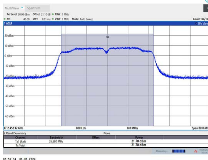
11N40MIMO_Ant2_2452
