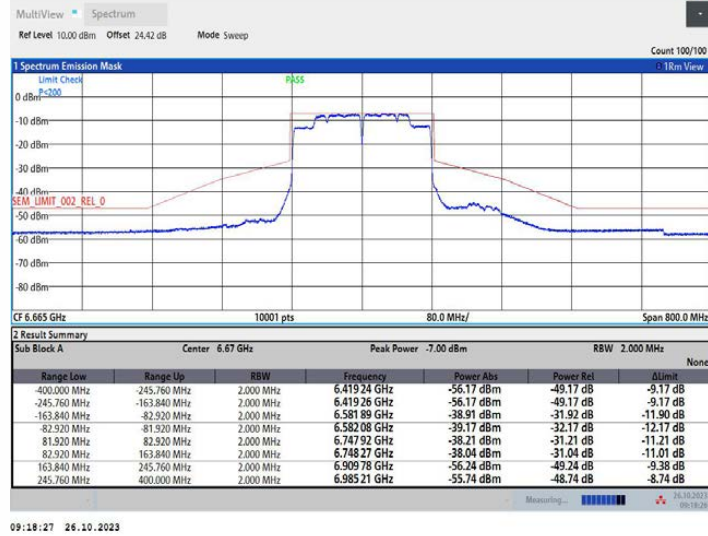
11AC160MIMO_Ant2_6665
