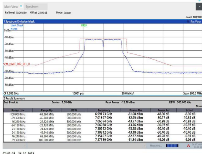
11AC40MIMO_Ant2_7085
