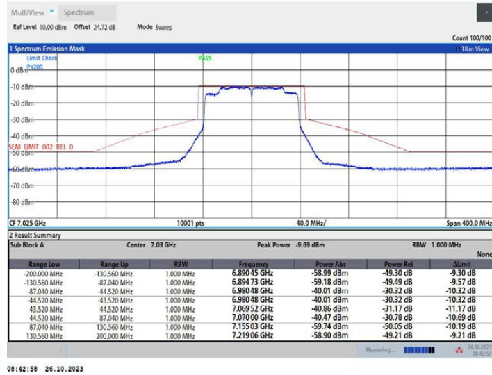
11AC80MIMO_Ant2_7025
