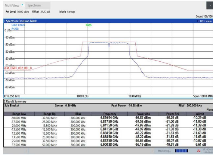
11AX20MIMO_Ant2_6855
