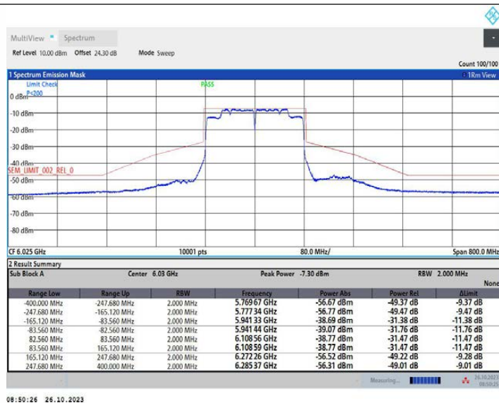
11AC160MIMO_Ant2_6025
