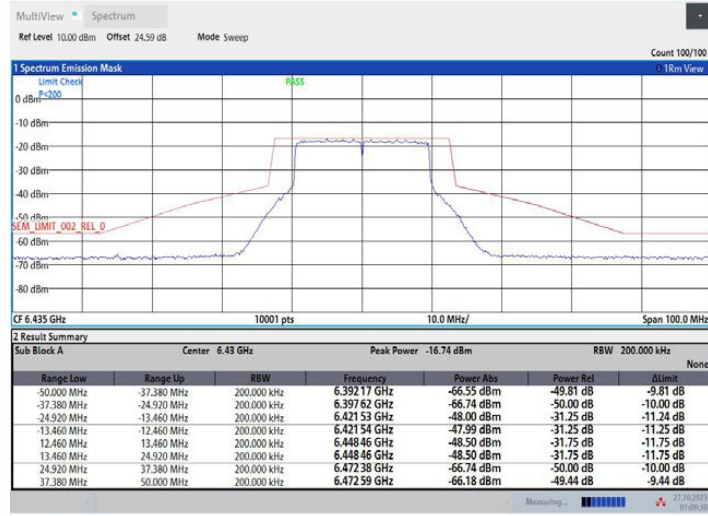
11AX20MIMO_Ant2_6435
