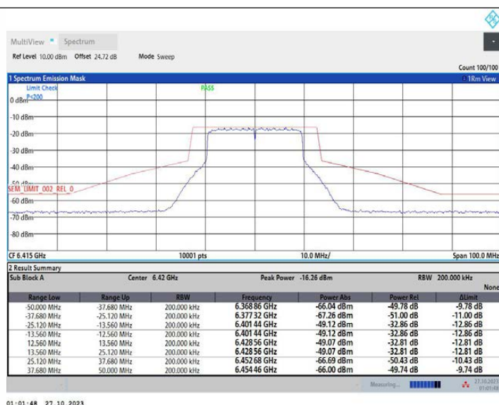
11AX20MIMO_Ant2_6415
