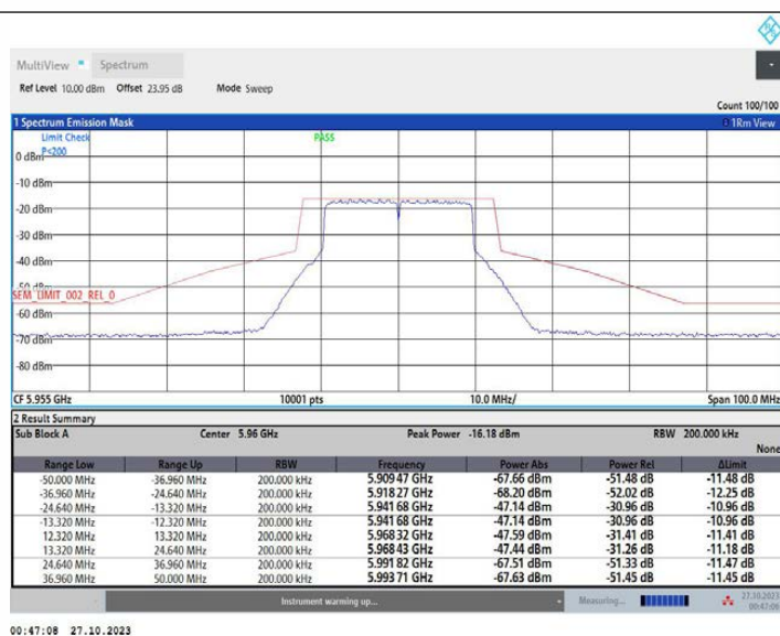
11AX20MIMO_Ant2_5955
