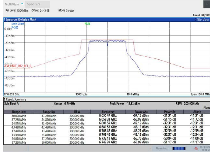
11N20MIMO_Ant2_6695
