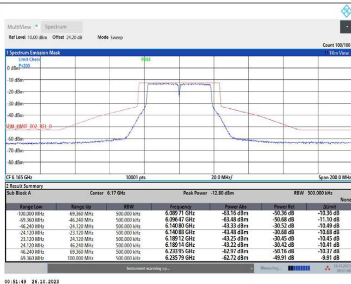
11N40MIMO_Ant2_6165
