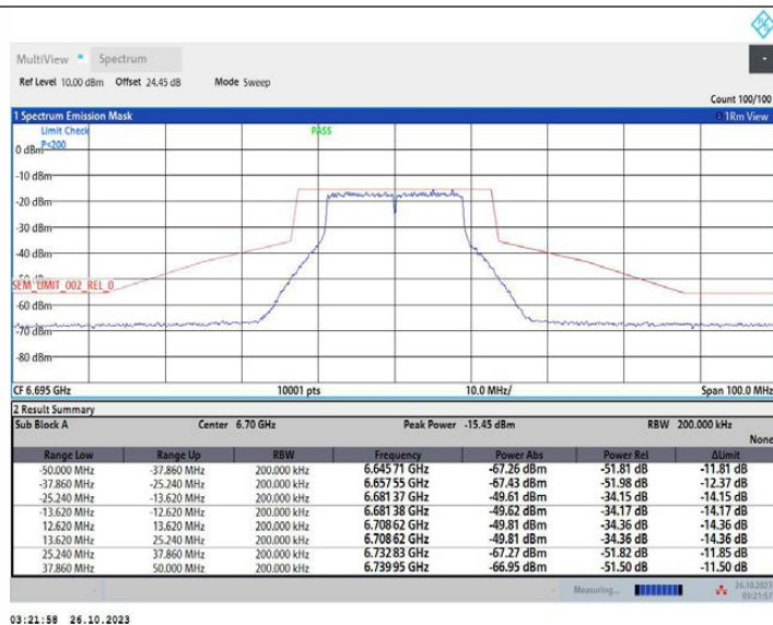
11AC20MIMO_Ant2_6695
