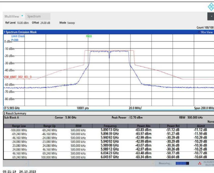
11AC40MIMO_Ant2_5965
