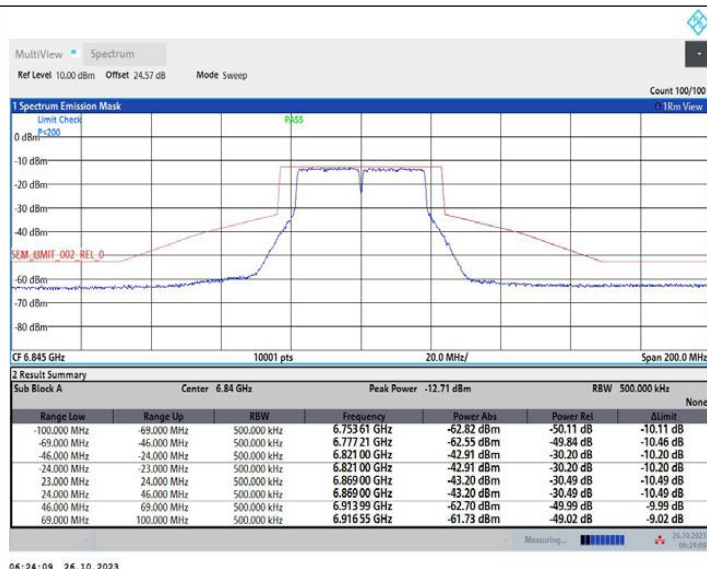
11AC40MIMO_Ant2_6845
