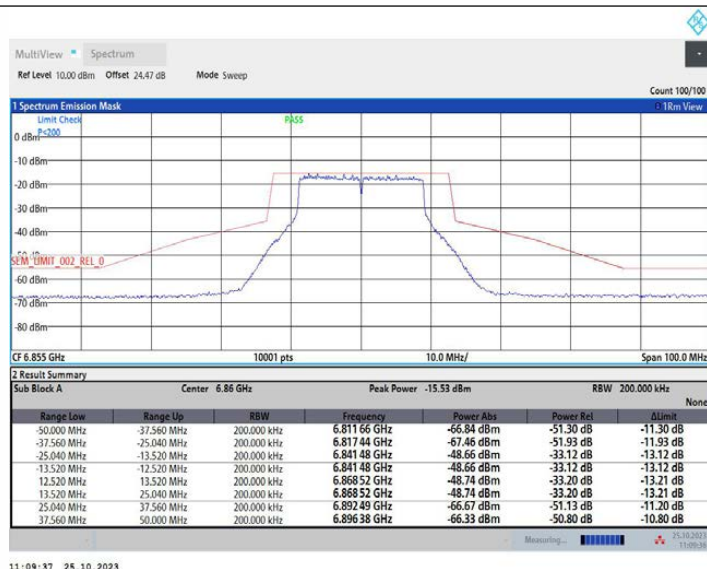
11N20MIMO_Ant2_6855
