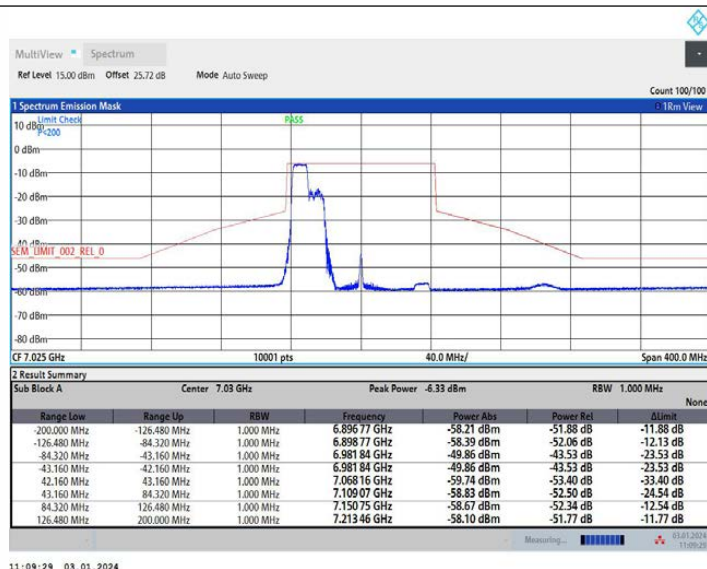
11AX80MIMO Ant1 7025 242Tone RU61
