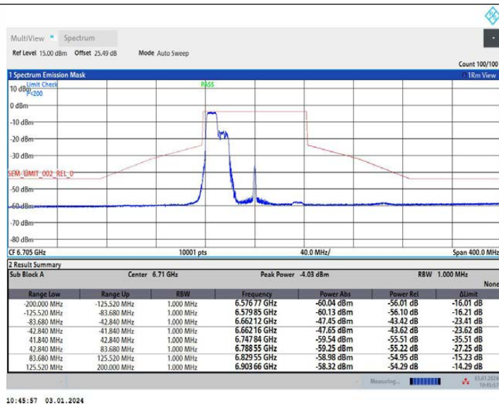
11AX80MIMO Ant1 6705 242Tone RU61
