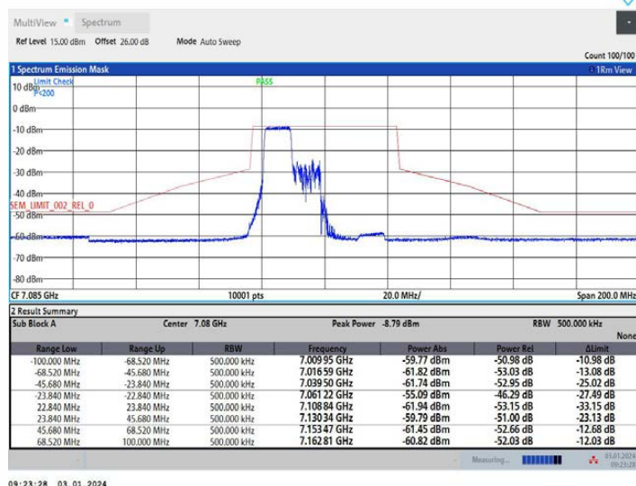
11AX40MIMO Ant1 7085 242Tone RU61
