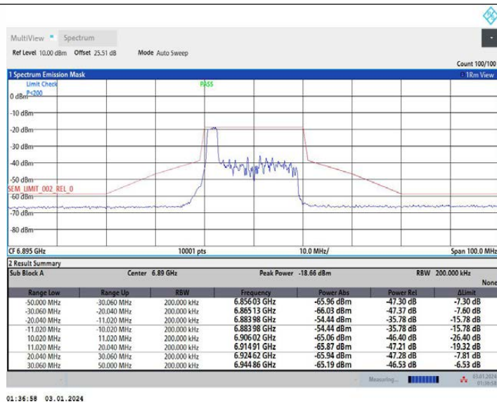
11AX20MIMO_Ant1_6895_52Tone_RU37
