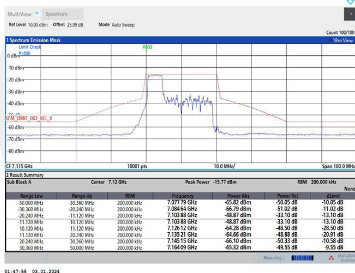
11AX20MIMO_Ant1_7115_106Tone_RU53
