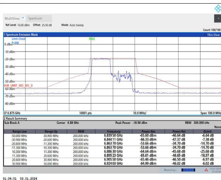
11AX20MIMO_Ant2_6875_26Tone_RU0
