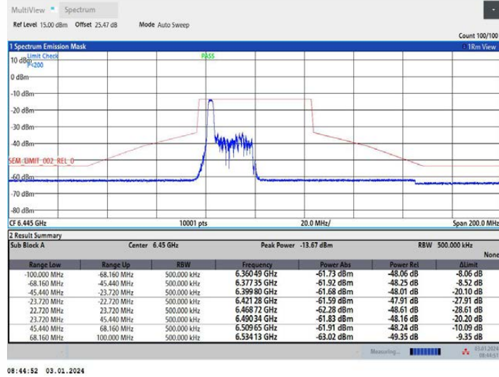
11AX40MIMO Ant1 6445 52Tone RU37
