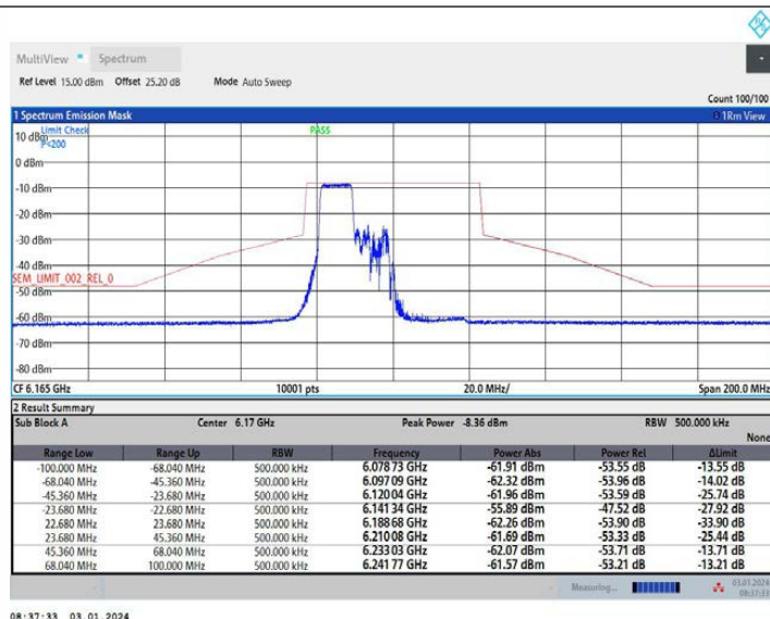
11AX40MIMO Ant1 6165 242Tone RU61
