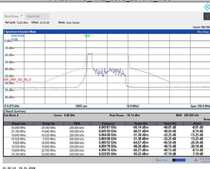
11AX20MIMO_Ant2_6875_52Tone_RU37
