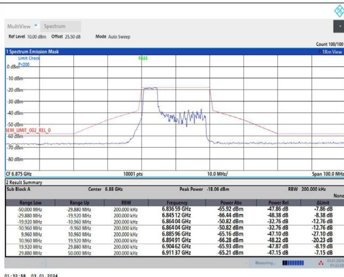
11AX20MIMO_Ant2_6875_106Tone_RU53
