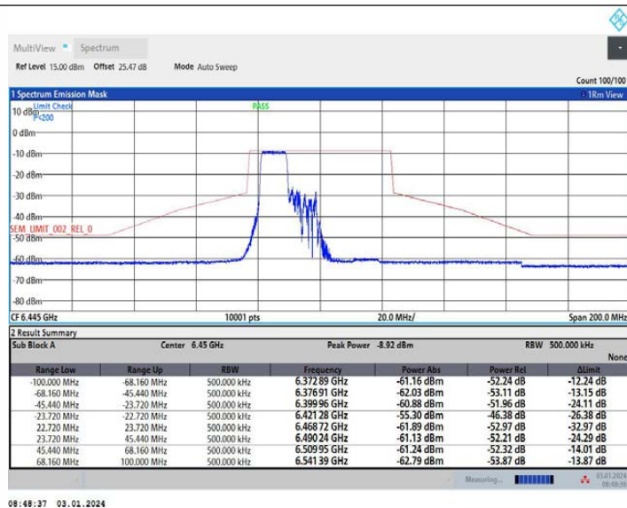
11AX40MIMO Ant1 6445 242Tone RU61
