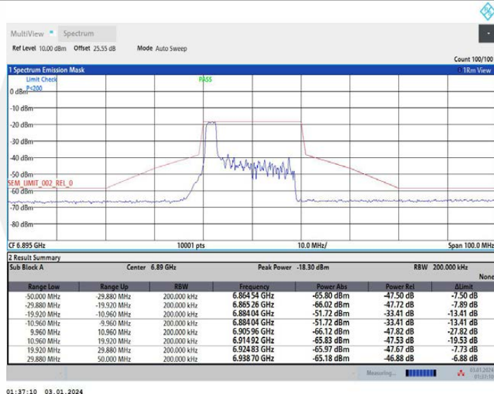
11AX20MIMO_Ant2_6895_52Tone_RU37
