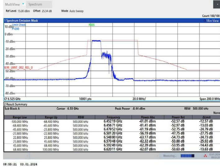
11AX40MIMO Ant1 6525 242Tone RU61
