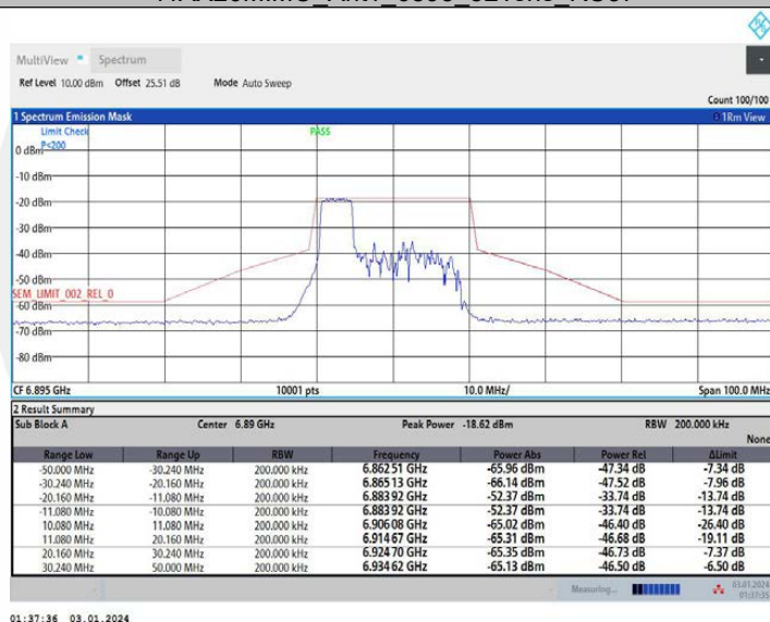
11AX20MIMO_Ant1_6895_106Tone_RU53
