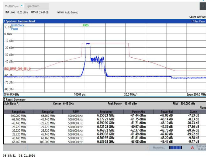
11AX40MIMO Ant1 6445 106Tone RU53
