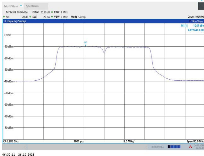
11AC40MIMO_Ant2_6885
