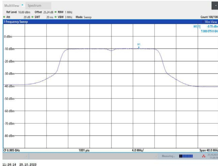
11N20MIMO_Ant2_6995
