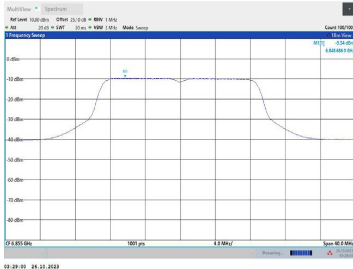
11AC20MIMO_Ant2_6855
