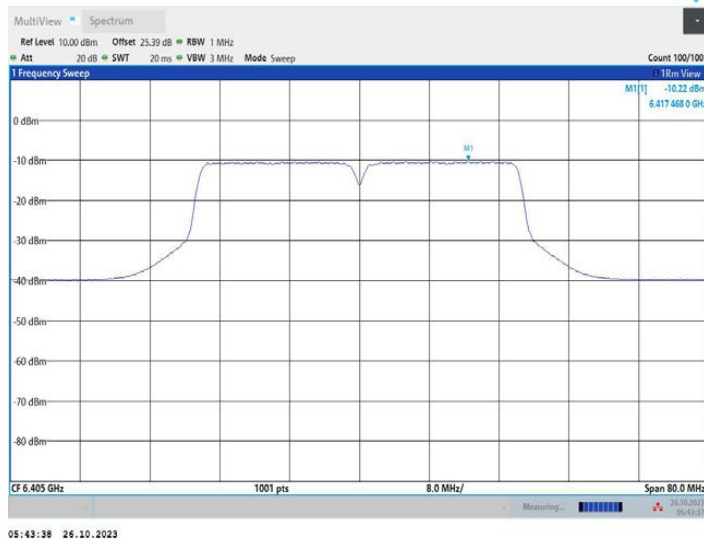
11AC40MIMO_Ant2_6405
