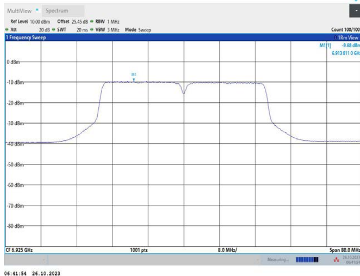
11AC40MIMO_Ant2_6925
