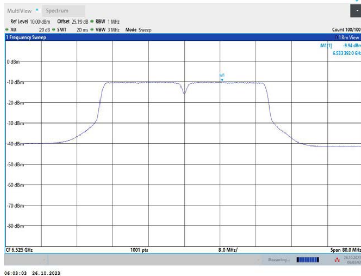
11AC40MIMO_Ant2_6525
