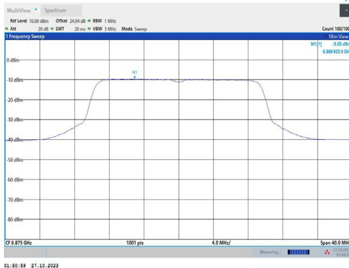
11AX20MIMO_Ant2_6875
