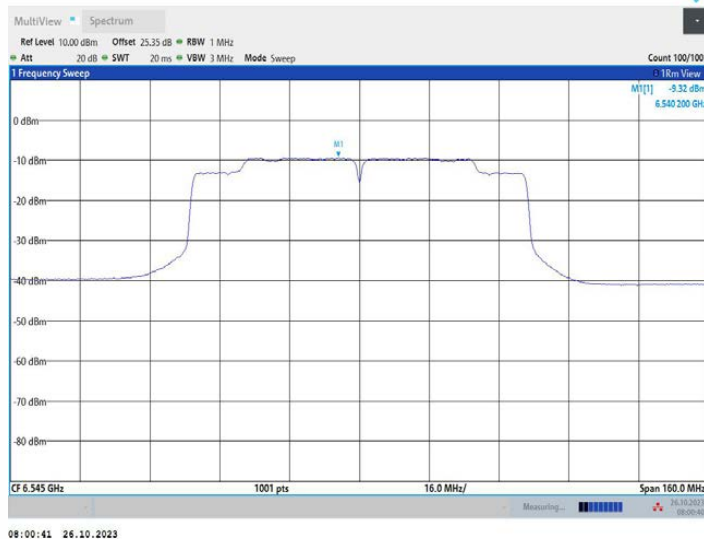
11AC80MIMO_Ant2_6545
