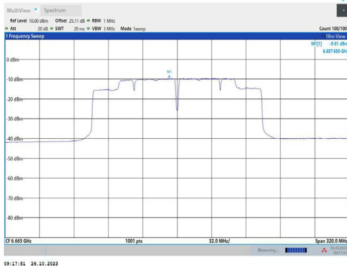
11AC160MIMO_Ant2_6665
