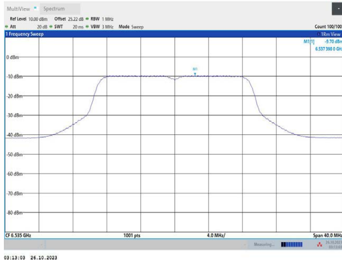
11AC20MIMO_Ant2_6535
