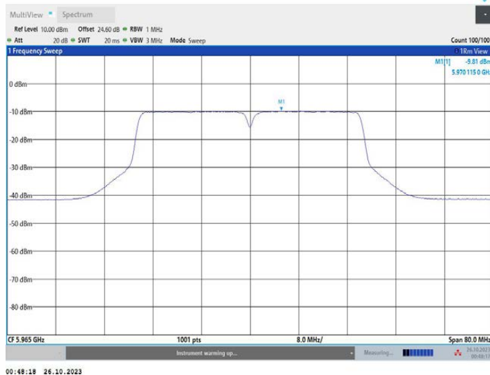
11N40MIMO_Ant2_5965
