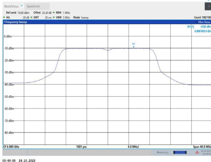
11AC20MIMO_Ant2_6995
