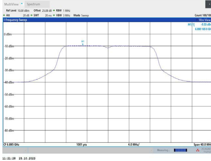
11N20MIMO_Ant2_6895
