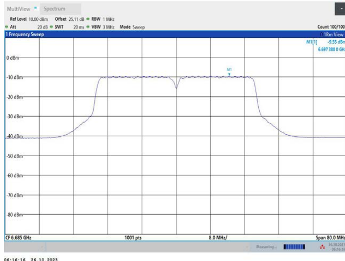
11AC40MIMO_Ant2_6685
