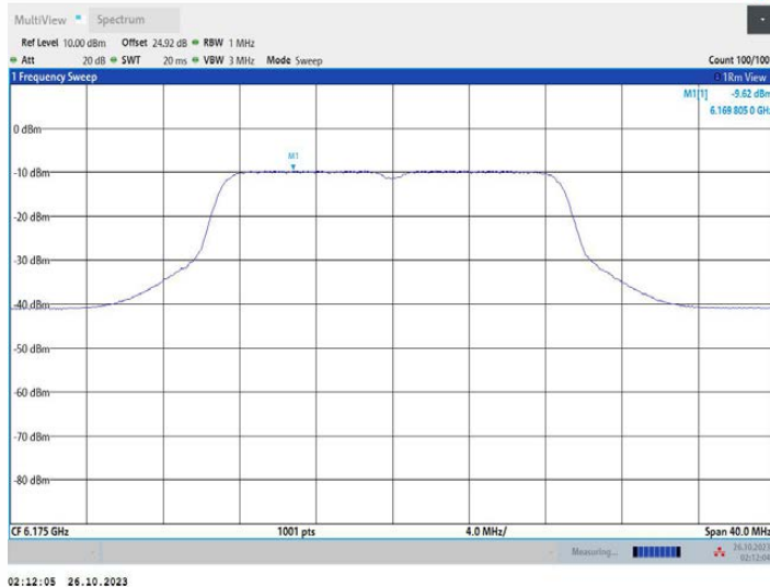
11AC20MIMO_Ant2_6175
