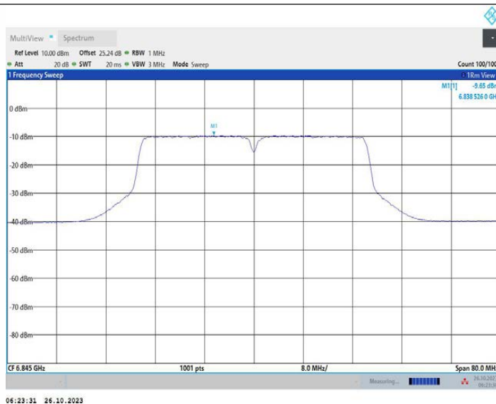
11AC40MIMO_Ant2_6845
