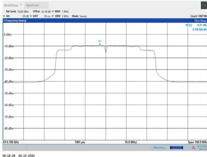
11AC80MIMO_Ant2_6705
