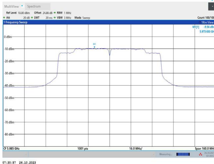
11AC80MIMO_Ant2_5985
