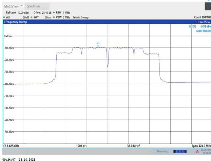
11AC160MIMO_Ant2_6825
