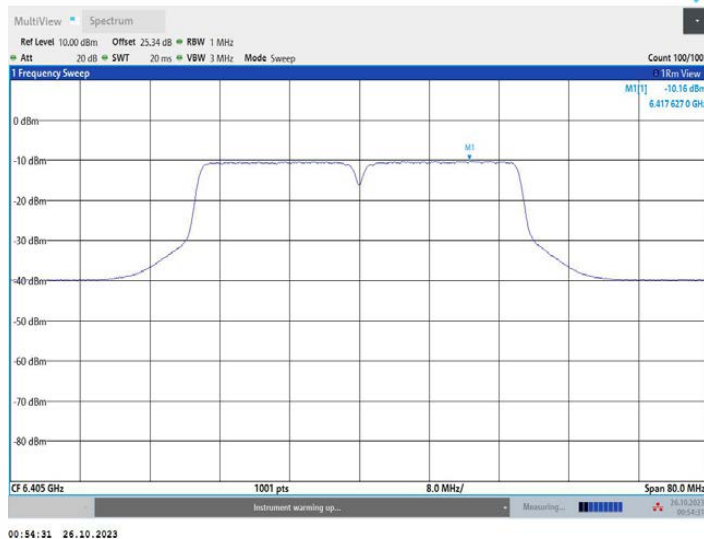
11N40MIMO_Ant2_6405
