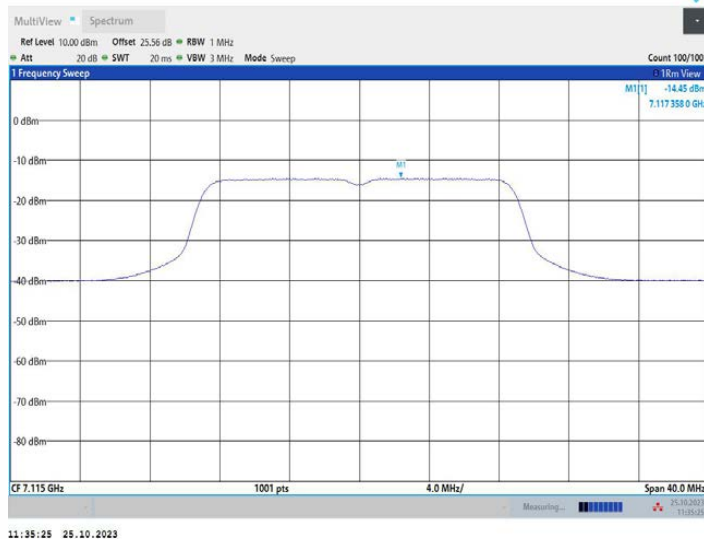
11N20MIMO_Ant2_7115
