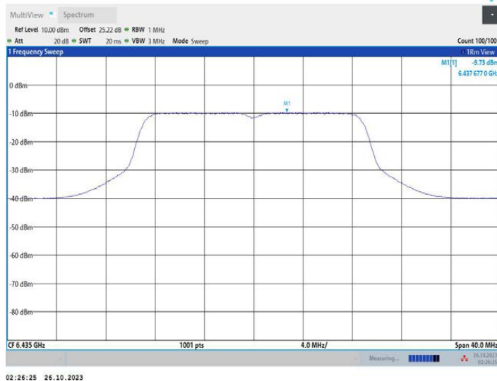
11AC20MIMO_Ant2_6435
