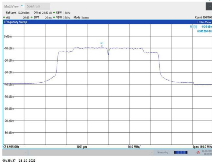
11AC80MIMO_Ant2_6945
