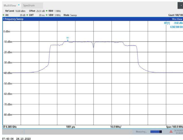
11AC80MIMO_Ant2_6385
