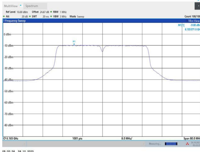
11AC40MIMO_Ant2_6165
