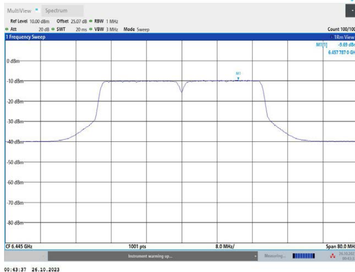
11N40MIMO_Ant2_6445
