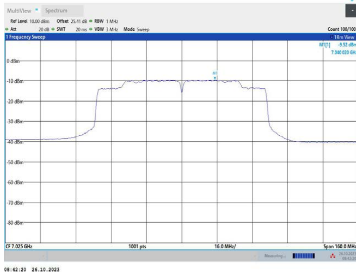
11AC80MIMO_Ant2_7025
