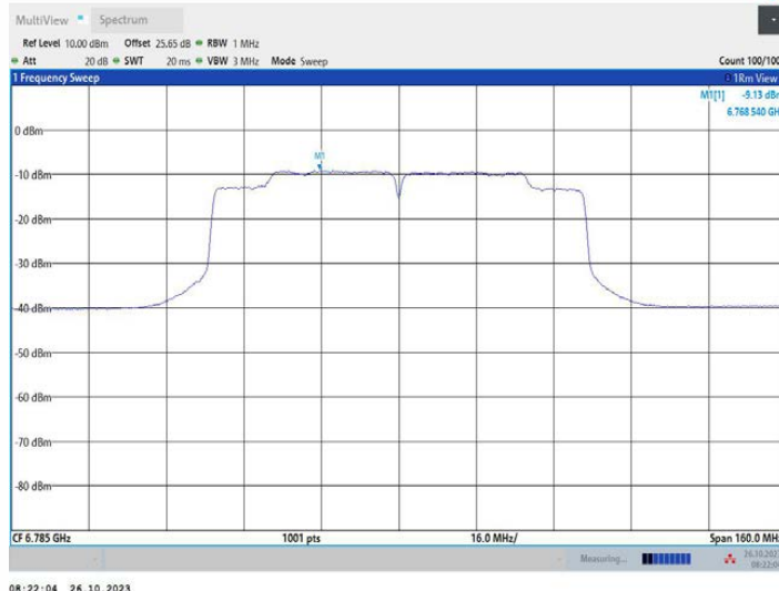
11AC80MIMO_Ant2_6785
