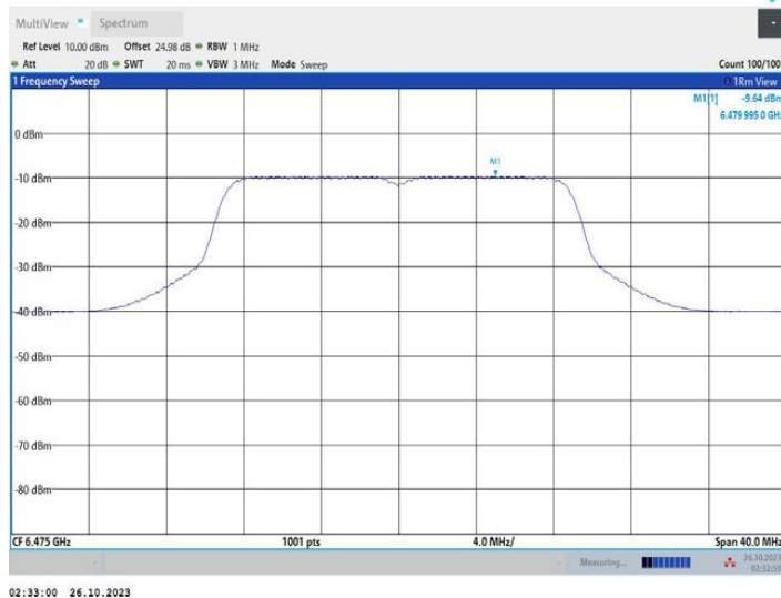
11AC20MIMO_Ant2_6475
