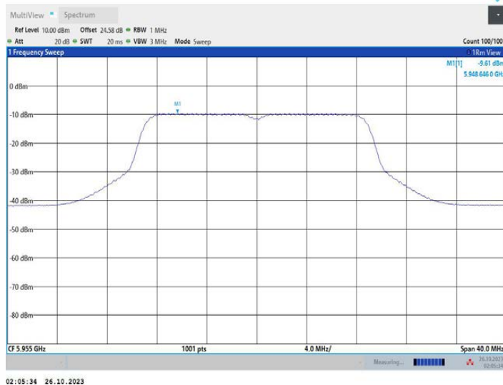
11AC20MIMO_Ant2_5955
