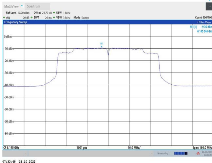
11AC80MIMO_Ant2_6145
