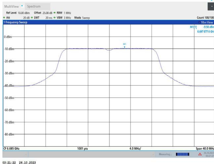
11AC20MIMO_Ant2_6695
