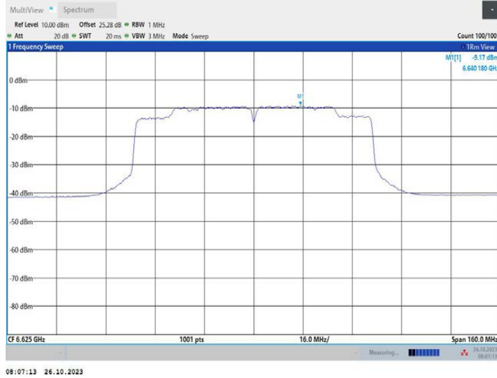
11AC80MIMO_Ant2_6625
