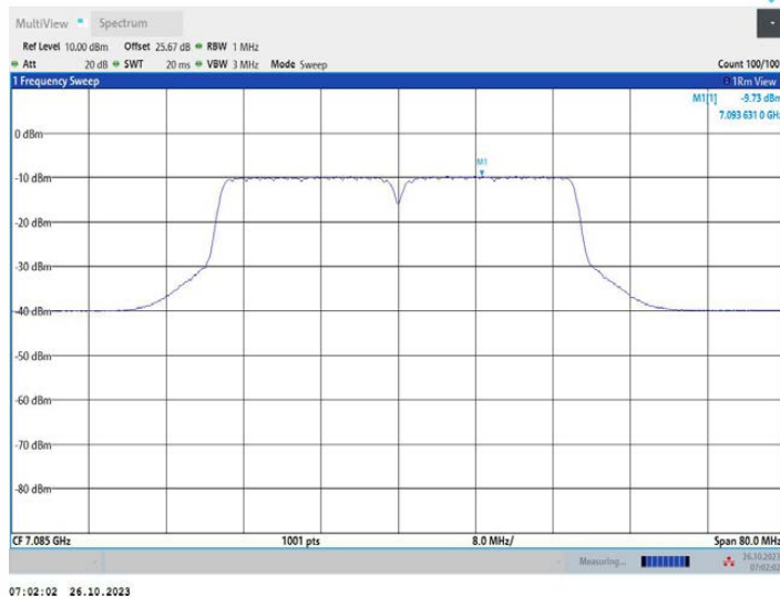
11AC40MIMO_Ant2_7085
