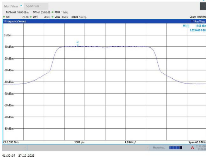
11AX20MIMO_Ant2_6535
