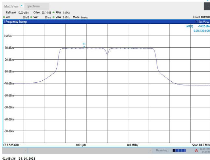
11N40MIMO_Ant2_6525
