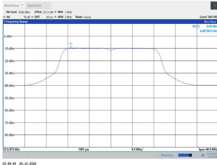
11AC20MIMO_Ant2_6875
