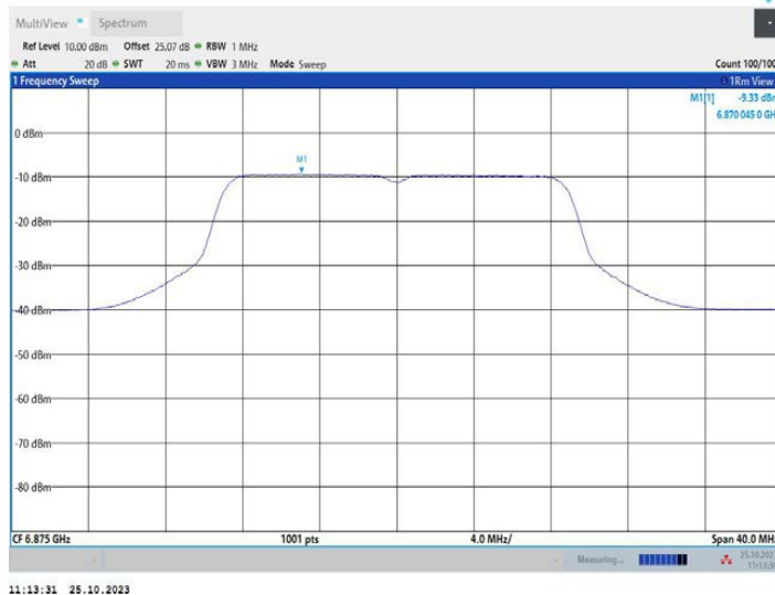
11N20MIMO_Ant2_6875
