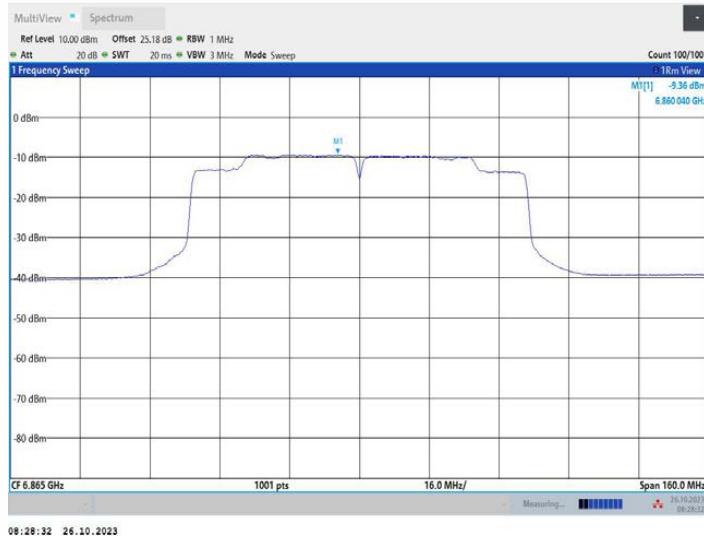
11AC80MIMO_Ant2_6865
