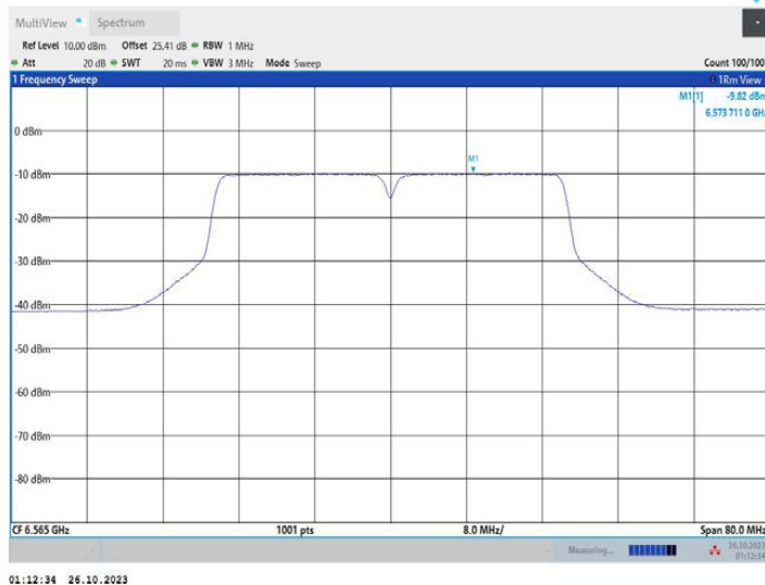
11N40MIMO_Ant2_6565
