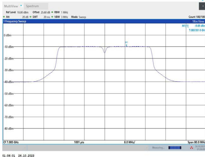
11N40MIMO_Ant2_7085
