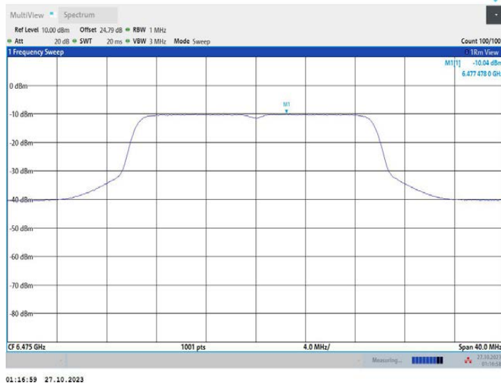
11AX20MIMO_Ant2_6475
