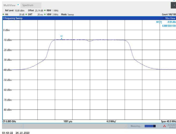
11AC20MIMO_Ant2_6895
