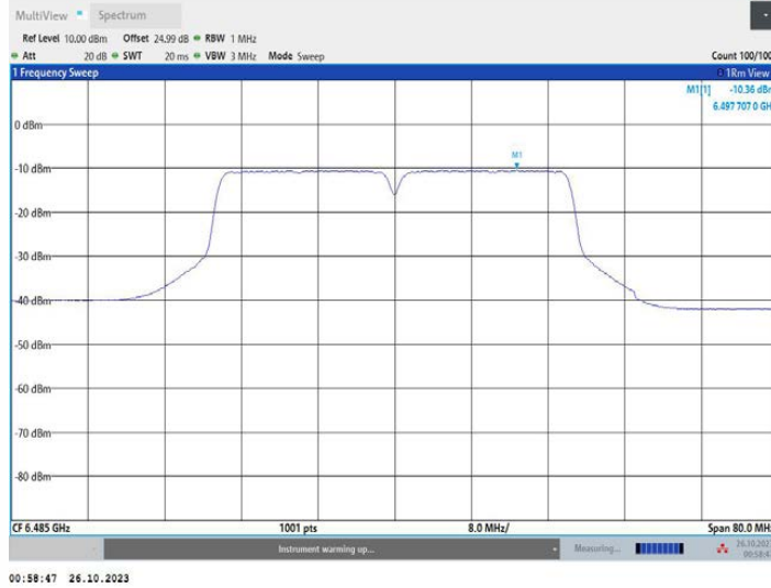
11N40MIMO_Ant2_6485
