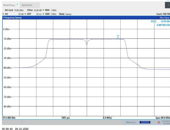
11AC40MIMO_Ant2_6485
