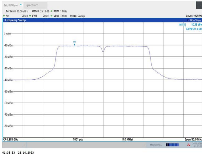
11N40MIMO_Ant2_6885
