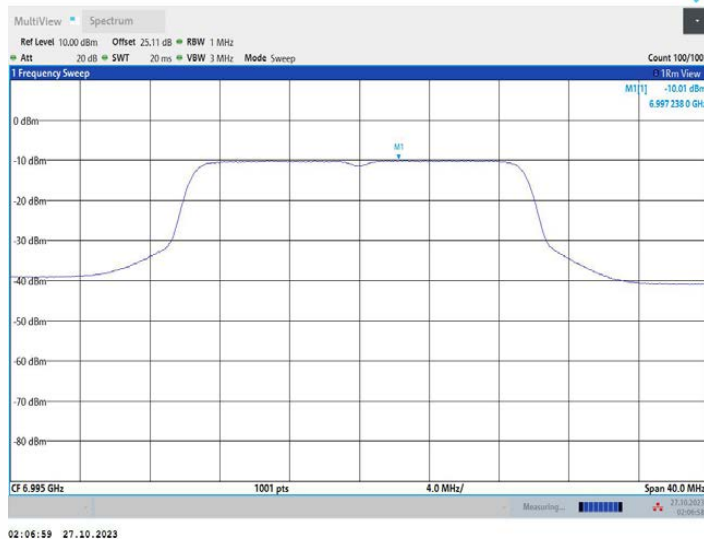
11AX20MIMO_Ant2_6995
