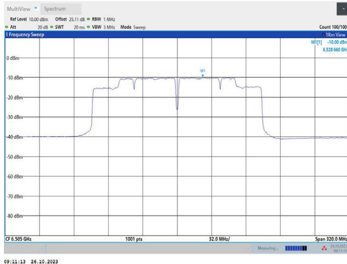
11AC160MIMO_Ant2_6505
