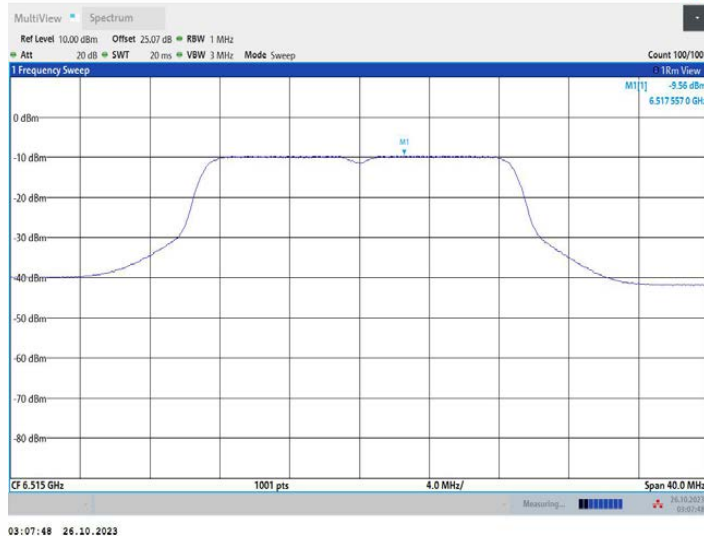
11AC20MIMO_Ant2_6515
