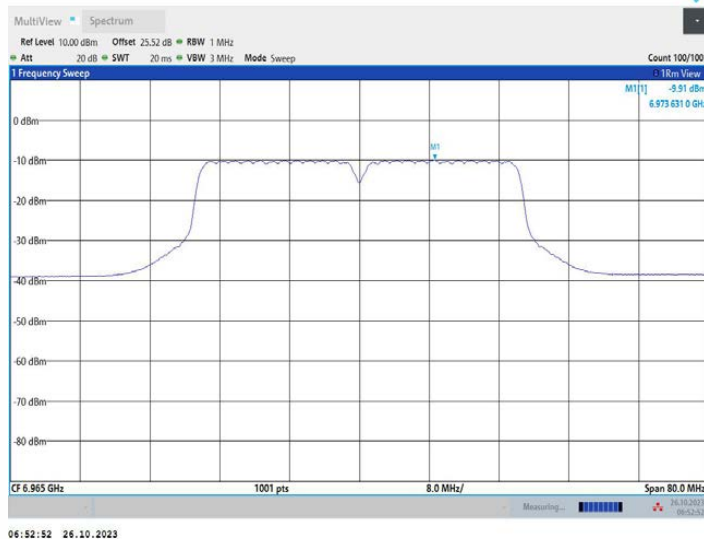
11AC40MIMO_Ant2_6965
