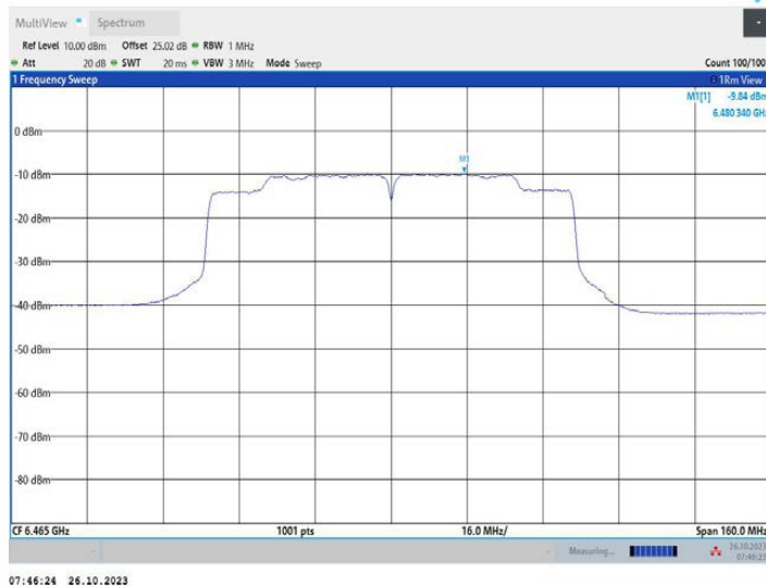
11AC80MIMO_Ant2_6465
