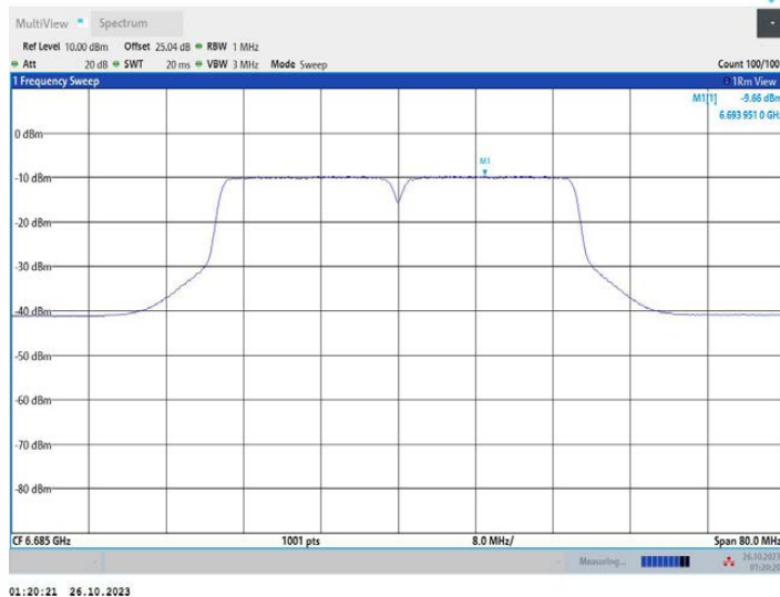
11N40MIMO_Ant2_6685
