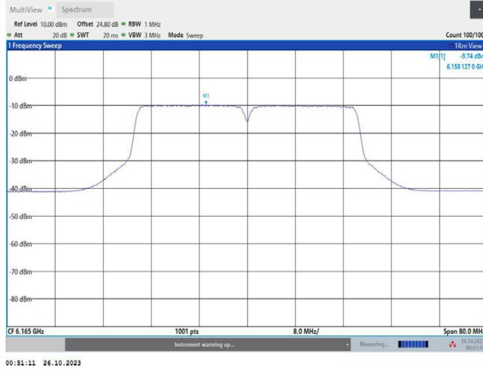
11N40MIMO_Ant2_6165
