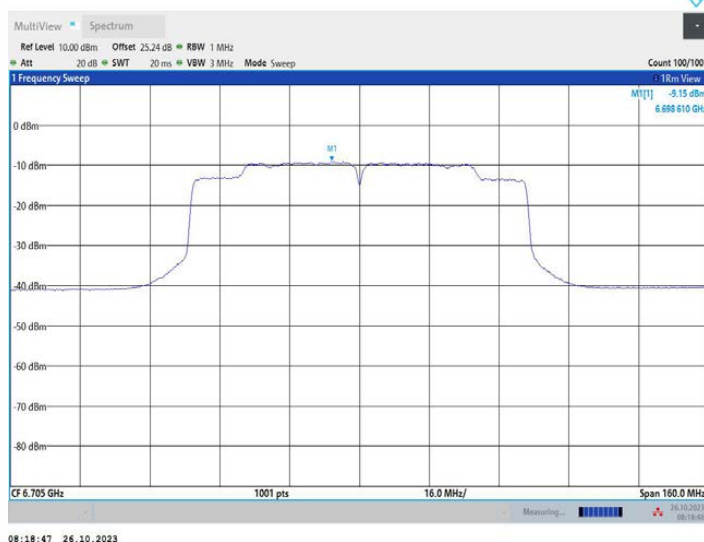
11AC80MIMO_Ant1_6785
