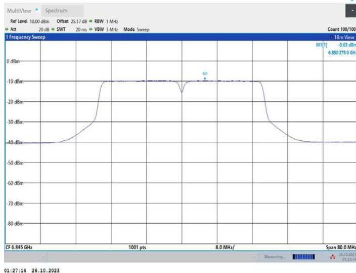
11N40MIMO_Ant2_6845
