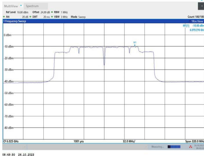
11AC160MIMO_Ant2_6025
