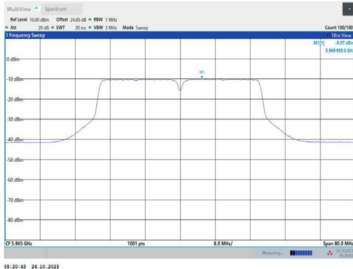
11AC40MIMO_Ant2_5965
