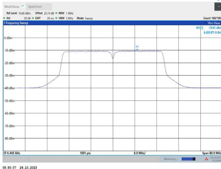
11AC40MIMO_Ant2_6445
