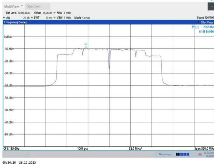
11AC160MIMO_Ant2_6185
