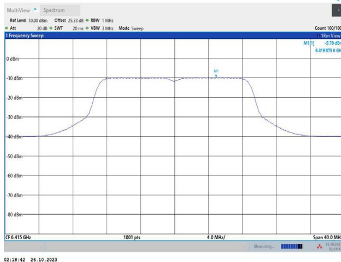
11AC20MIMO_Ant2_6415
