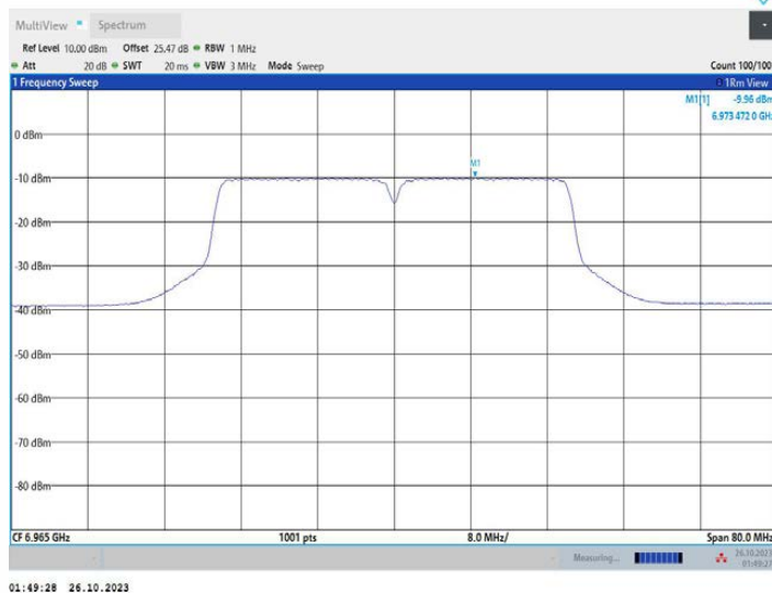
11N40MIMO_Ant2_6965
