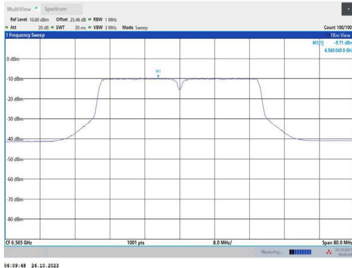
11AC40MIMO_Ant2_6565
