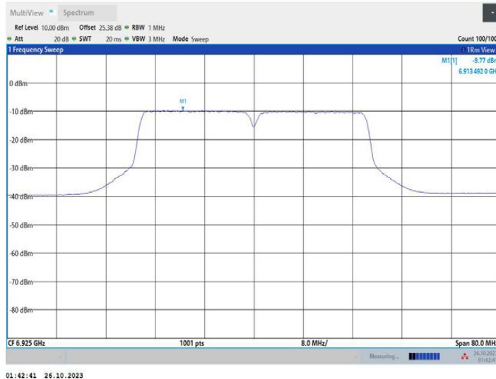
11N40MIMO_Ant2_6925
