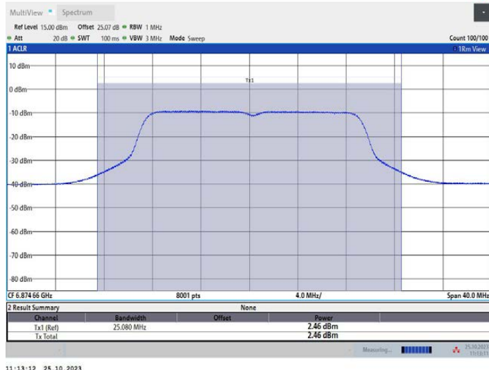
11N20MIMO_Ant2_6875
