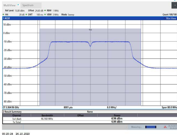
11AC40MIMO_Ant2_5965
