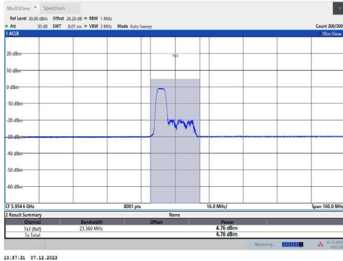
11AX80MIMO_Ant1_5985_106Tone_RU53
