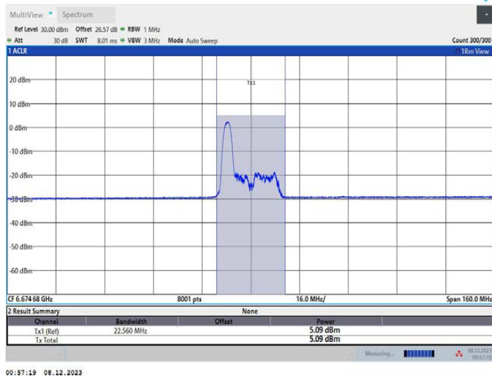
11AX80MIMO_Ant1_6705_52Tone_RU37
