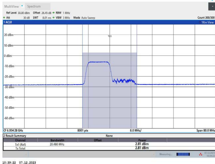
11AX40MIMO_Ant2_6965_242Tone_RU61
