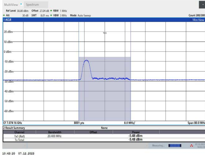
11AX40MIMO_Ant1_7085_52Tone_RU37
