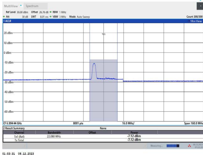
11AX80MIMO_Ant1_7025_52Tone_RU37
