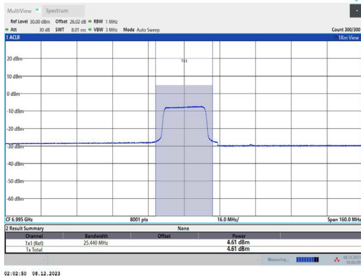
11AX80MIMO_Ant2_7025_484Tone_RU65
