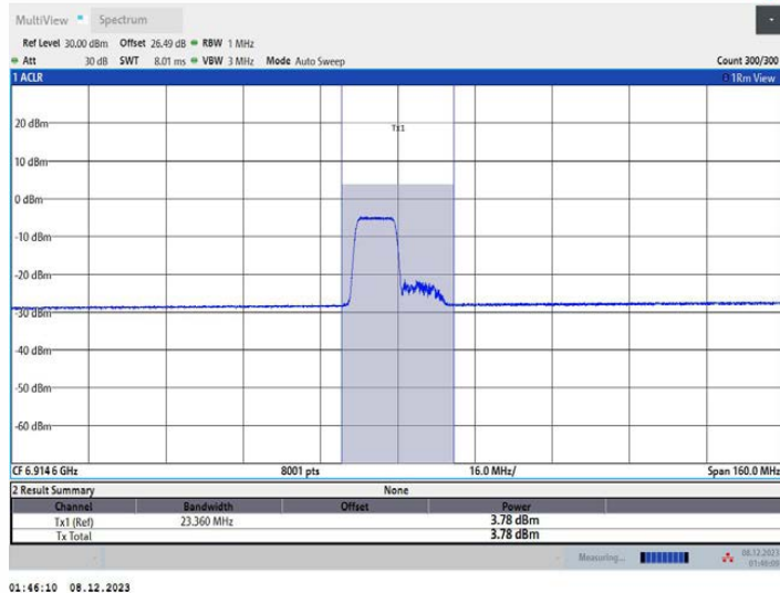
11AX80MIMO_Ant1_6945_242Tone_RU61
