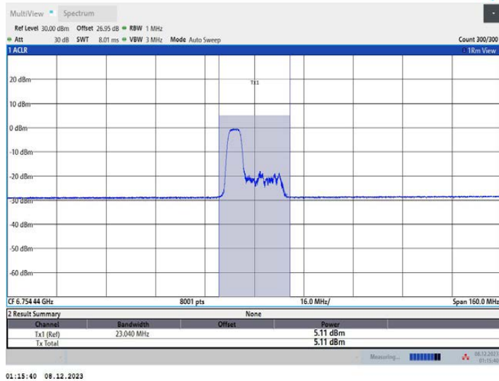
11AX80MIMO_Ant1_6785_106Tone_RU53
