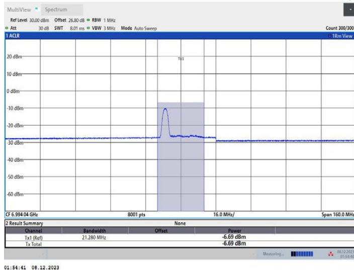
11AX80MIMO_Ant2_7025_52Tone_RU37
