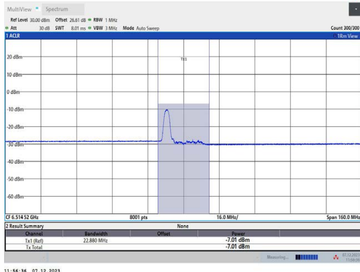
11AX80MIMO_Ant1_6545_52Tone_RU37
