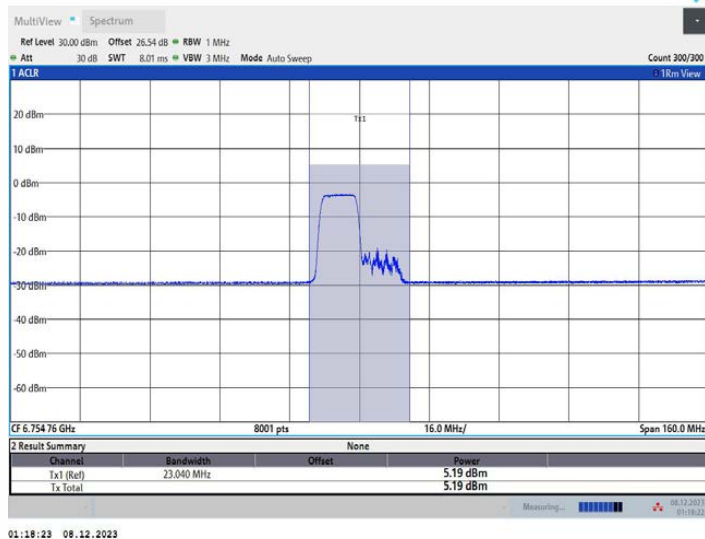
11AX80MIMO_Ant1_6785_242Tone_RU61
