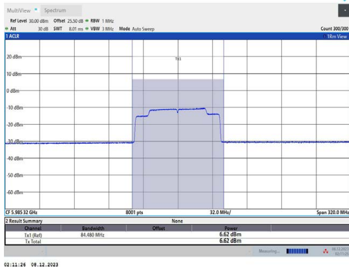
11AX160MIMO_Ant2_6025_996Tone_RU67
