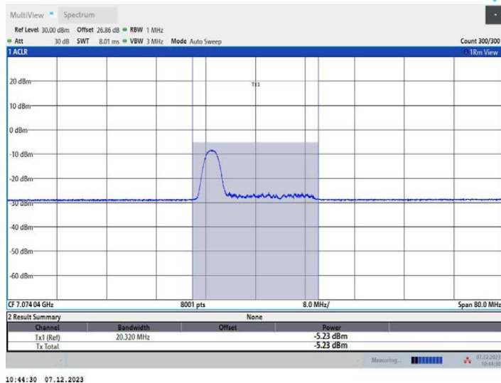
11AX40MIMO_Ant2_7085_52Tone_RU37
