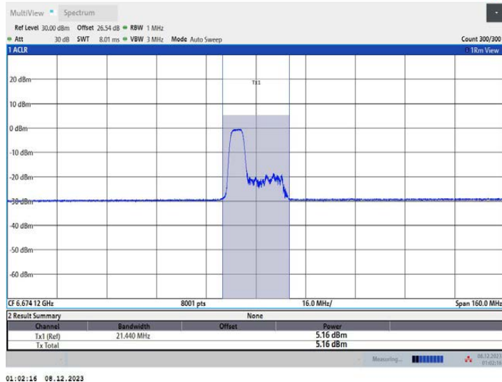
11AX80MIMO_Ant2_6705_106Tone_RU53
