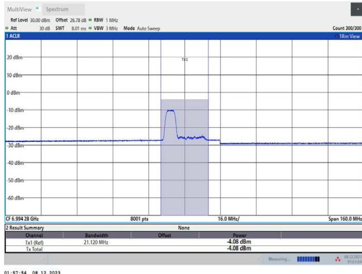
11AX80MIMO_Ant2_7025_106Tone_RU53
