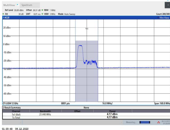
11AX80MIMO_Ant2_6865_106Tone_RU53
