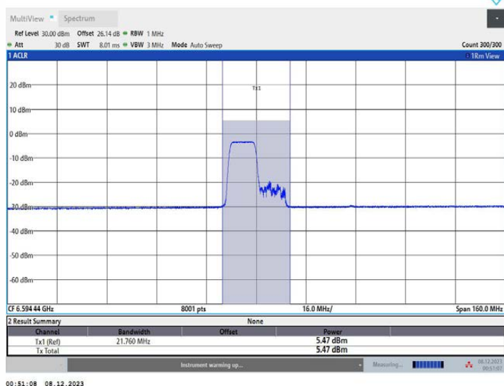
11AX80MIMO_Ant2_6625_242Tone_RU61
