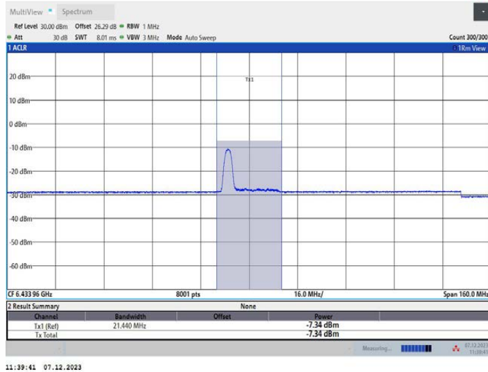
11AX80MIMO_Ant2_6465_52Tone_RU37
