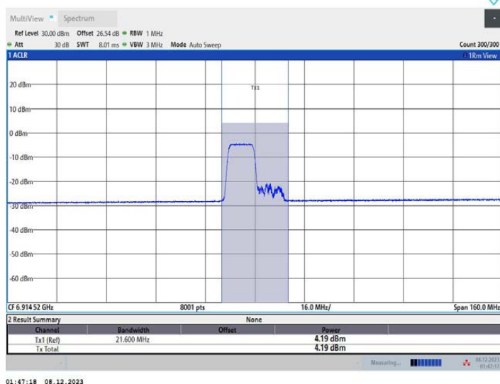
11AX80MIMO_Ant2_6945_242Tone_RU61
