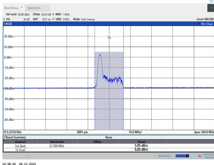
11AX80MIMO_Ant2_6705_52Tone_RU37
