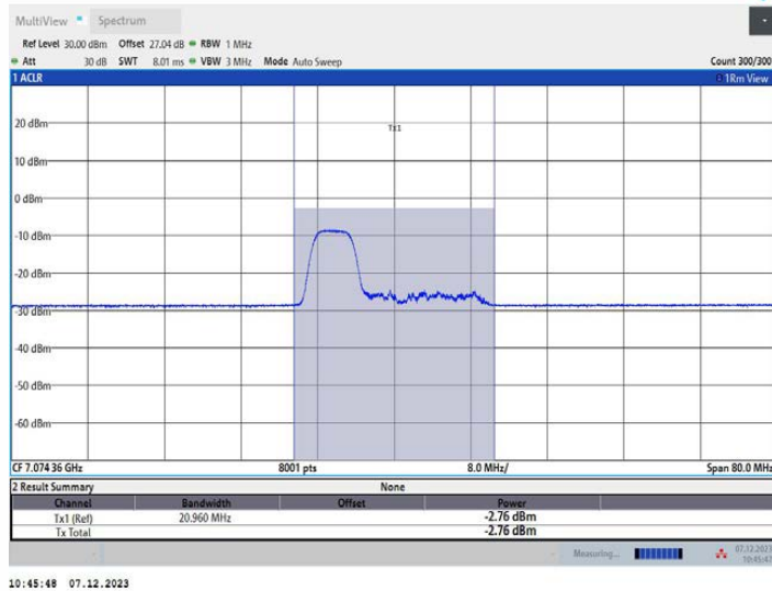
11AX40MIMO_Ant1_7085_106Tone_RU53
