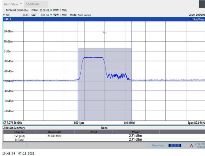
11AX40MIMO_Ant1_7085_242Tone_RU61
