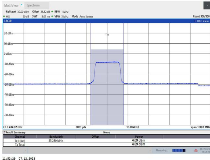
11AX80MIMO_Ant2_6465_484Tone_RU65
