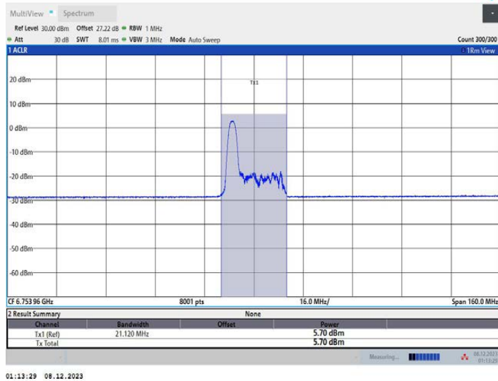
11AX80MIMO_Ant2_6785_52Tone_RU37
