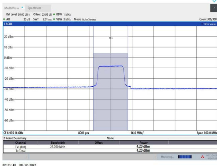
11AX80MIMO_Ant1_7025_484Tone_RU65
