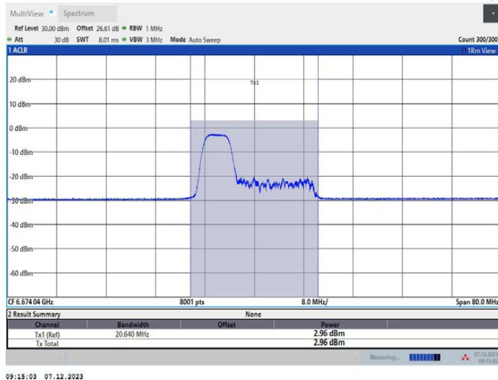
11AX40MIMO_Ant2_6685_106Tone_RU53
