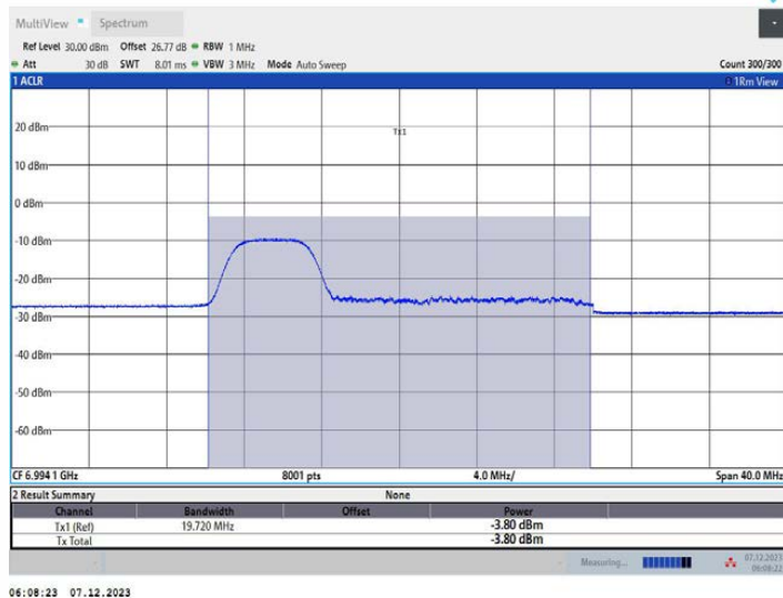
11AX20MIMO_Ant2_6995_106Tone_RU53
