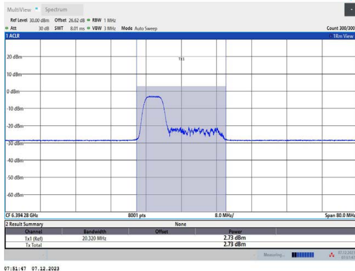
11AX40MIMO_Ant2_6405_106Tone_RU53
