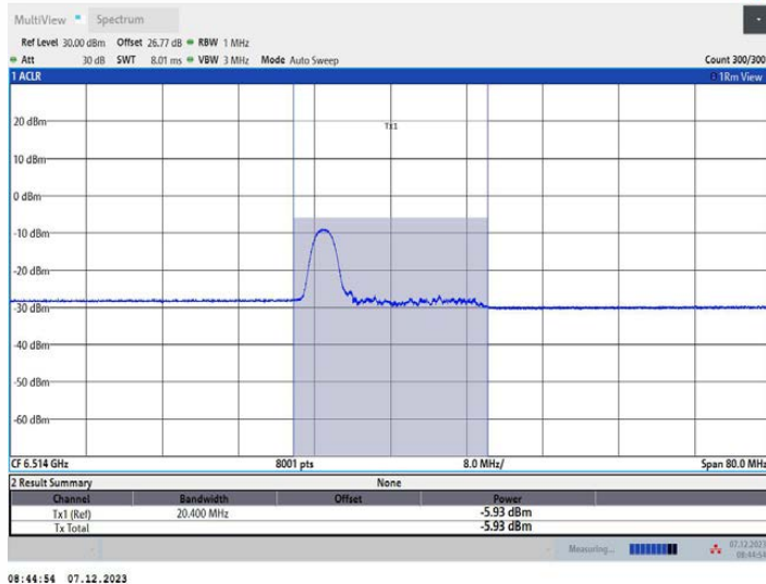
11AX40MIMO_Ant2_6525_52Tone_RU37
