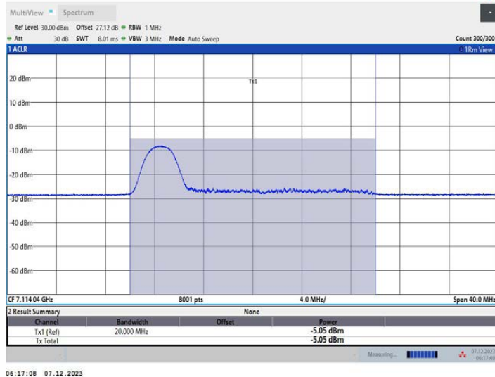
11AX20MIMO_Ant1_7115_52Tone_RU37
