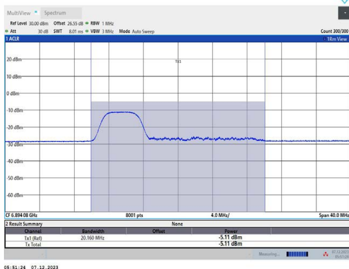
11AX20MIMO_Ant1_6895_106Tone_RU53
