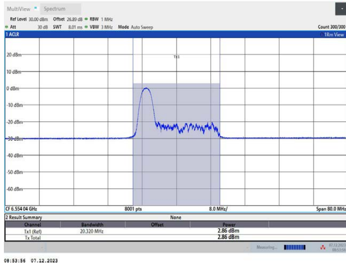
11AX40MIMO_Ant1_6565_52Tone_RU37
