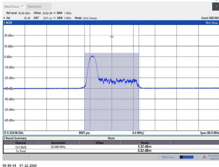
11AX40MIMO_Ant2_6565_52Tone_RU37
