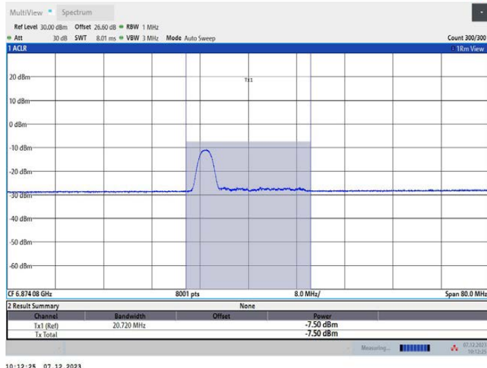
11AX40MIMO_Ant1_6885_52Tone_RU37
