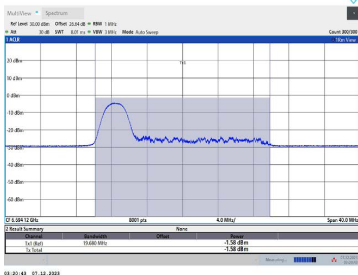
11AX20MIMO_Ant2_6695_52Tone_RU37
