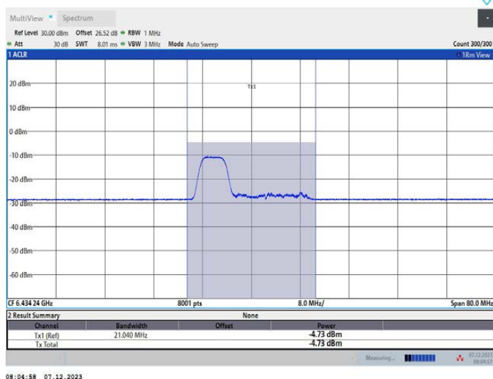
11AX40MIMO_Ant1_6445_106Tone_RU53
