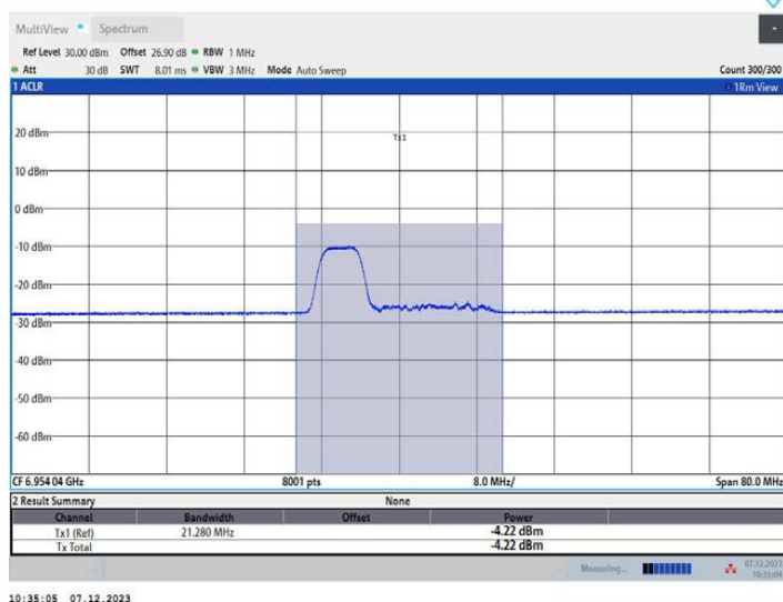
11AX40MIMO_Ant1_6965_106Tone_RU53
