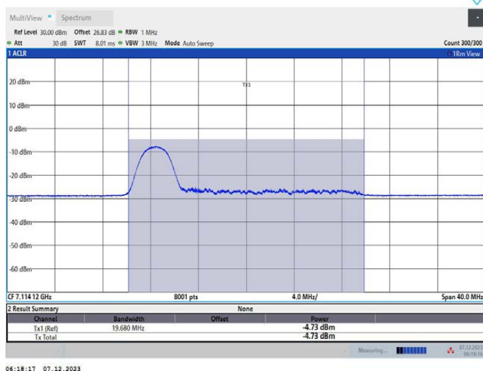
11AX20MIMO_Ant2_7115_52Tone_RU37
