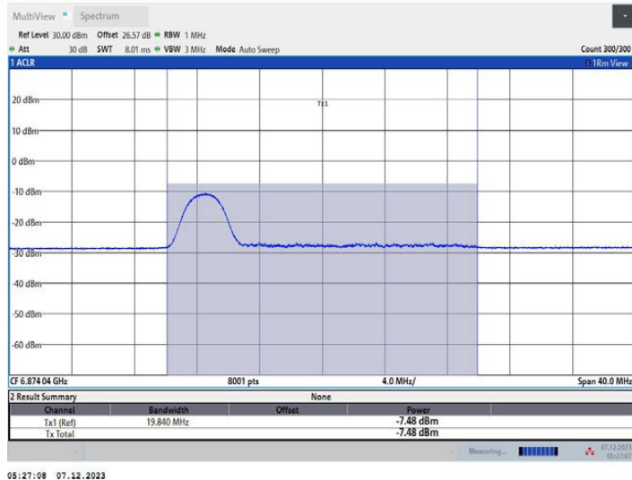
11AX20MIMO_Ant1_6875_52Tone_RU37
