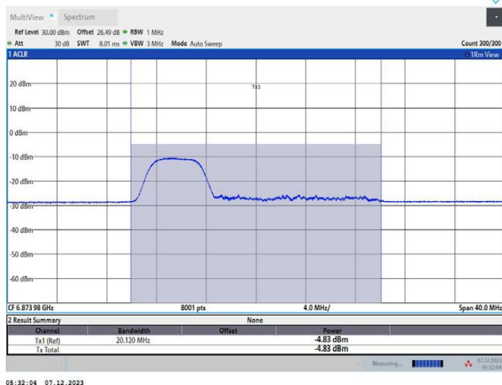
11AX20MIMO_Ant1_6875_106Tone_RU53
