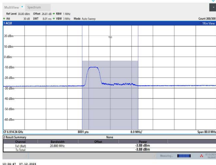
11AX40MIMO_Ant1_6925_106Tone_RU53
