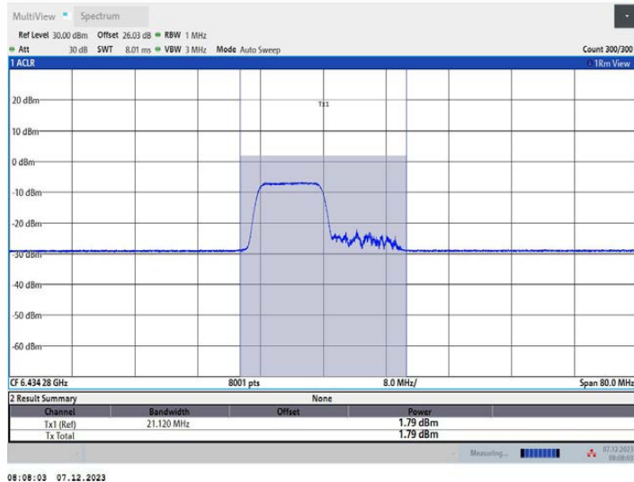
11AX40MIMO_Ant1_6445_242Tone_RU61
