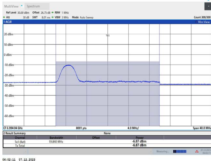
11AX20MIMO_Ant1_6995_52Tone_RU37
