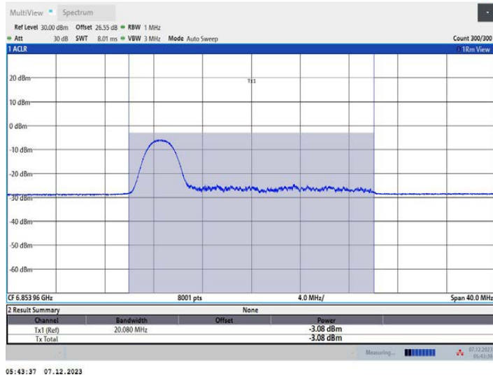
11AX20MIMO_Ant1_6855_52Tone_RU37
