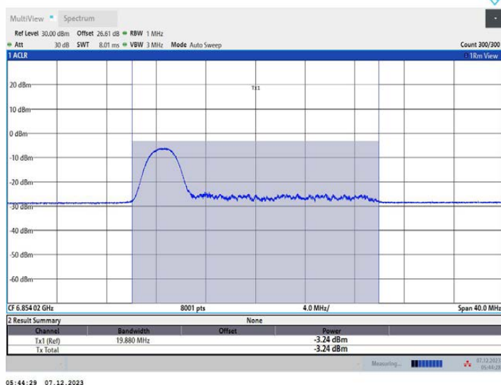
11AX20MIMO_Ant2_6855_52Tone_RU37
