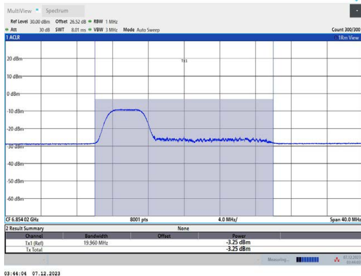
11AX20MIMO_Ant2_6855_106Tone_RU53
