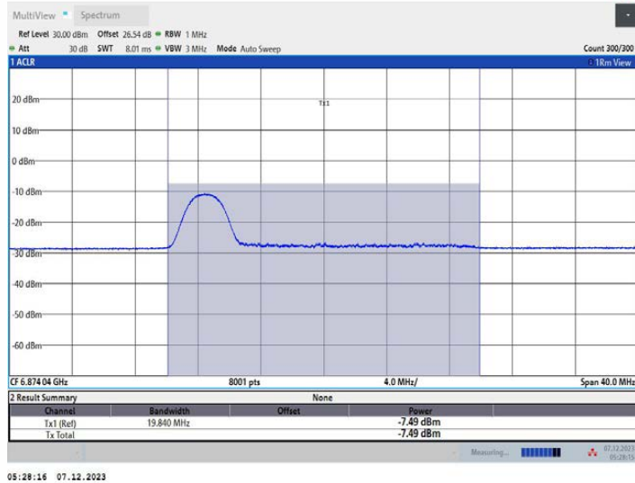
11AX20MIMO_Ant2_6875_52Tone_RU37
