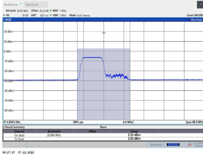
11AX40MIMO_Ant2_6845_242Tone_RU61
