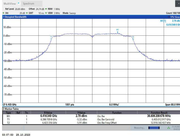
11N40MIMO_Ant2_6405
