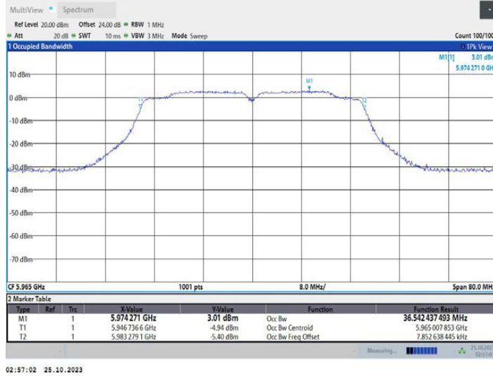
11N40MIMO_Ant2_5965
