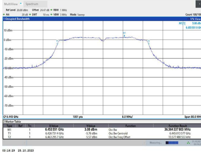
11N40MIMO_Ant2_6445
