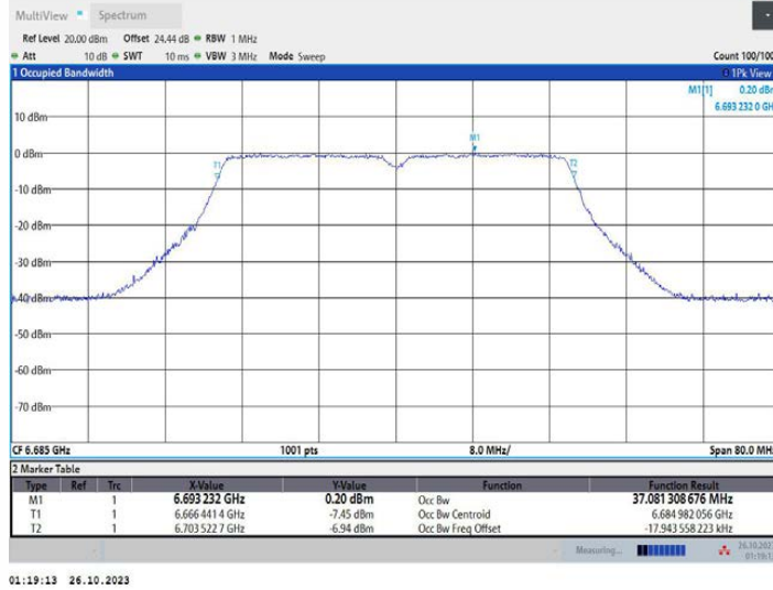
11N40MIMO_Ant2_6685
