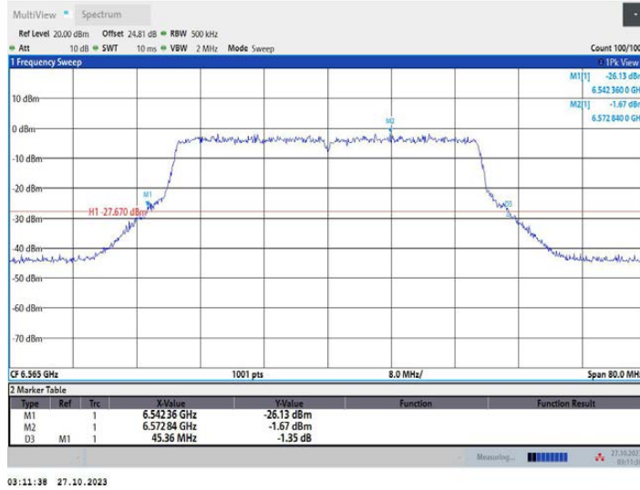
11AX40MIMO_Ant2_6565
