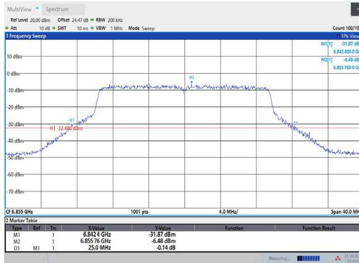
11AX20MIMO_Ant2_6855
