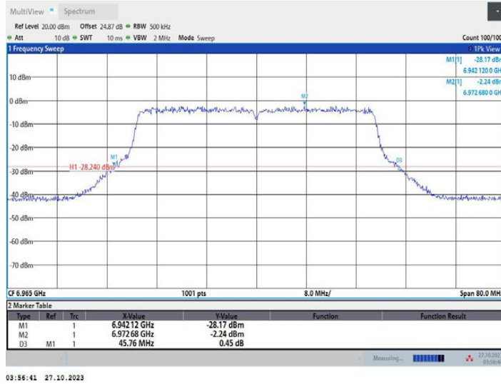
11AX40MIMO_Ant2_6965
