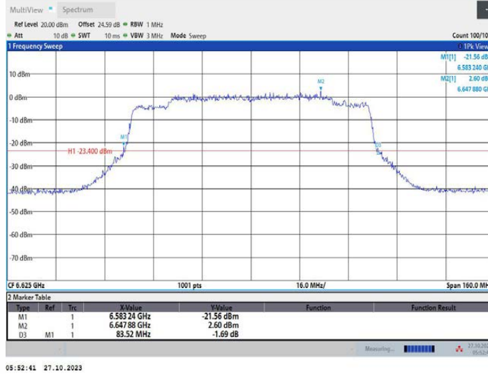
11AX80MIMO_Ant2_6625
