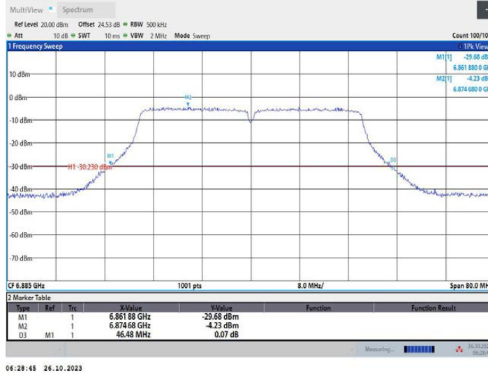
11AC40MIMO_Ant2_6885
