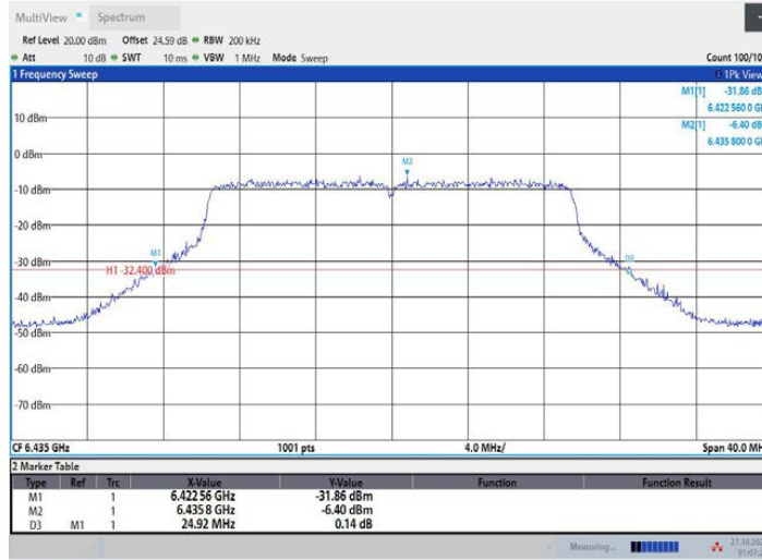
11AX20MIMO_Ant2_6435
