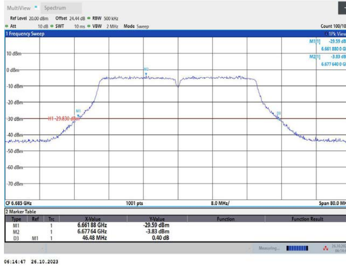
11AC40MIMO_Ant2_6685
