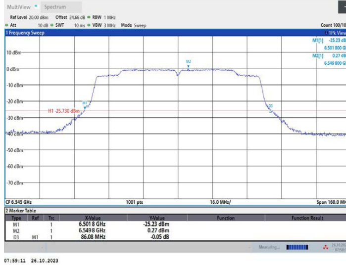
11AC80MIMO_Ant2_6545
