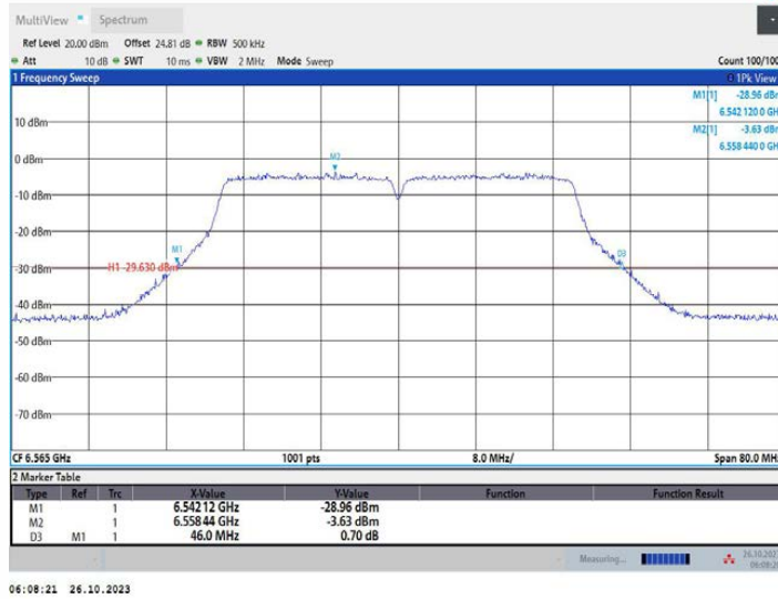
11AC40MIMO_Ant2_6565
