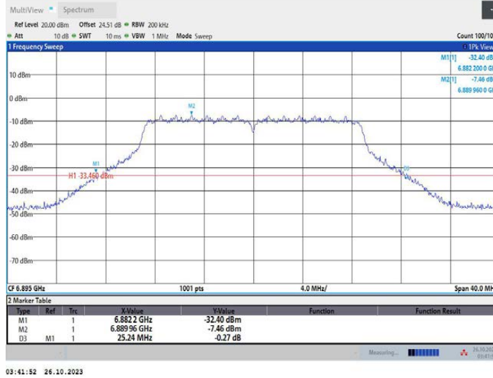
11AC20MIMO_Ant2_6895
