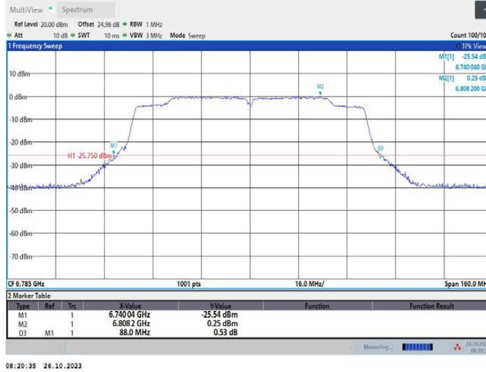
11AC80MIMO_Ant2_6785
