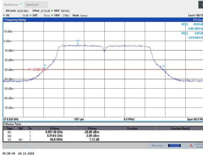
11AC40MIMO_Ant2_6925
