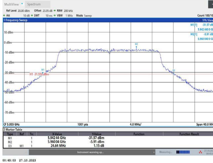
11AX20MIMO_Ant2_5955
