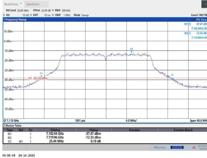
11AC20MIMO_Ant2_7115
