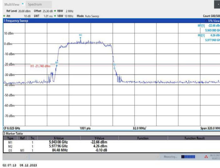
11AX160MIMO_Ant2_6025_996Tone_RU67
