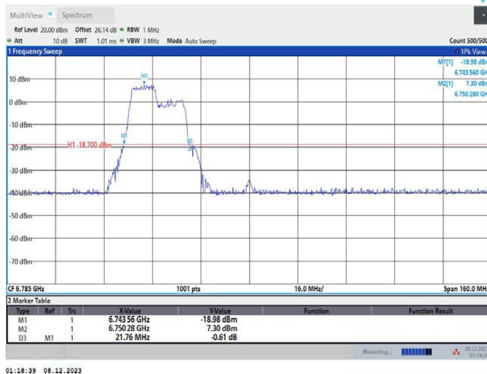
11AX80MIMO_Ant2_6785_242Tone_RU61
