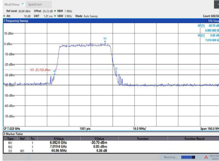
11AX80MIMO_Ant2_7025_26Tone_RU0
