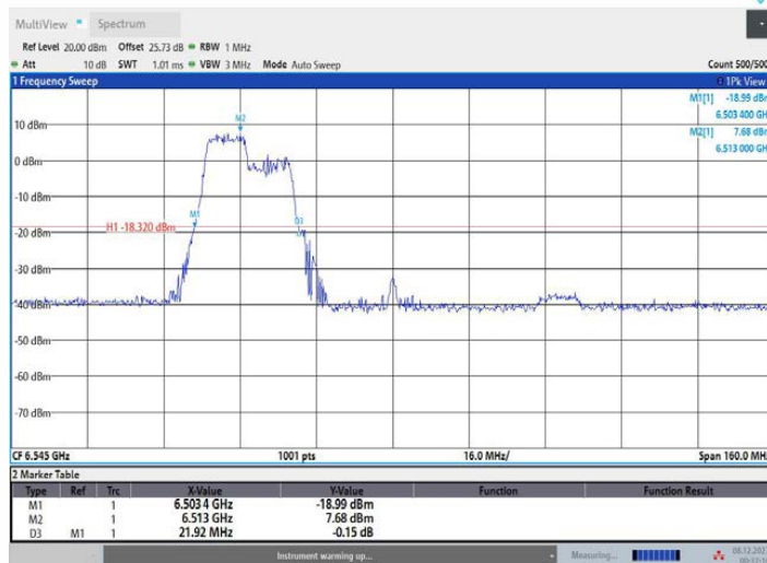
11AX80MIMO_Ant2_6545_242Tone_RU61
