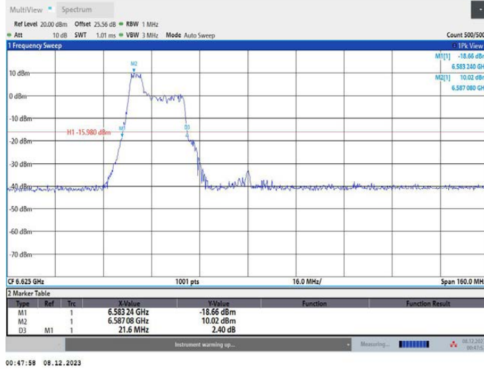
11AX80MIMO_Ant2_6625_106Tone_RU53
