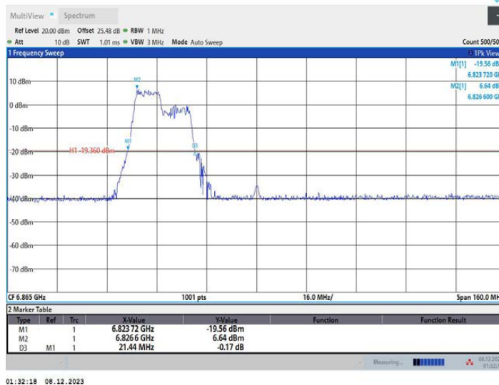
11AX80MIMO_Ant2_6865_242Tone_RU61
