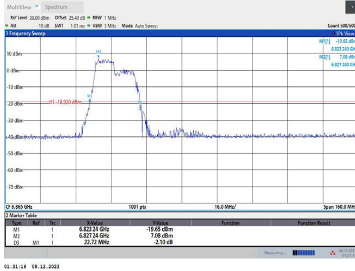
11AX80MIMO_Ant1_6865_242Tone_RU61
