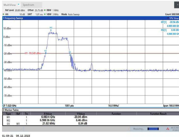
11AX80MIMO_Ant2_7025_242Tone_RU61
