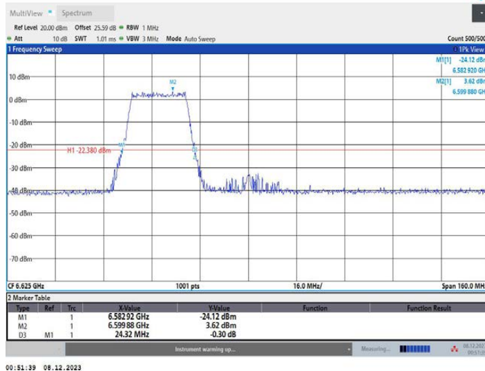
11AX80MIMO_Ant1_6625_484Tone_RU65
