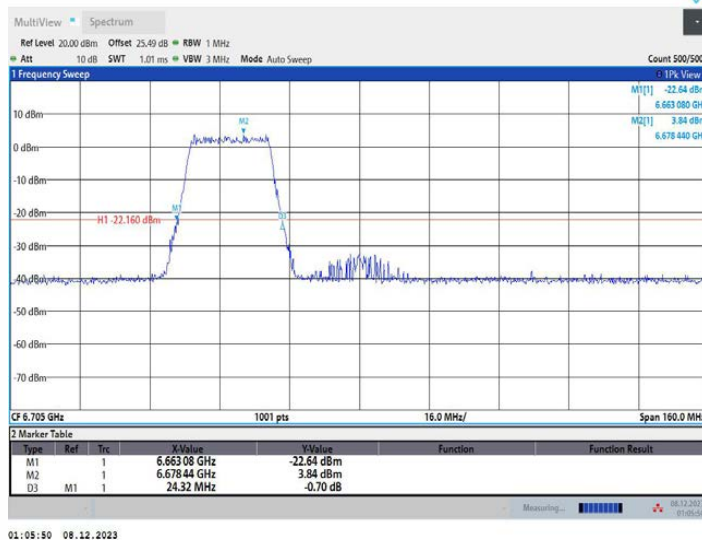
11AX80MIMO_Ant1_6705_484Tone_RU65
