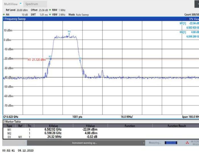
11AX80MIMO_Ant2_6625_484Tone_RU65
