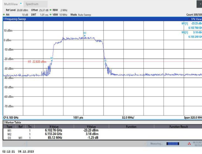
11AX160MIMO_Ant2_6185_996Tone_RU67
