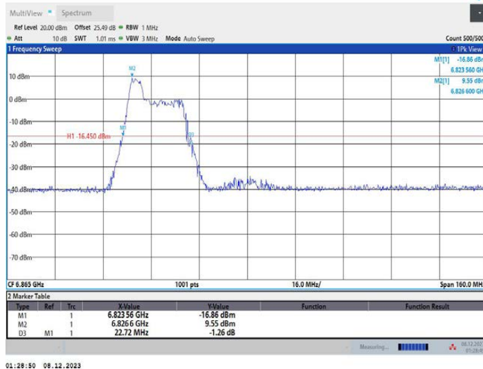
11AX80MIMO_Ant1_6865_106Tone_RU53
