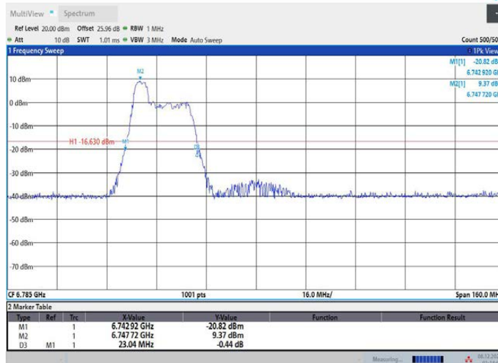
11AX80MIMO_Ant1_6785_106Tone_RU53
