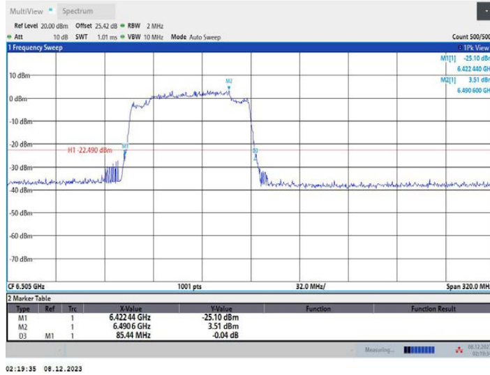
11AX160MIMO_Ant2_6505_996Tone_RU67
