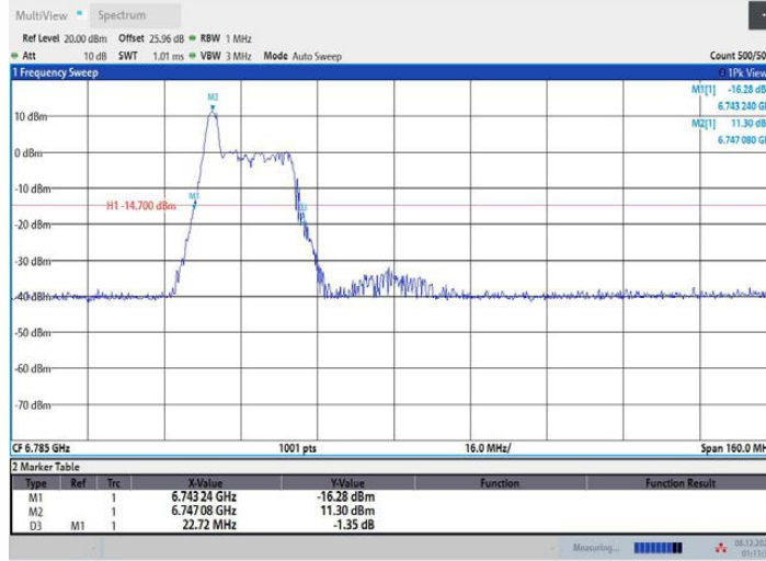
11AX80MIMO_Ant1_6785_52Tone_RU37
