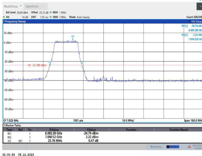
11AX80MIMO_Ant1_7025_484Tone_RU65
