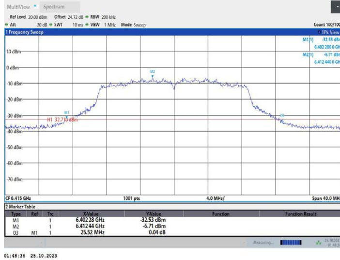
11N20MIMO_Ant2_6415
