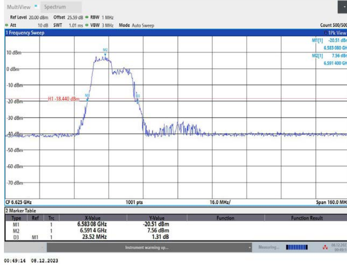
11AX80MIMO_Ant1_6625_242Tone_RU61
