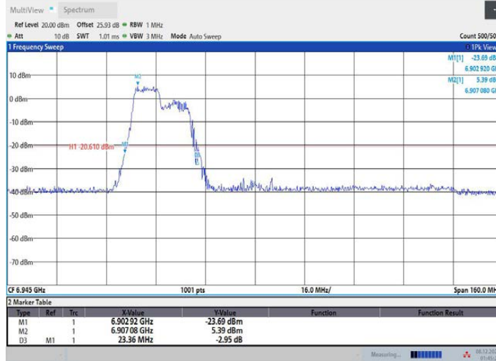
11AX80MIMO_Ant1_6945_242Tone_RU61
