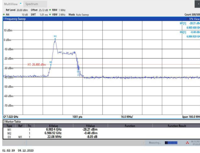
11AX80MIMO_Ant1_7025_52Tone_RU37
