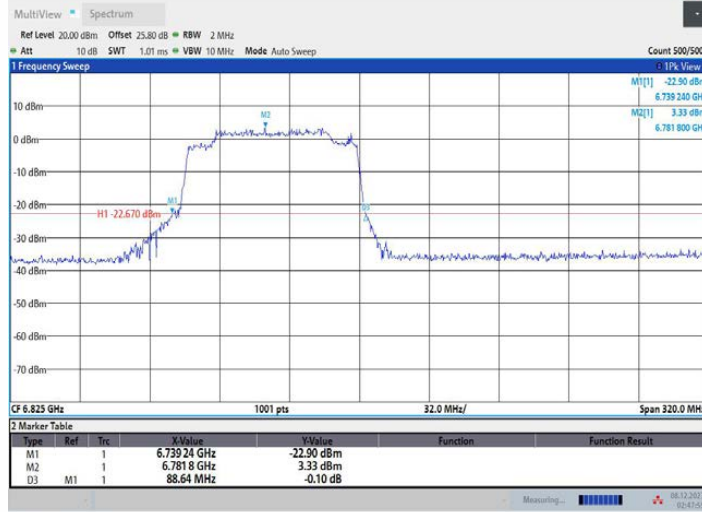
11AX160MIMO_Ant2_6825_996Tone_RU67
