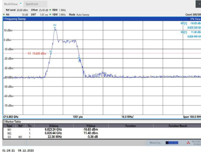
11AX80MIMO_Ant1_6865_52Tone_RU37
