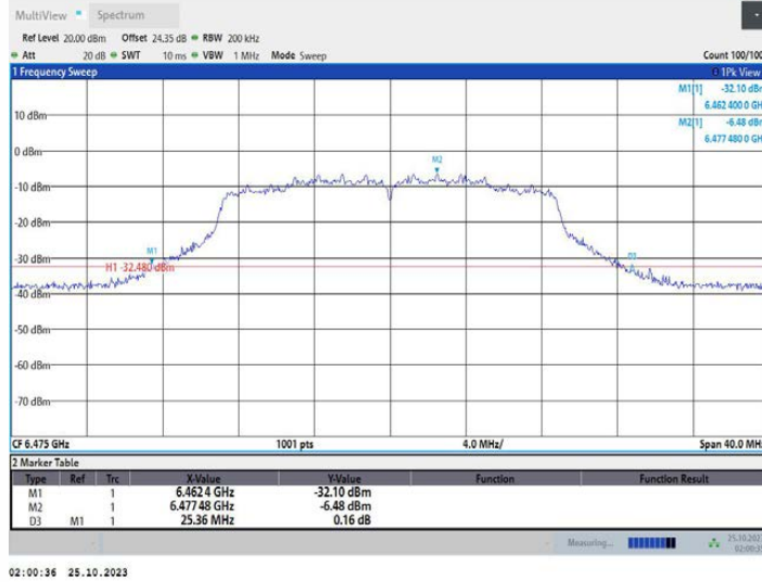
11N20MIMO_Ant2_6475
