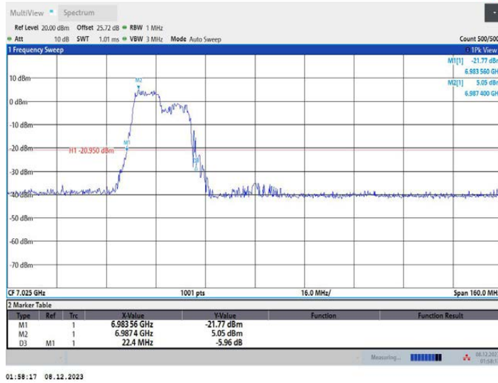
11AX80MIMO_Ant1_7025_242Tone_RU61
