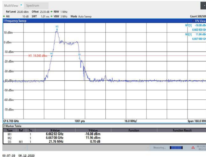
11AX80MIMO_Ant2_6705_52Tone_RU37
