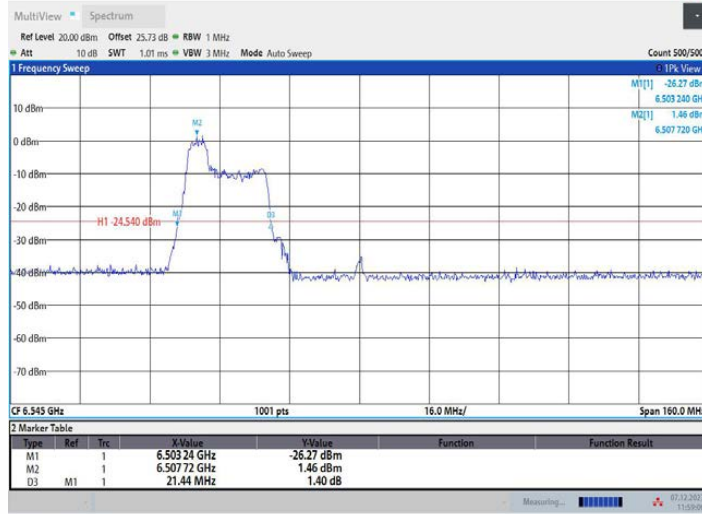
11AX80MIMO_Ant2_6545_106Tone_RU53
