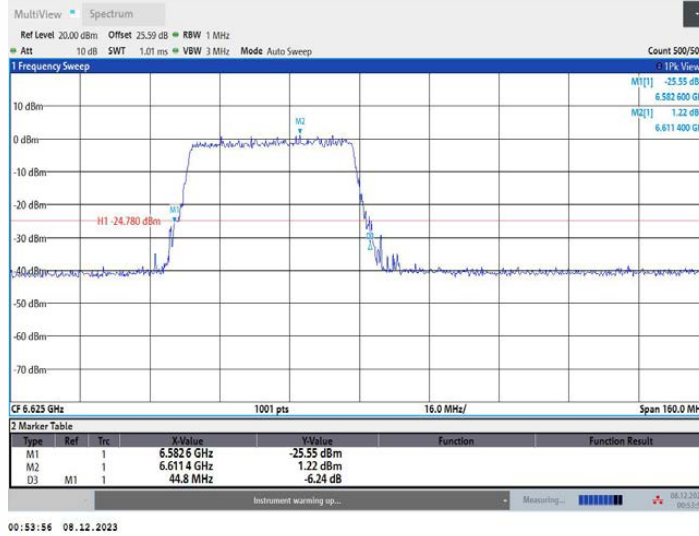
11AX80MIMO_Ant2_6625_26Tone_RU0
