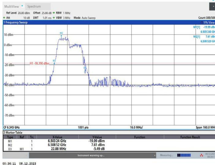
11AX80MIMO_Ant1_6545_242Tone_RU61
