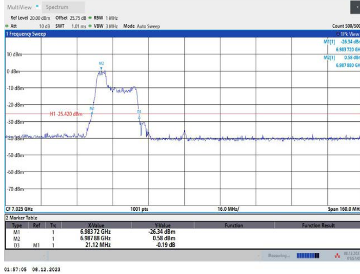
11AX80MIMO_Ant2_7025_106Tone_RU53
