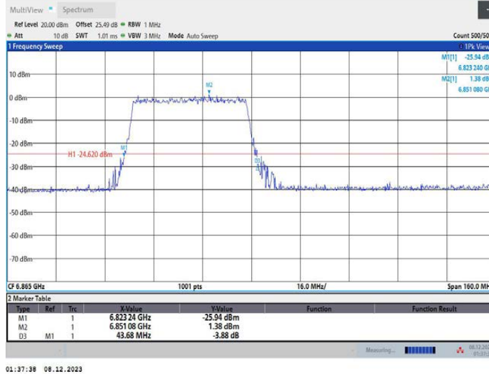
11AX80MIMO_Ant2_6865_26Tone_RU0
