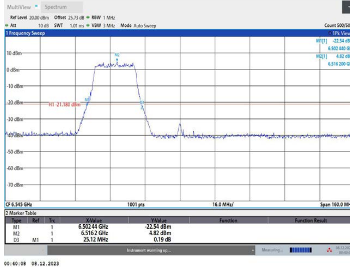
11AX80MIMO_Ant2_6545_484Tone_RU65
