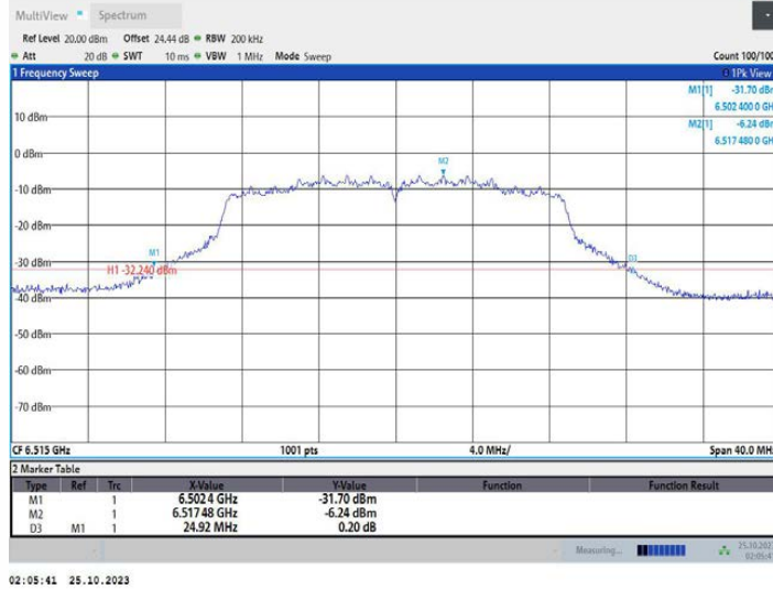
11N20MIMO_Ant2_6515
