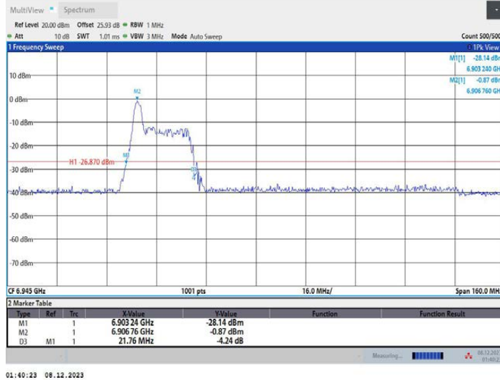
11AX80MIMO_Ant1_6945_52Tone_RU37
