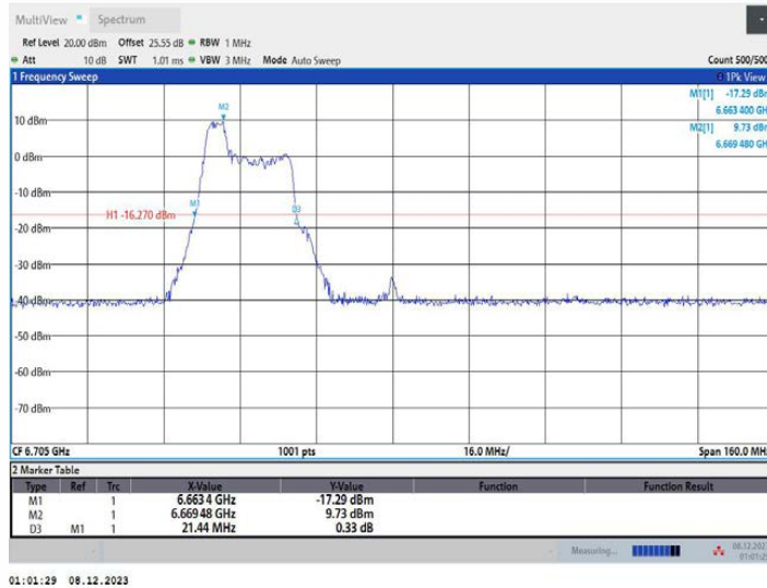
11AX80MIMO_Ant2_6705_106Tone_RU53
