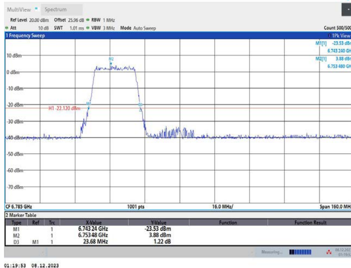
11AX80MIMO_Ant1_6785_484Tone_RU65
