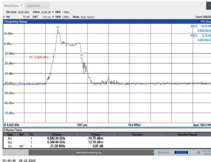
11AX80MIMO_Ant2_6625_52Tone_RU37
