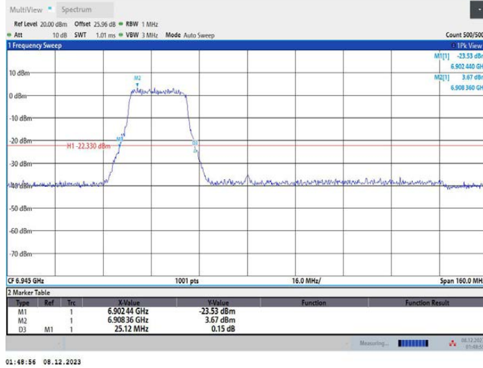
11AX80MIMO_Ant2_6945_484Tone_RU65
