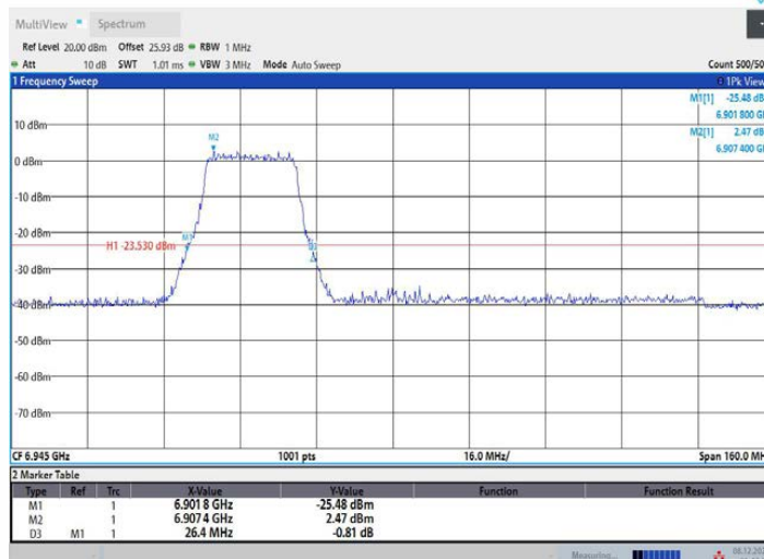
11AX80MIMO_Ant1_6945_484Tone_RU65
