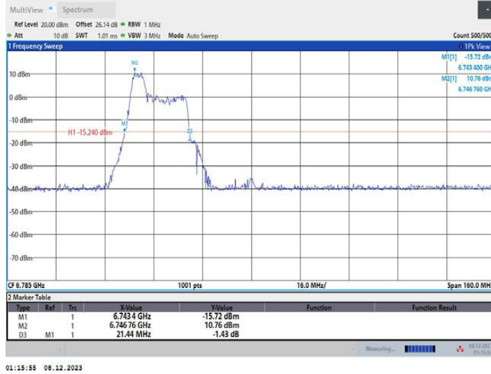
11AX80MIMO_Ant2_6785_106Tone_RU53
