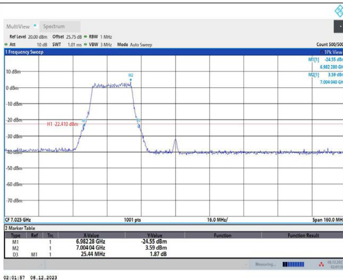
11AX80MIMO_Ant2_7025_484Tone_RU65
