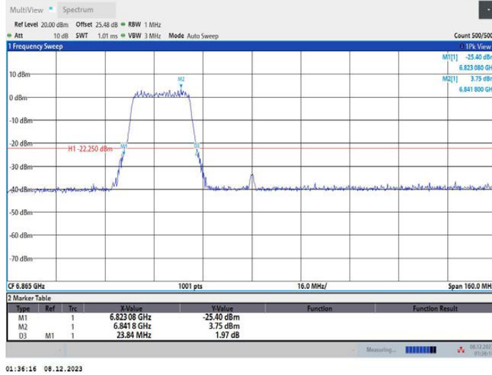
11AX80MIMO_Ant2_6865_484Tone_RU65
