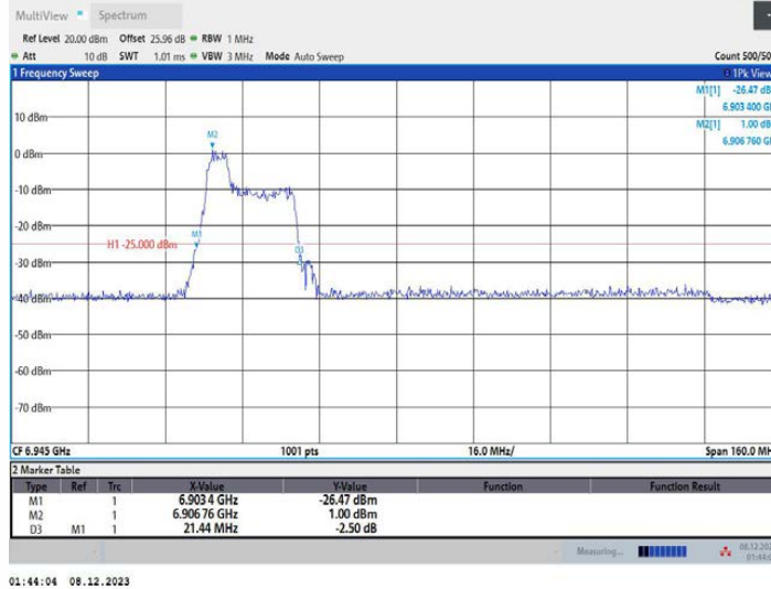
11AX80MIMO_Ant2_6945_106Tone_RU53
