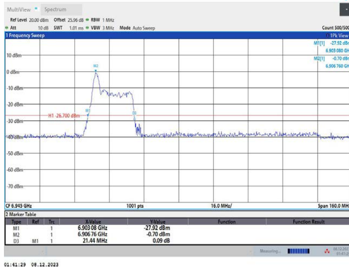
11AX80MIMO_Ant2_6945_52Tone_RU37
