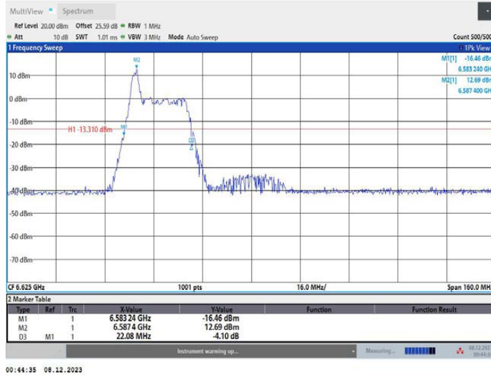
11AX80MIMO_Ant1_6625_52Tone_RU37
