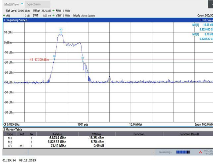
11AX80MIMO_Ant2_6865_106Tone_RU53
