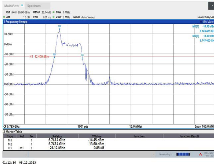
11AX80MIMO_Ant2_6785_52Tone_RU37
