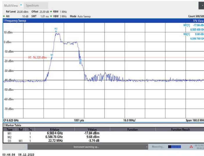
11AX80MIMO_Ant1_6625_106Tone_RU53
