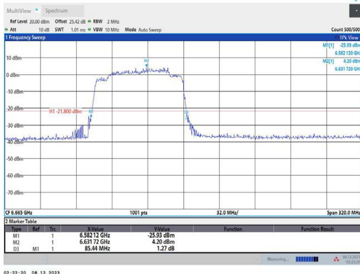
11AX160MIMO_Ant2_6665_996Tone_RU67
