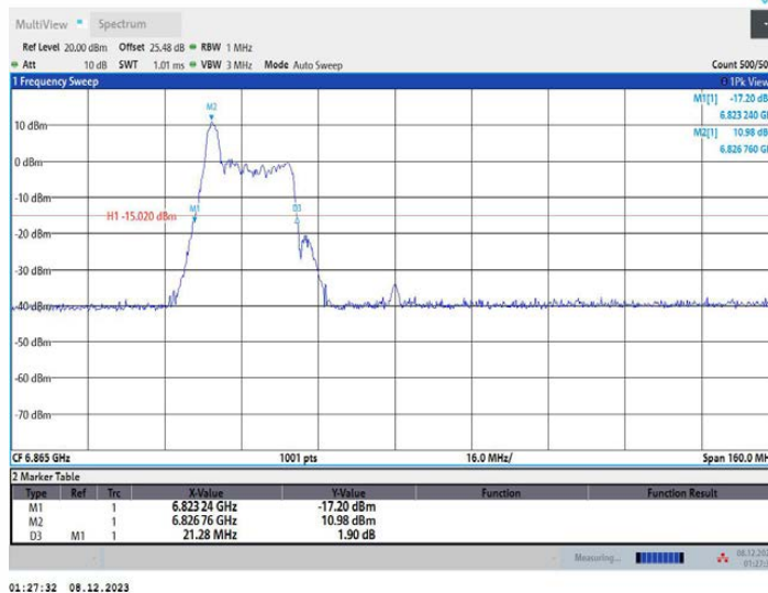
11AX80MIMO_Ant2_6865_52Tone_RU37
