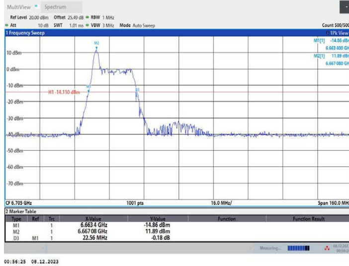
11AX80MIMO_Ant1_6705_52Tone_RU37
