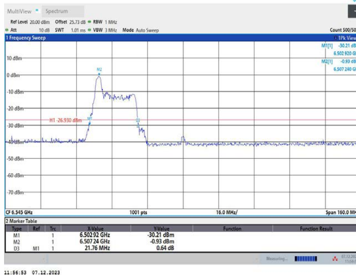
11AX80MIMO_Ant2_6545_52Tone_RU37
