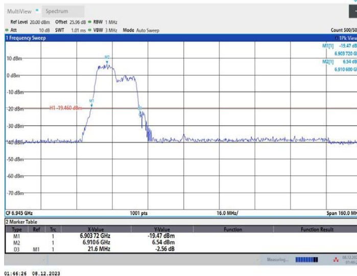
11AX80MIMO_Ant2_6945_242Tone_RU61
