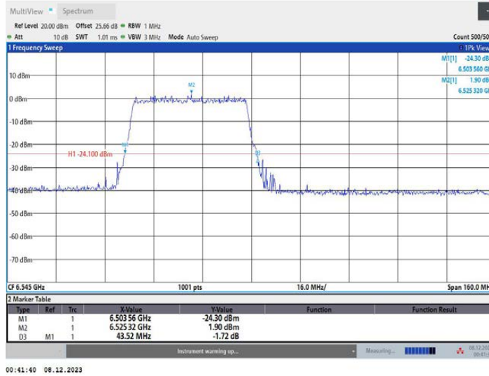
11AX80MIMO_Ant2_6545_26Tone_RU0
