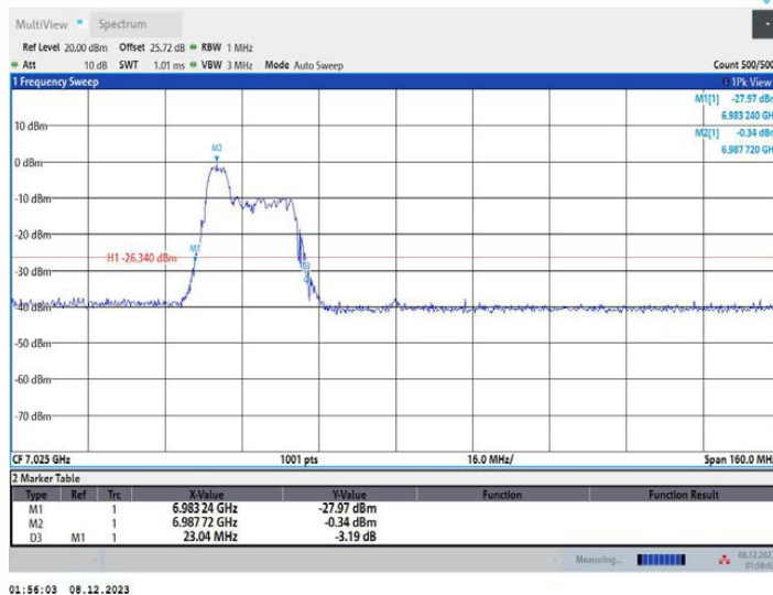
11AX80MIMO_Ant1_7025_106Tone_RU53
