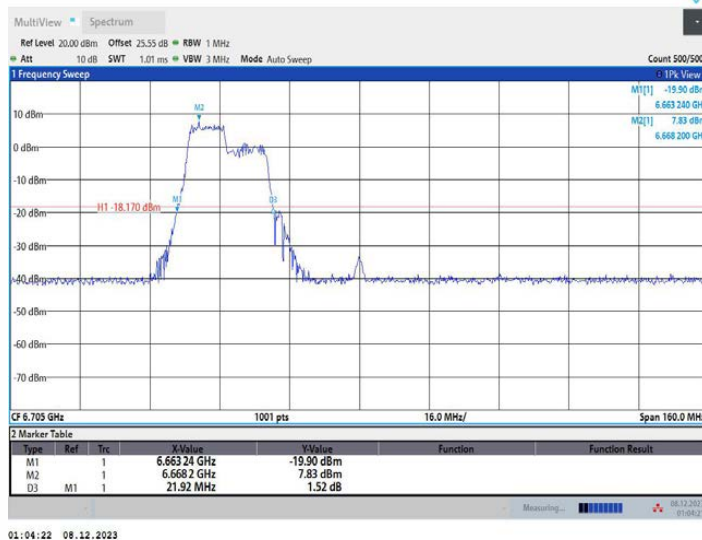
11AX80MIMO_Ant2_6705_242Tone_RU61
