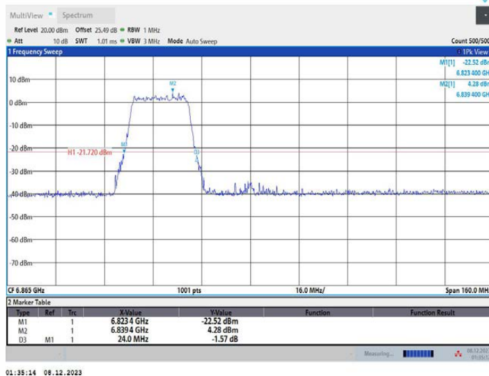
11AX80MIMO_Ant1_6865_484Tone_RU65
