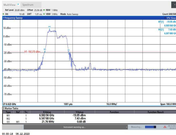
11AX80MIMO_Ant2_6625_242Tone_RU61
