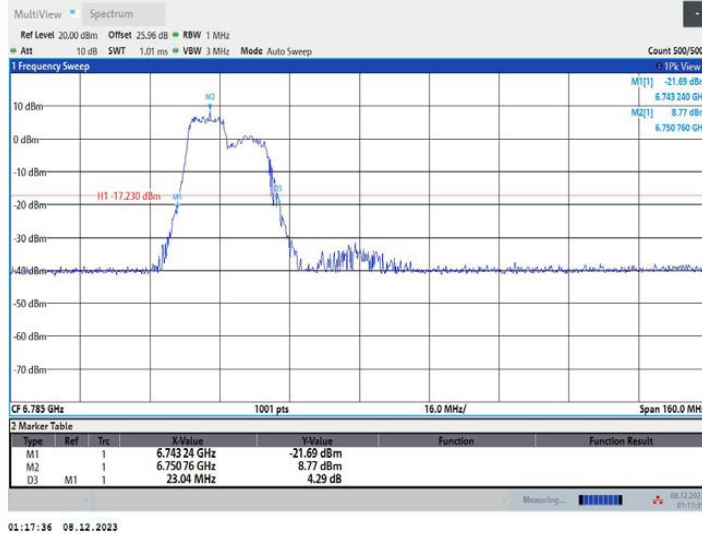
11AX80MIMO_Ant1_6785_242Tone_RU61
