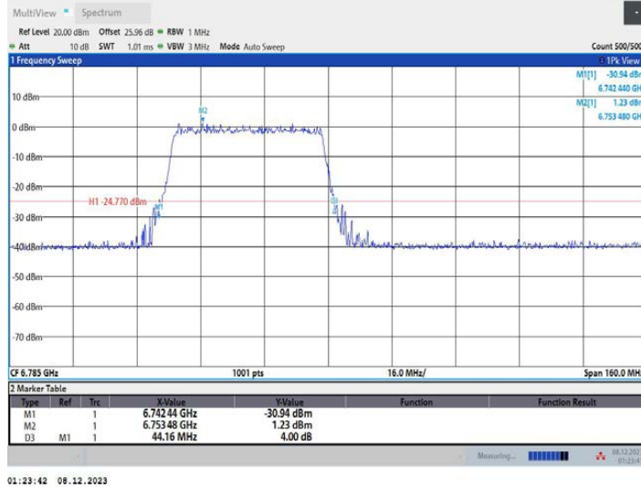
11AX80MIMO_Ant2_6785_26Tone_RU0
