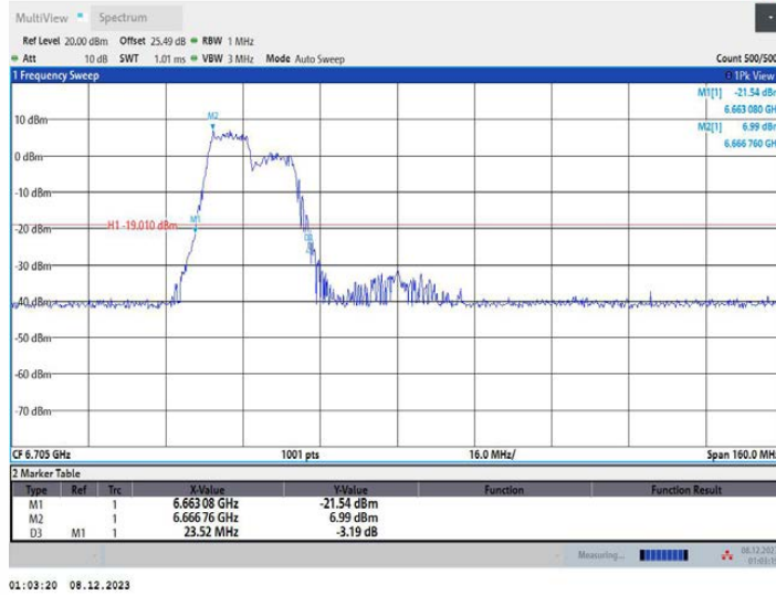
11AX80MIMO_Ant1_6705_242Tone_RU61
