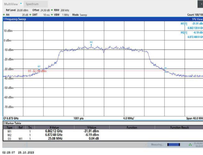
11N20MIMO_Ant2_6875
