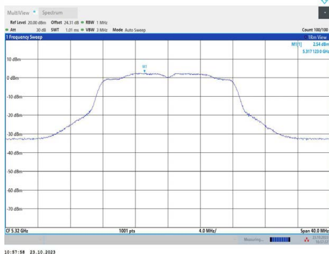
11A_Ant2_5320
