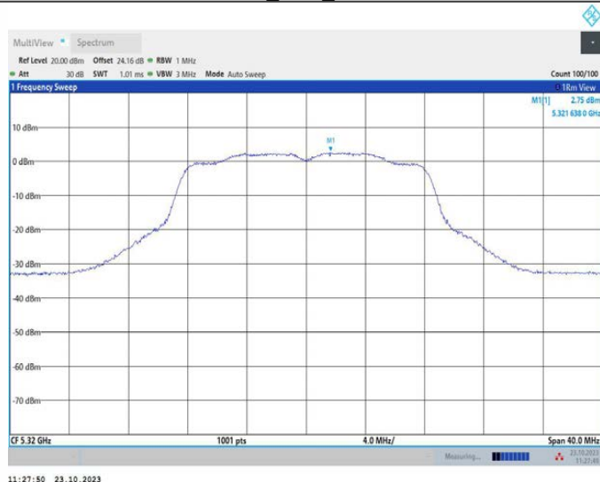
11A_Ant2_5320
