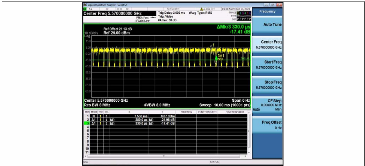
11AC160MIMO_Ant2_5570
