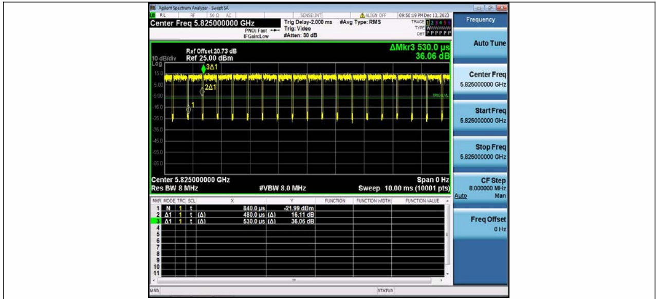
11AX20MIMO Ant2 5825
