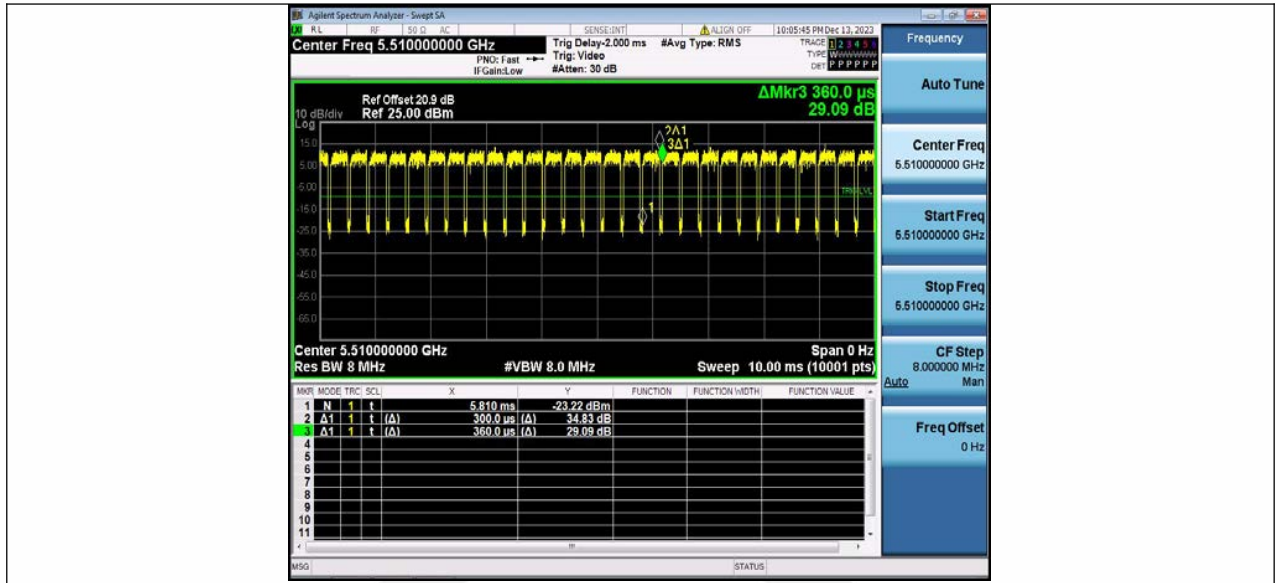
11AX40MIMO Ant2 5510
