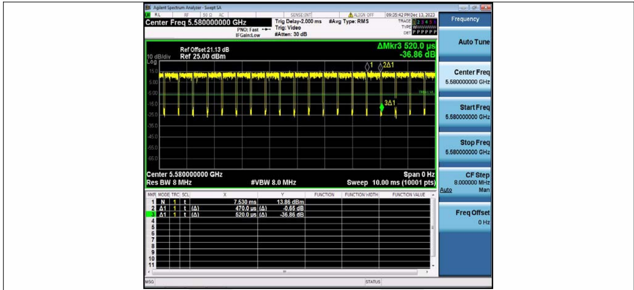
11AX20MIMO Ant2 5580
