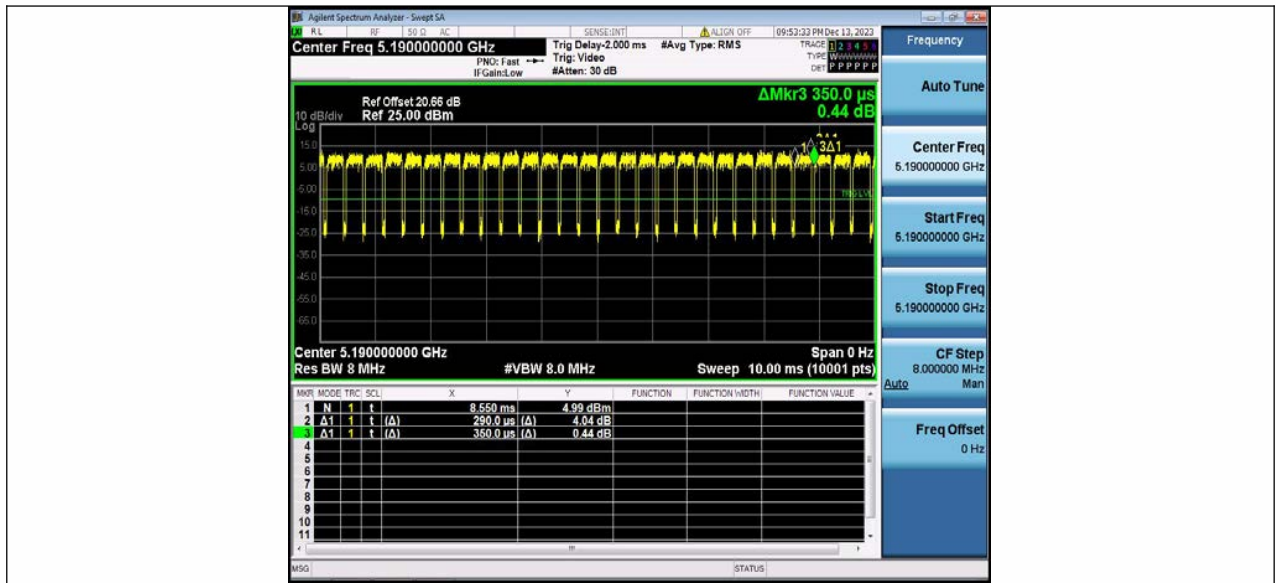
11AX40MIMO Ant2 5190
