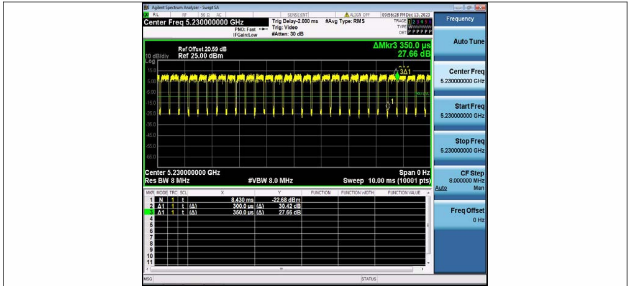
11AX40MIMO Ant2 5230
