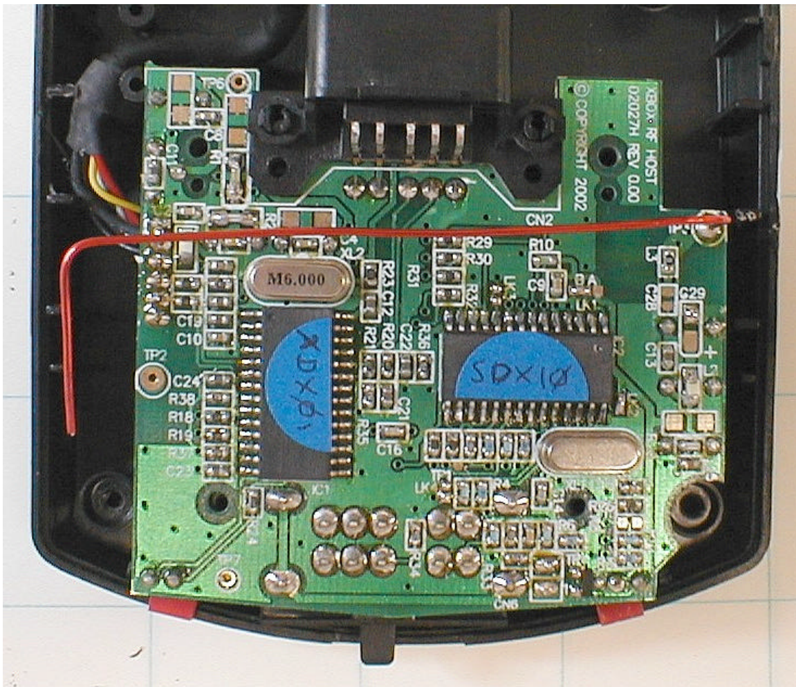
PCB Top
