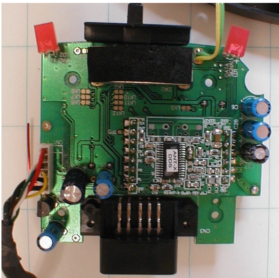
PCB Bottom
