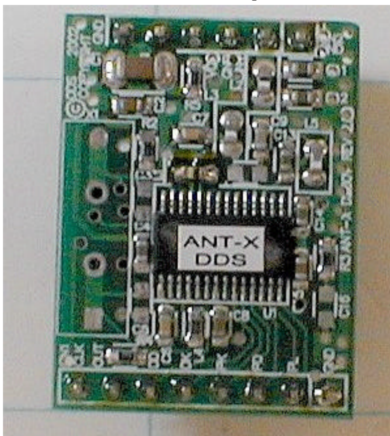
ANT Module Top
