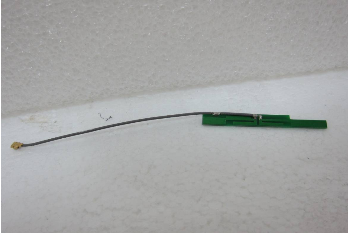
EUT 13 (antenna 5)
