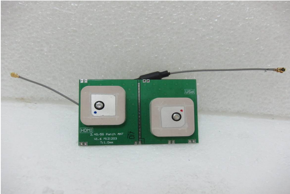
EUT 9 (antenna 3-2)
