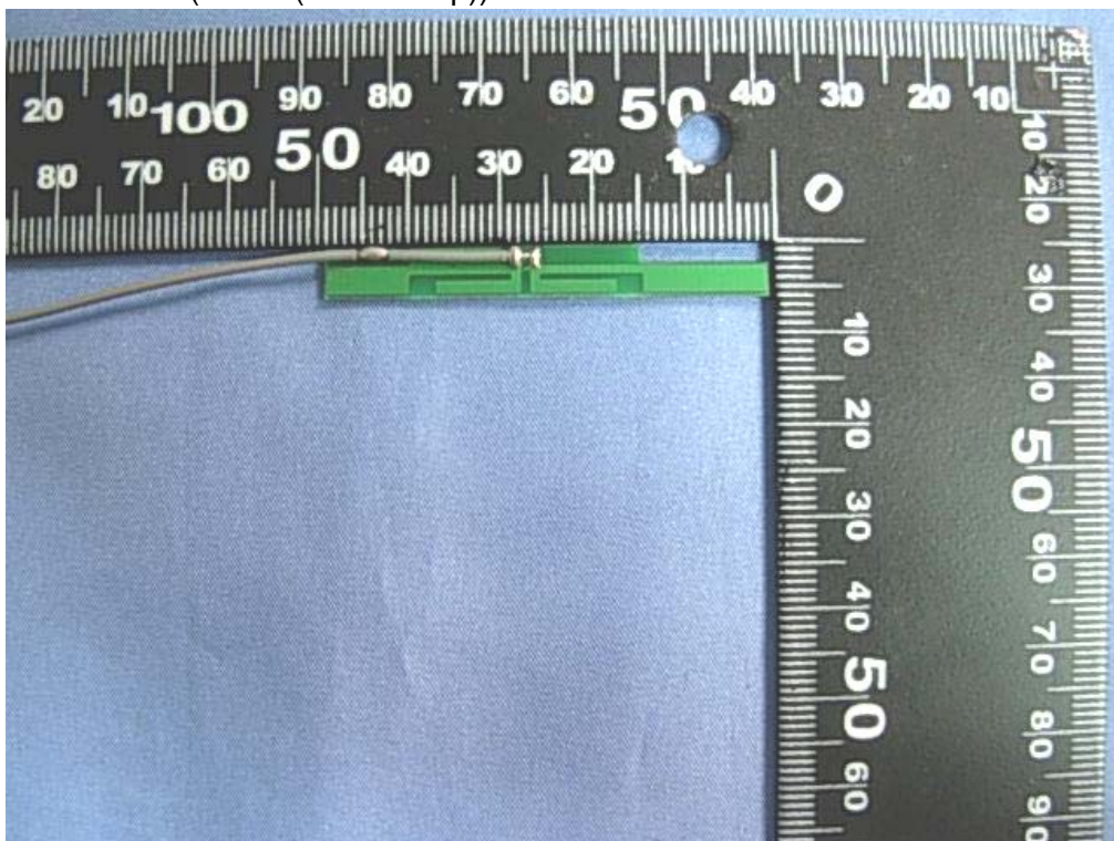
(7) EUT Photo (Ant. 4 (UDMGroup))
