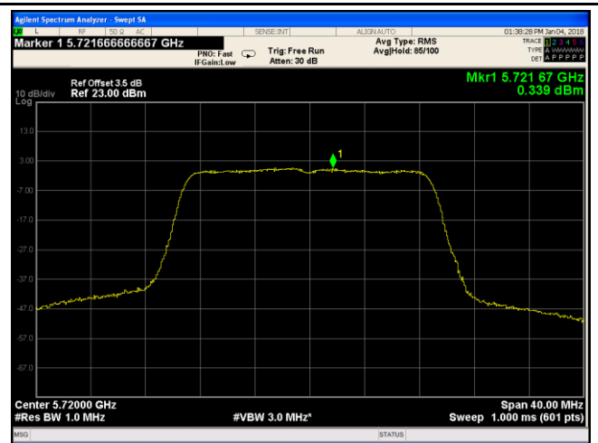
5725-5850MHz PSD - Mid CH 5720
