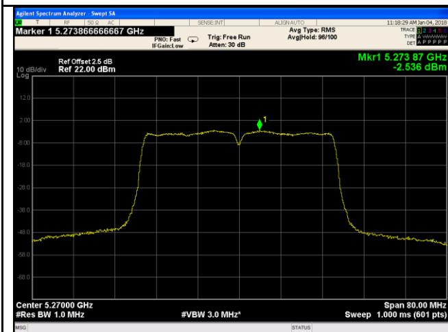
5250-5350MHz PSD - Low CH 5270
