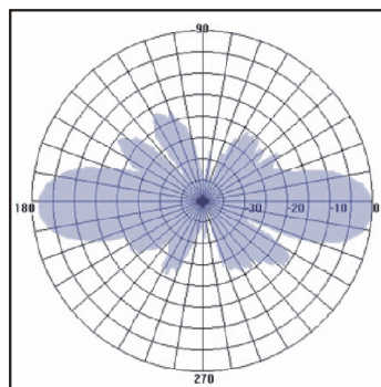
垂直面方向图 Vertical pattern
