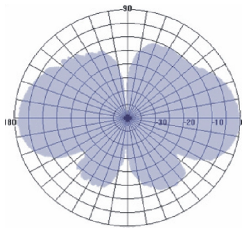
垂直面方向图 Vertical pattern
