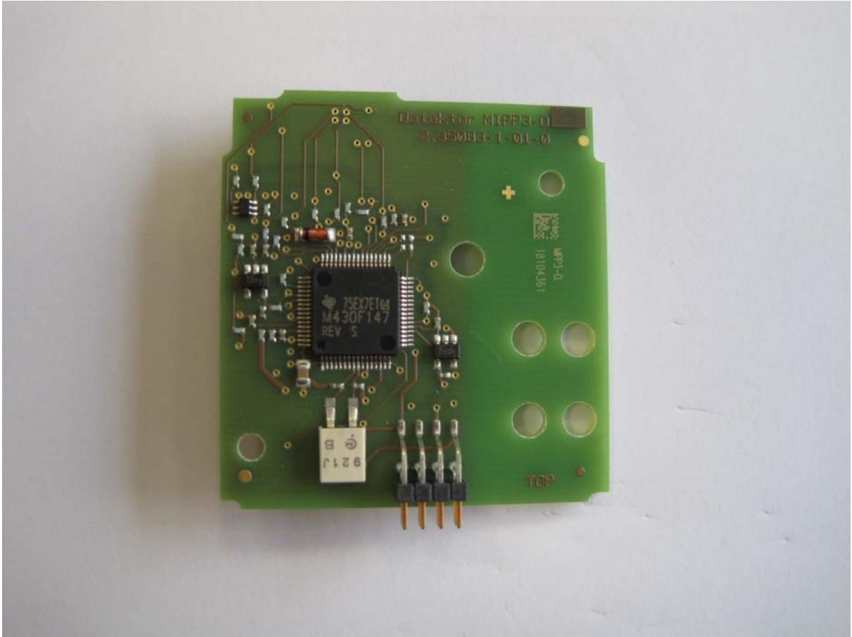
Detector Top
