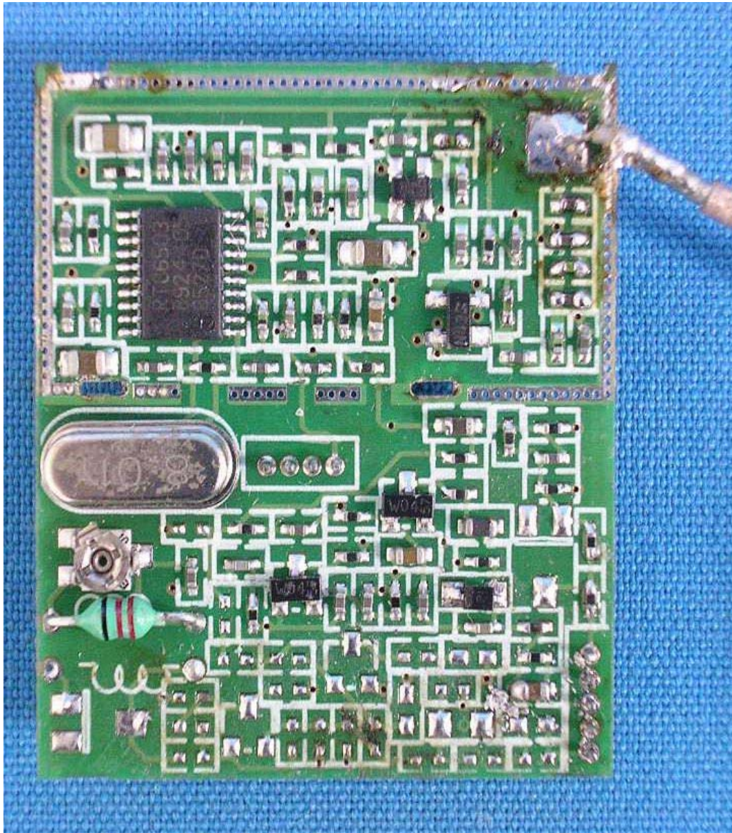
(14) EUT Photo
