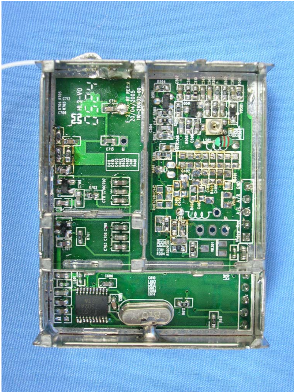
(17) EUT Photo
