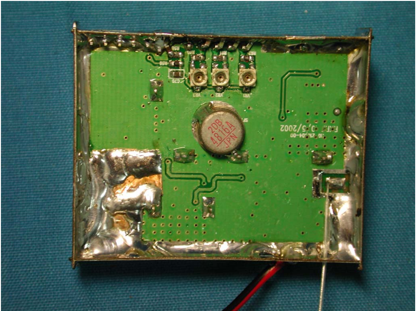
(13) EUT Photo
