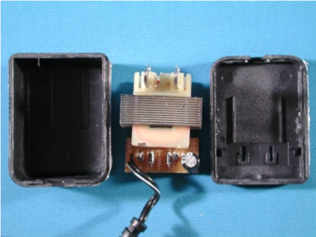
(18) EUT Photo
