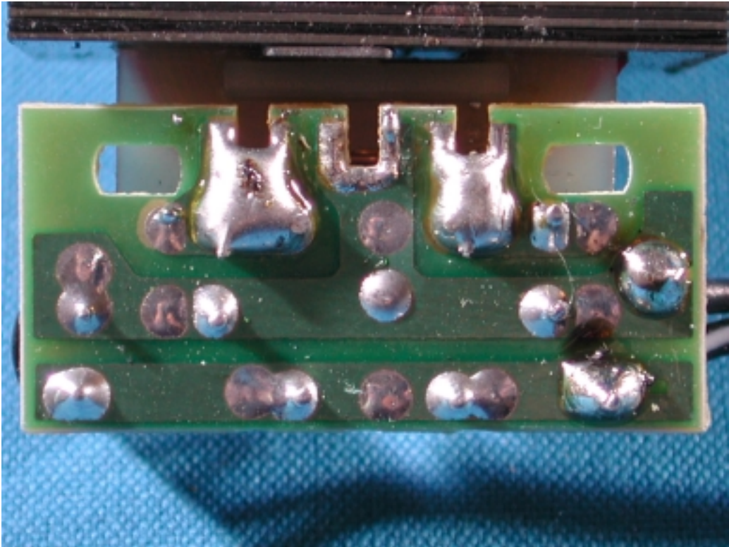
(19) EUT Photo
