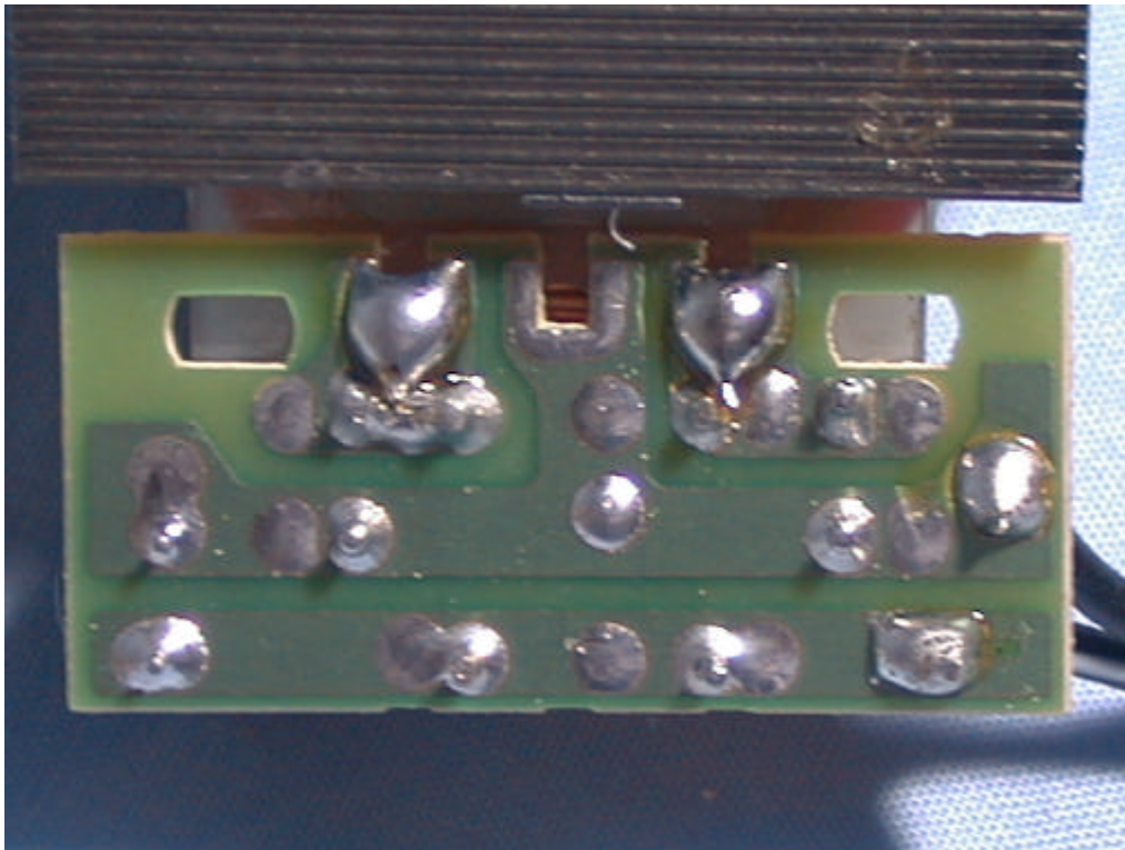
(31) EUT Photo
