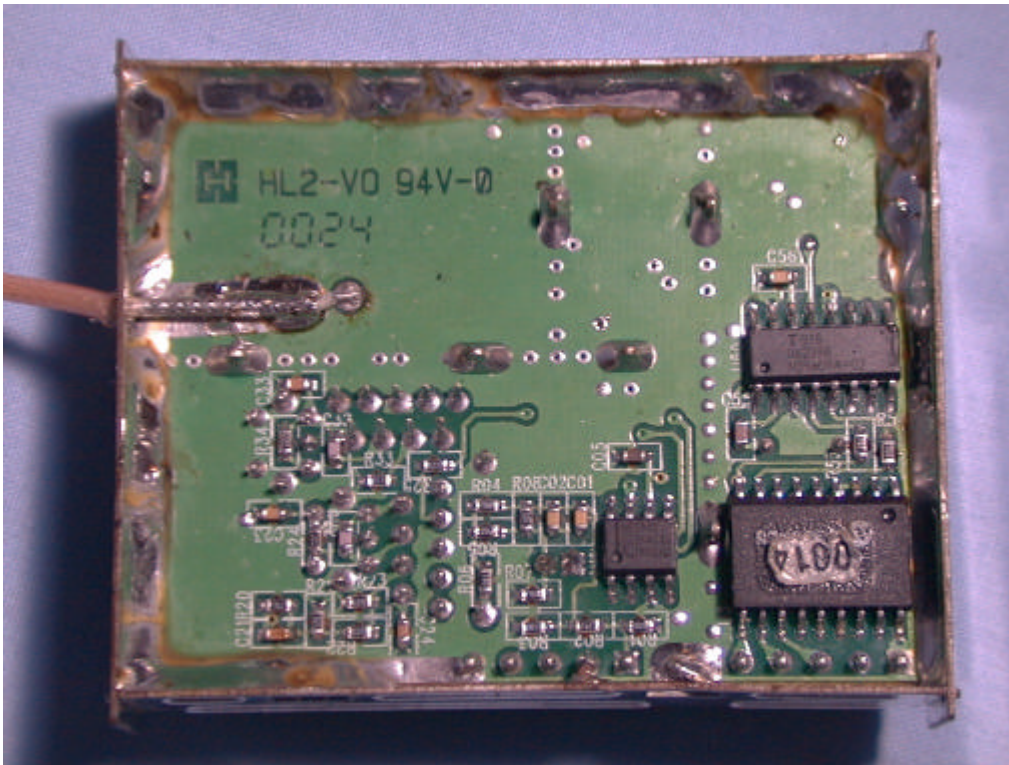
(13) EUT Photo
