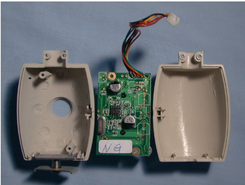
(15) EUT Photo
