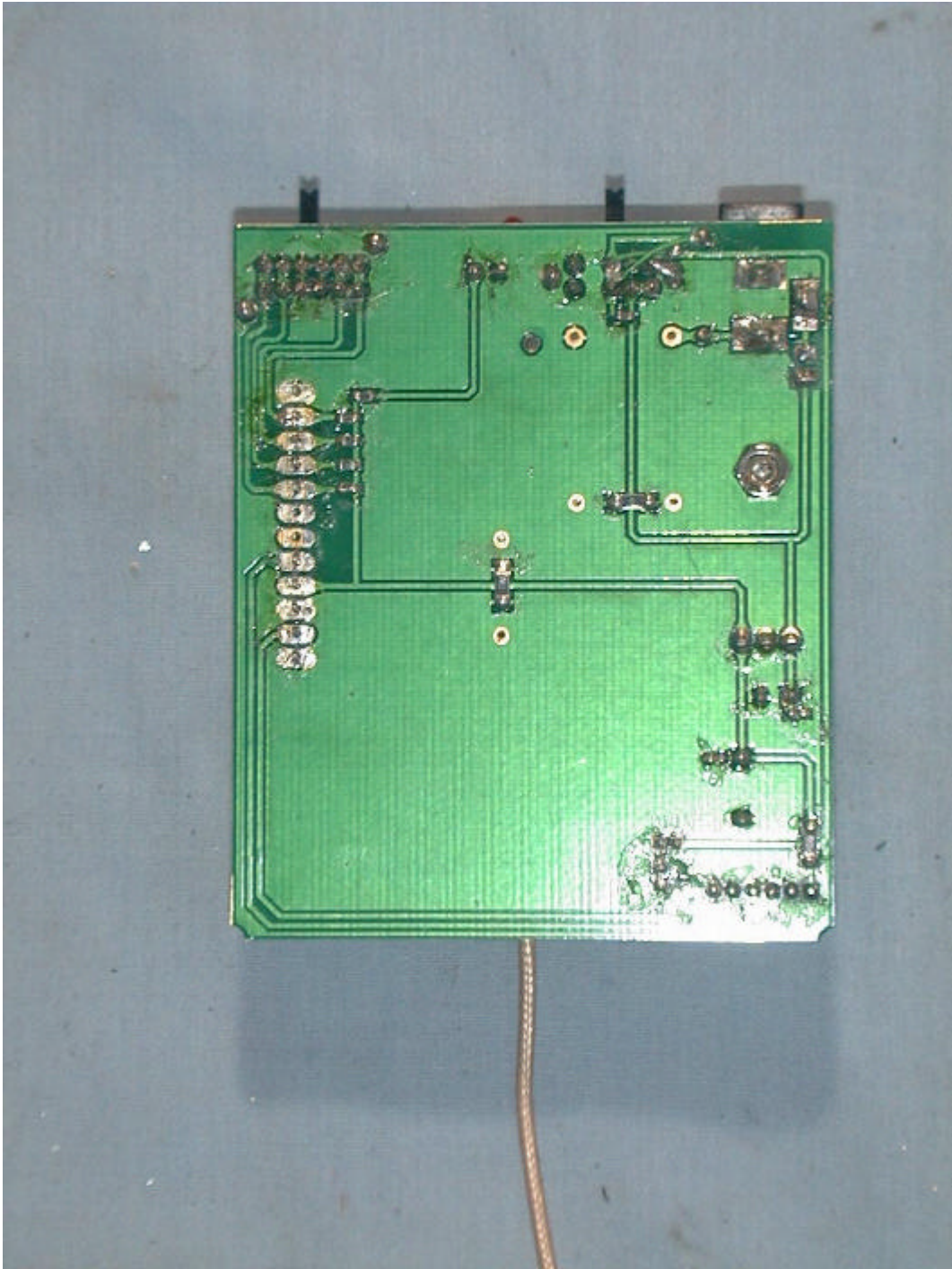
(24) EUT Photo
