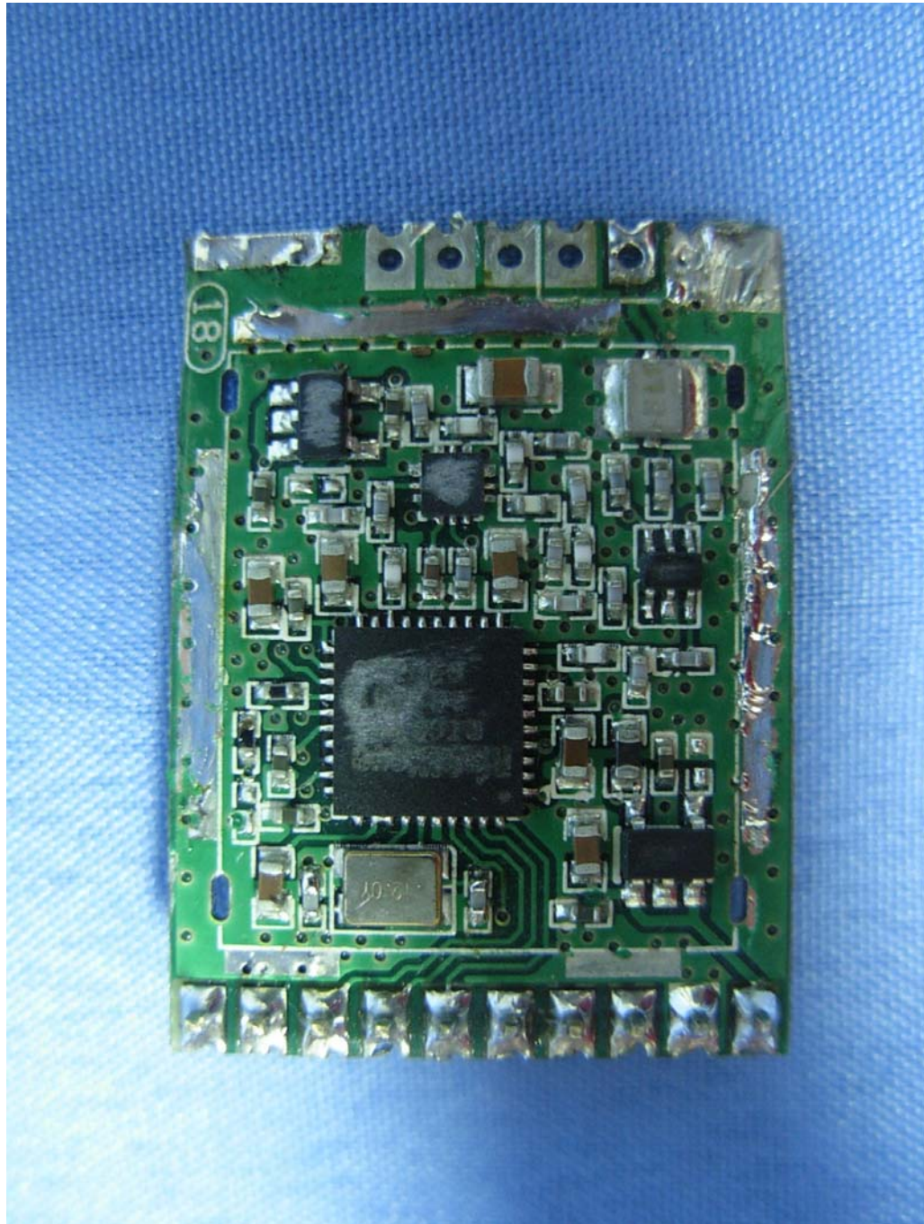
(9) EUT Photo
