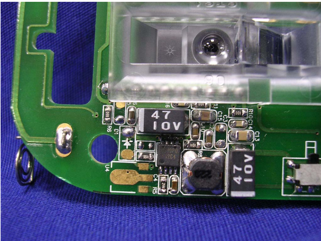
(8) EUT Photo (N747)
