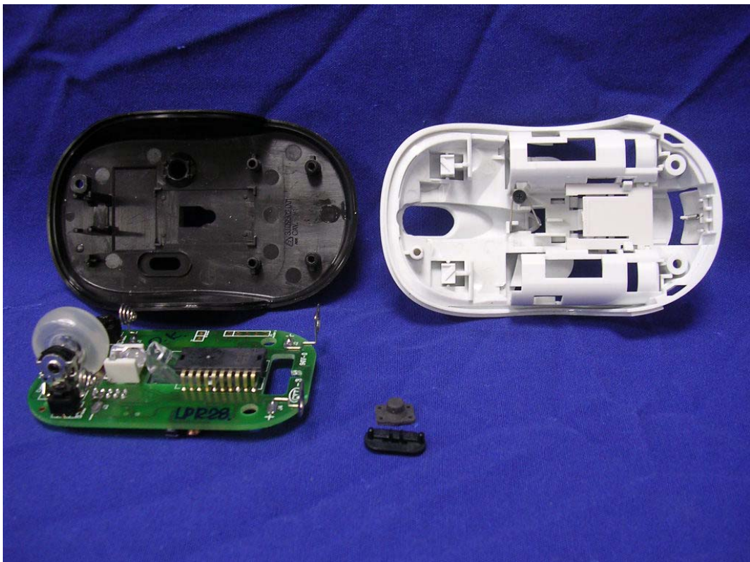
(4) EUT Photo (N747)
