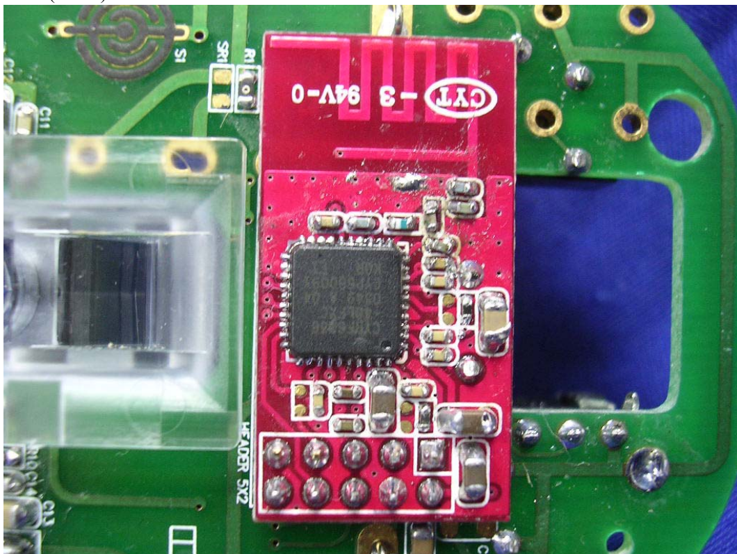
(22) EUT Photo (N745)
