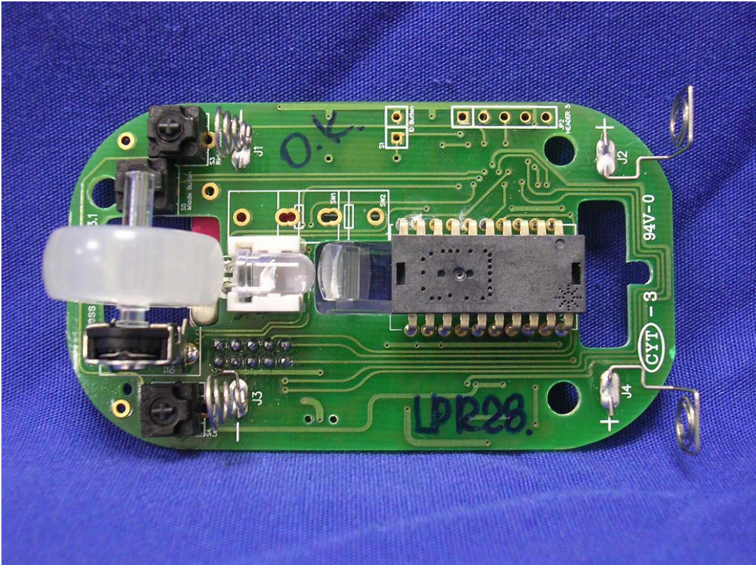
(5) EUT Photo (N747)
