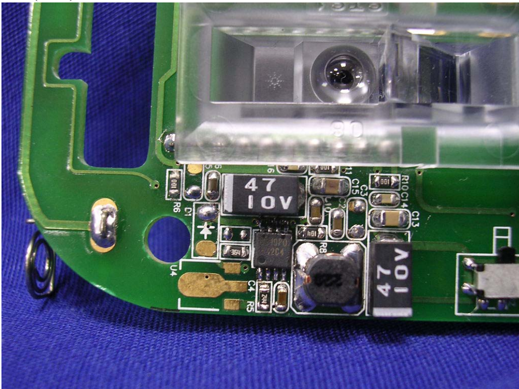
(20) EUT Photo (N745)
