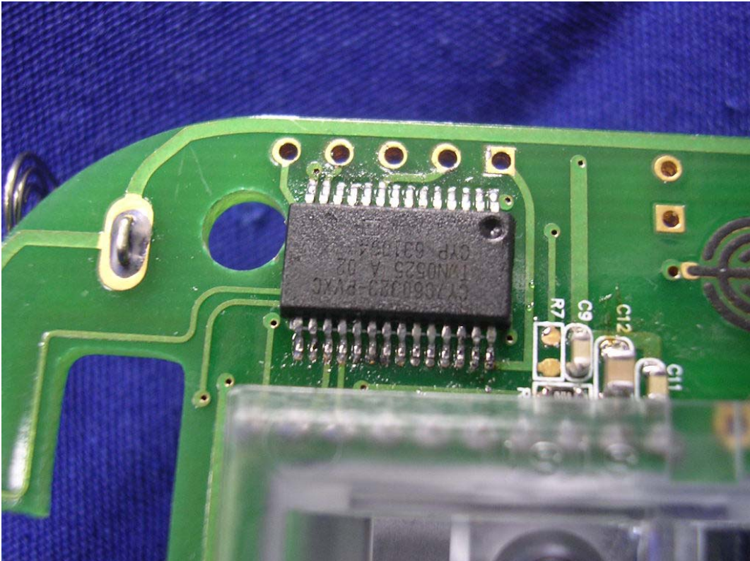
(7) EUT Photo (N747)
