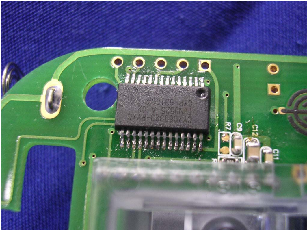
(19) EUT Photo (N745)
