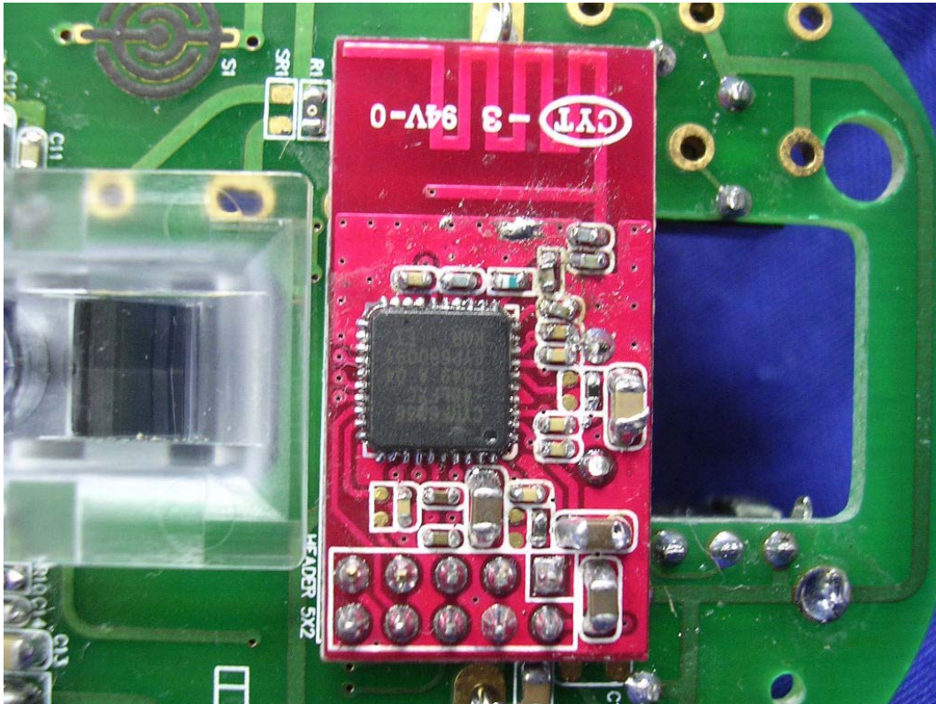
(9) EUT Photo (N747)
