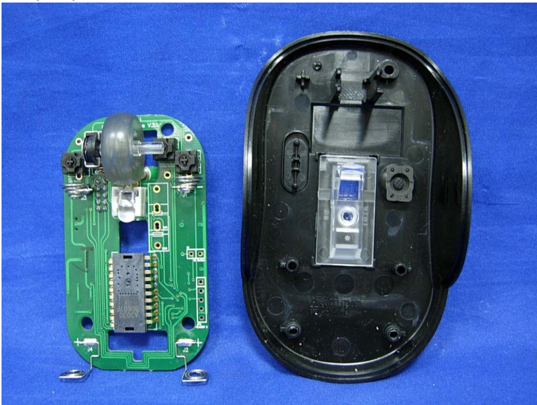
(16) EUT Photo (N745)
