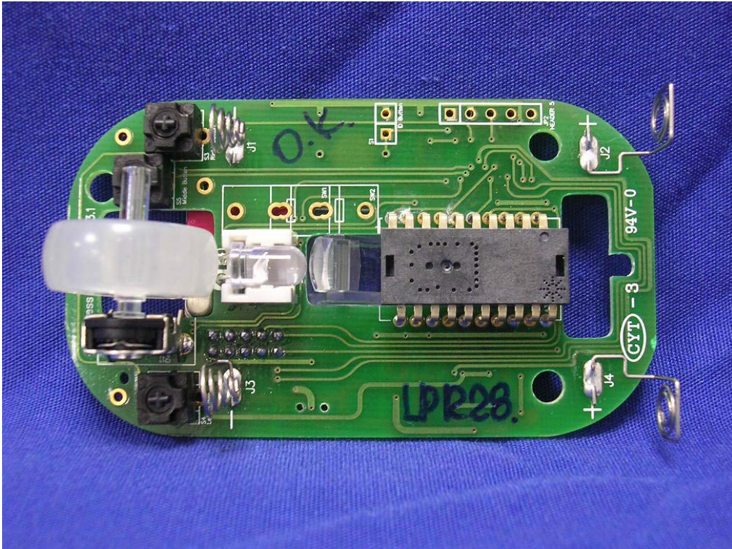
(17) EUT Photo (N745)
