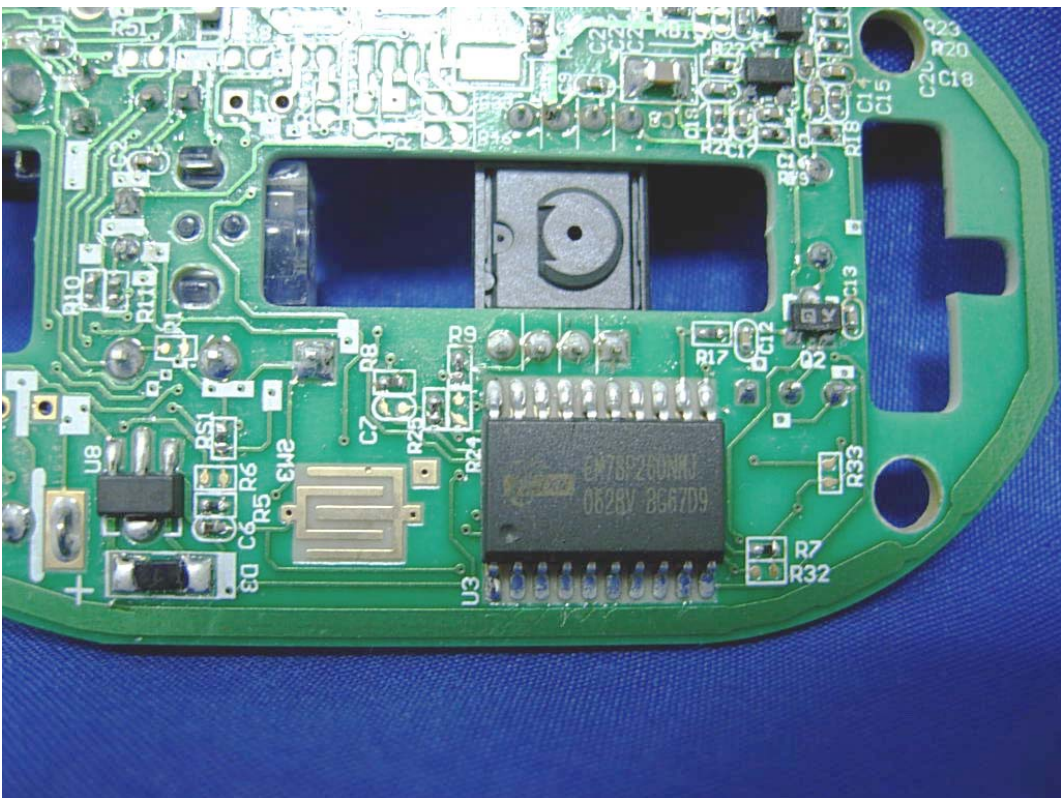
(26) EUT Photo(M/N:M310)
