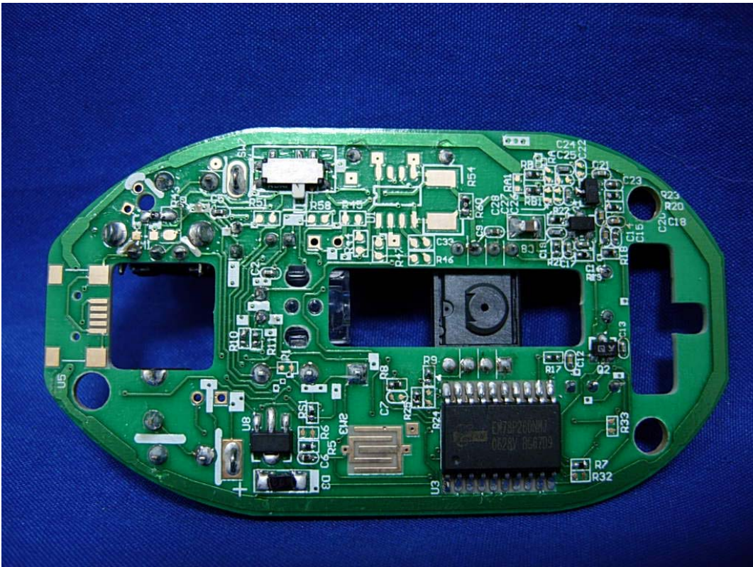
(25) EUT Photo(M/N:M310)
