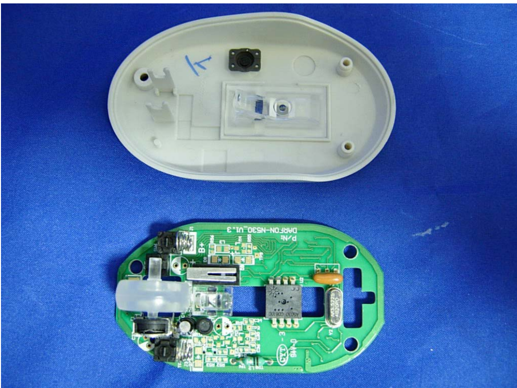
(22) EUT Photo(M/N:M310)
