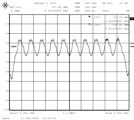
2410-2411MHz
