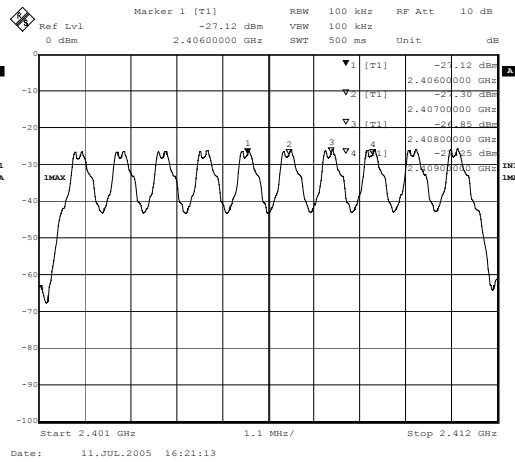
2406-2409MHz
