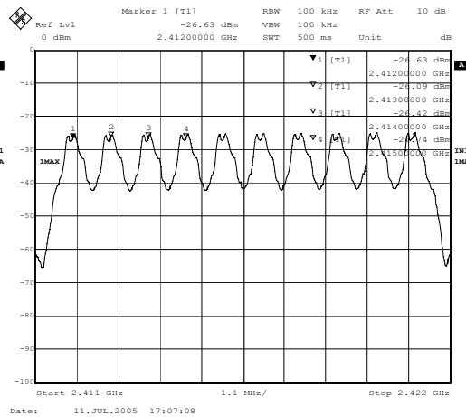
2412-2415MHz
