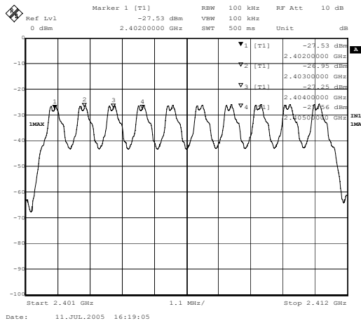
2402-2405MHz
