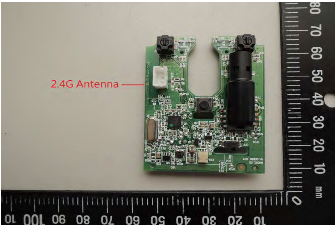
2.4G Antenna
