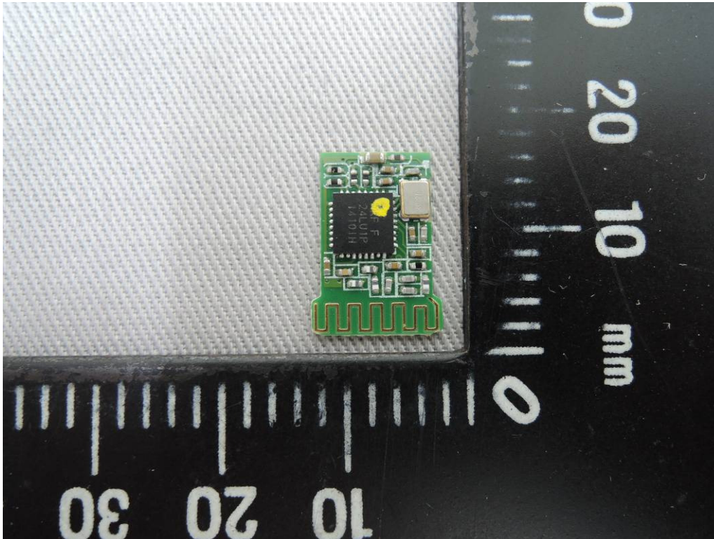
2.4G Antenna
