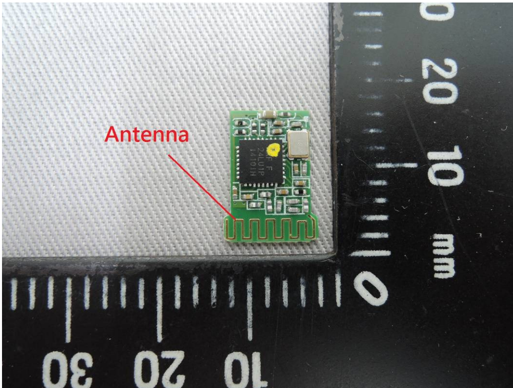
2.4G Antenna
