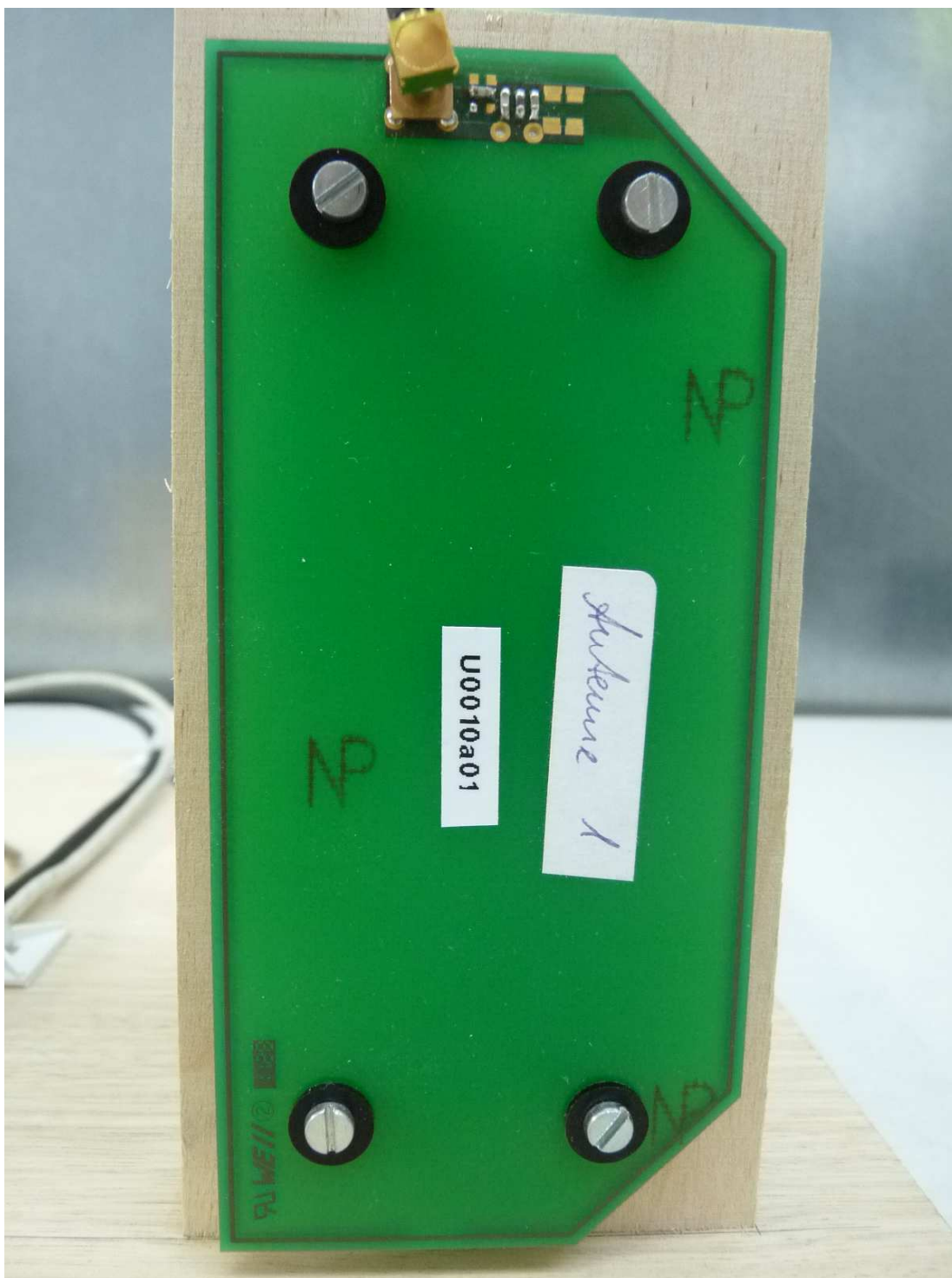
Antenna Validator (0364127)
