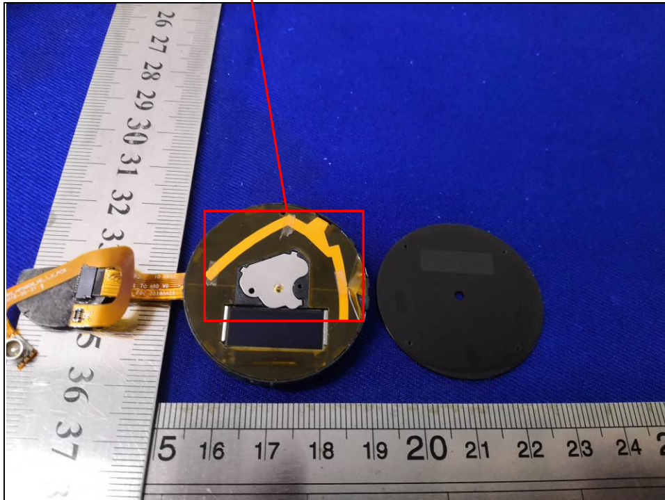
BLE Antenna
