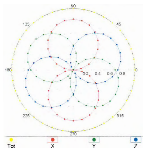
f=1800 MHz,R22
