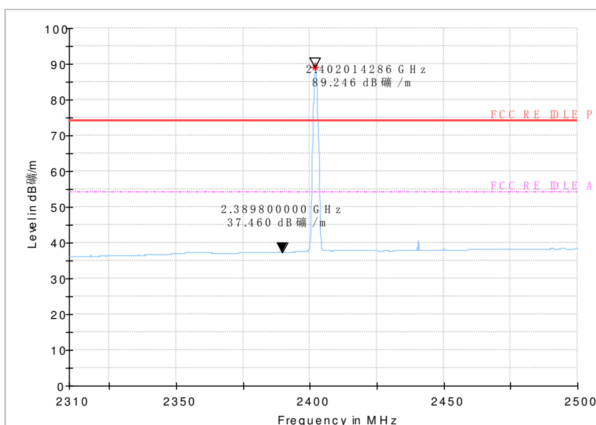
AV detector
