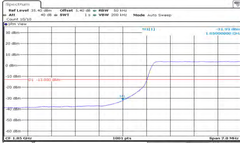
Band2-5MHz-QPSK-18625-25RB#0
