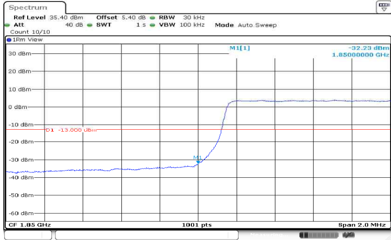
Band2-3MHz-16QAM-18615-15RB#0
