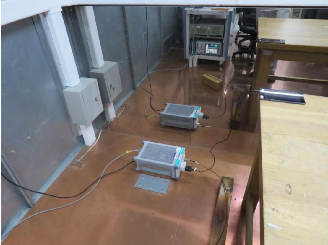
Test Setup photos Lenovo TB-7504X 15B-CE
