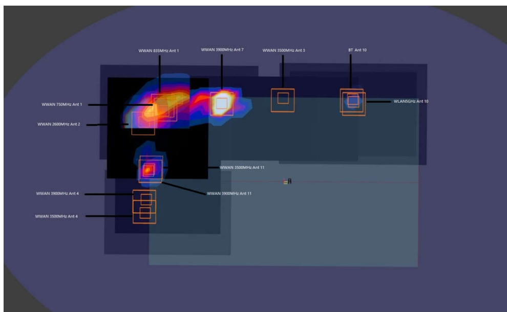
WWAN+5G+BT_Bottom 0mm
