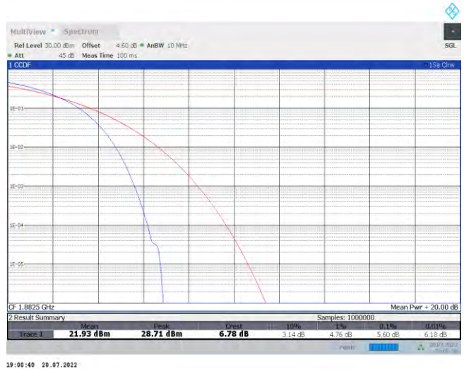
Band25-20MHz-QPSK-26365-100RB#0
