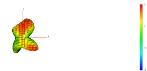
7000MHZ
