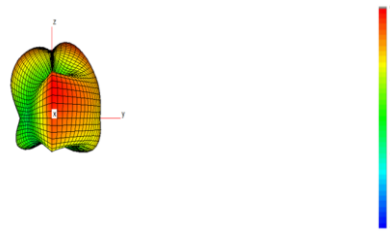
6000MHZ
