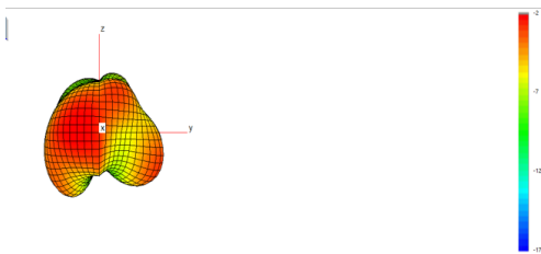
2500MHZ
