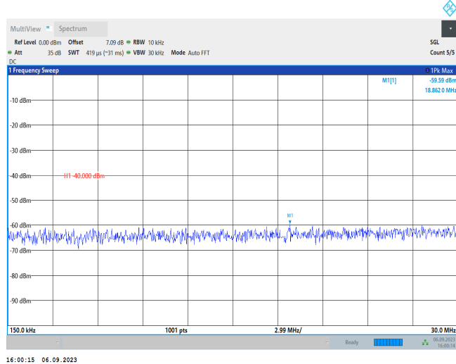
Band30-10MHz-QPSK-27710-1RB#0-Range2:0.15~30MHz
