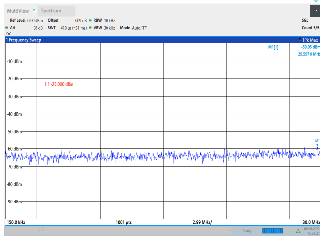
Band14-10MHz-QPSK-23330-1RB#0-Range2:0.15~30MHz
