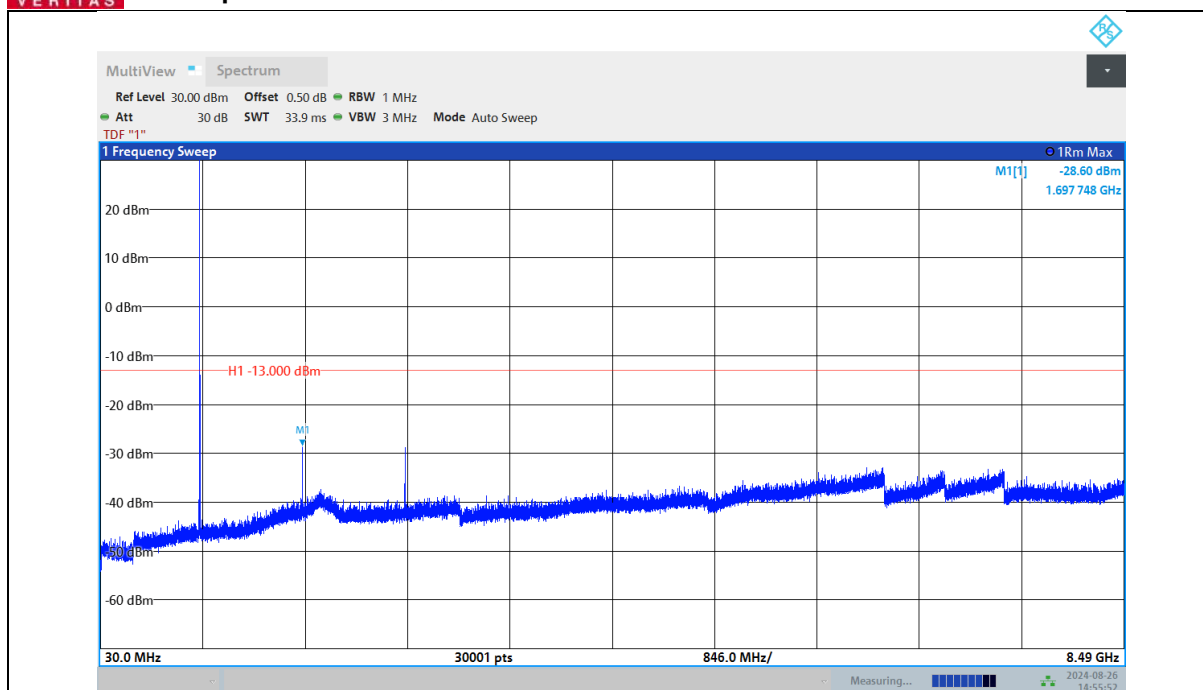
EGPRS850-128-30~8490MHz
