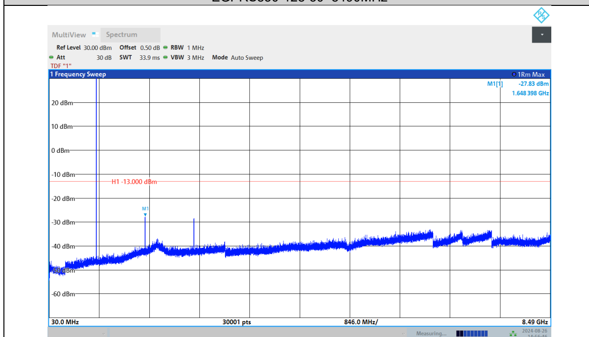
EGPRS850-189-30~8490MHz
