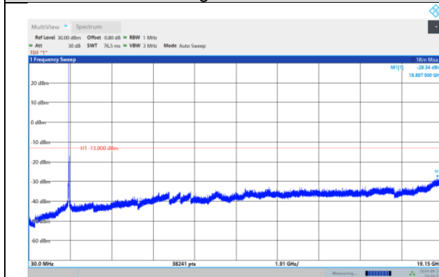
Band25-20MHz-16QAM-26590-1RB#0-
